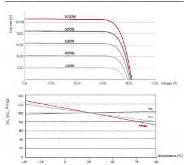
Figura 13. Scheda tecnica modulo fotovoltaico LG325N1C-A5 utilizzato nell’impianto.
