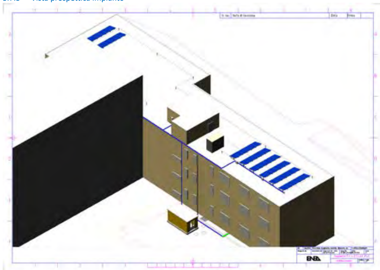
Figura 6. Vista prospettica impianto.
