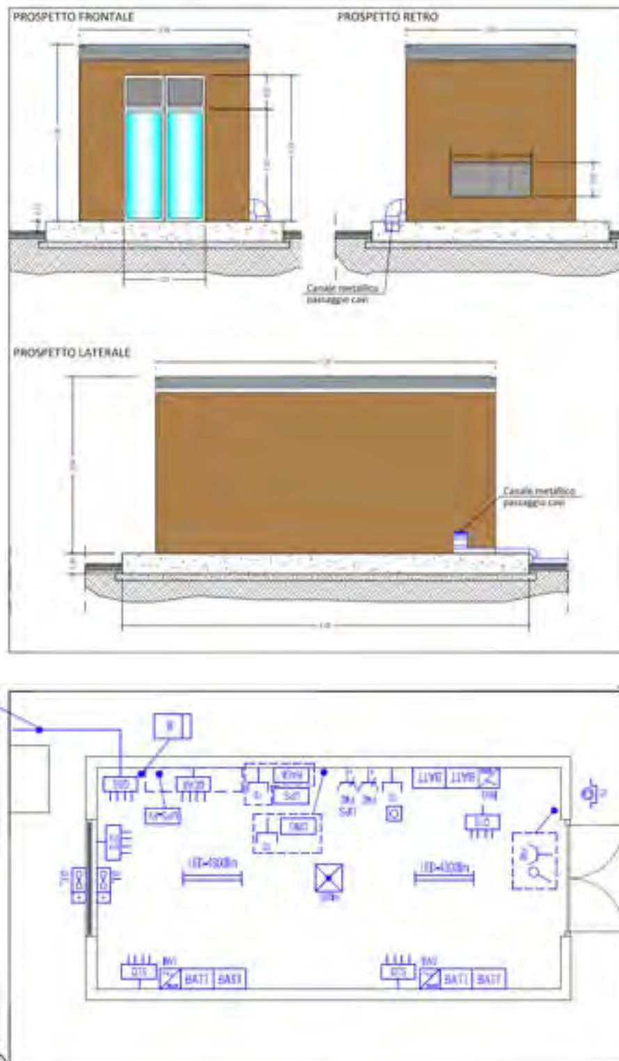
Figura 3. Cabina elettrica con le apparecchiature di potenza e dati.
