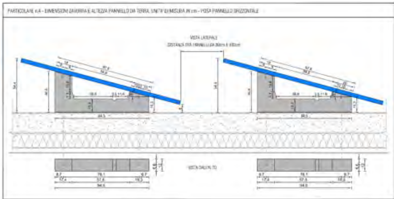
Figura 2. Particolari della zavorra utilizzata.
