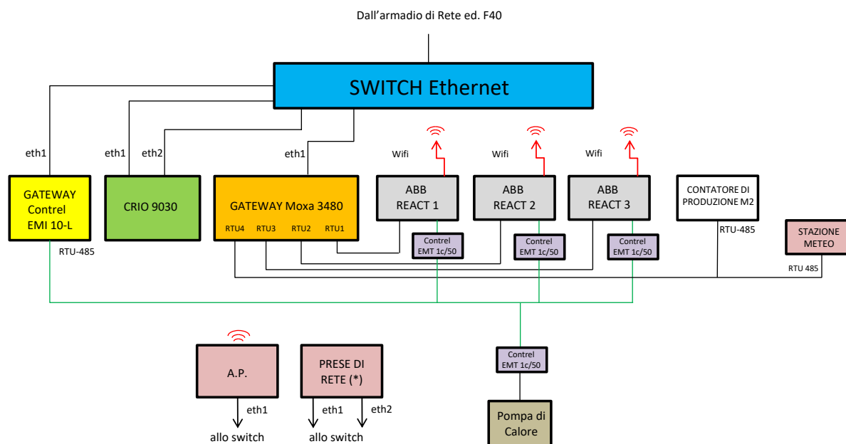
Figura 8. Schema della catena di misura del Sistema Smart metering
