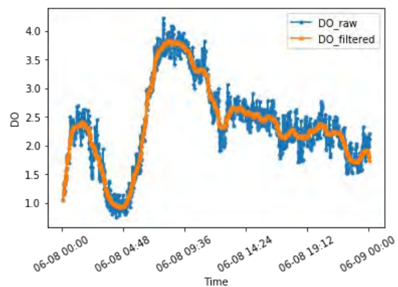
Figura 84: Andamento giornaliero DO
