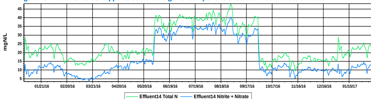
Figura 11- Andamento delle concentrazioni di azoto espresse come azoto totale e forme ossidate in uscita all'impianto
