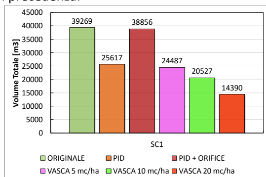
Figura 4: grafico relativo a volume (sinistra) e massa (destra) sversati nelle differenti configurazioni analizzate per lo scenario 1
