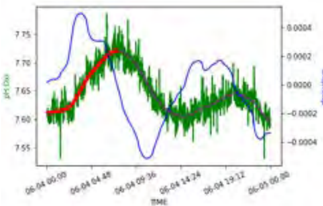
Figura 79: Massimo pH Ox alle Ore:Min= 07:36
