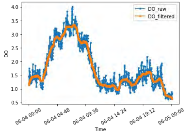
Figura 78: Andamento giornaliero DO
