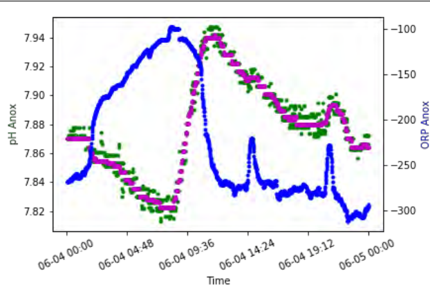
Figura 82: Andamenti corretti pH e ORP in vasca anossica
