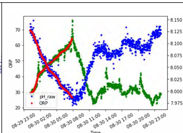
Figura 66: Valori non corretti di pH e ORP in vasca anossica. \text{ORP} > 0 \text{ mV}
