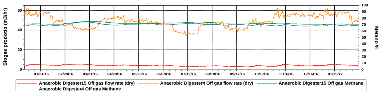
Figura 15 Produzione di biogas oraria e percentuale di metano.
