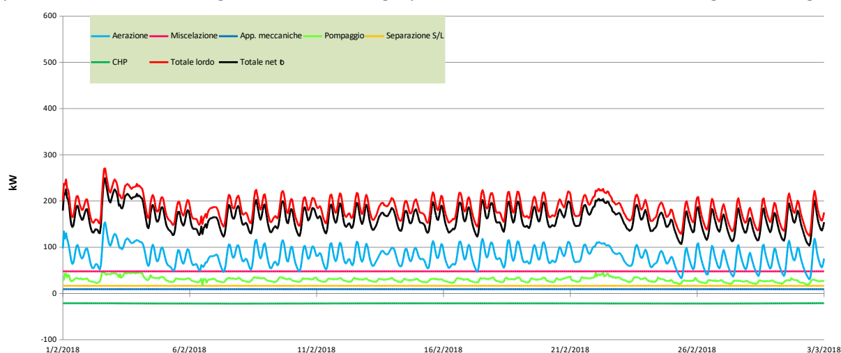
Figura 49: Andamento nel tempo delle potenze richieste dalle utenze dell'impianto nello scenario EFF3.
