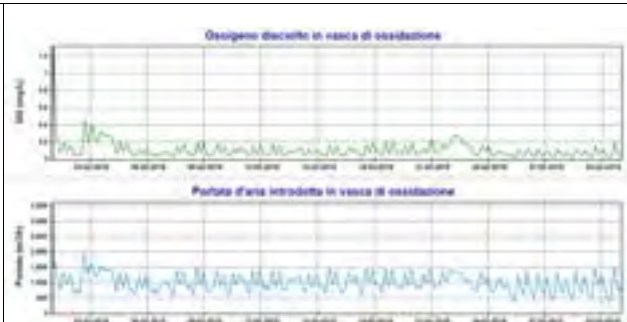
Figura 47: EFF2 controllore basato sulla misura dell'ossigeno e dell'ammoniaca (set point ammoniaca di 2 mg/l)
