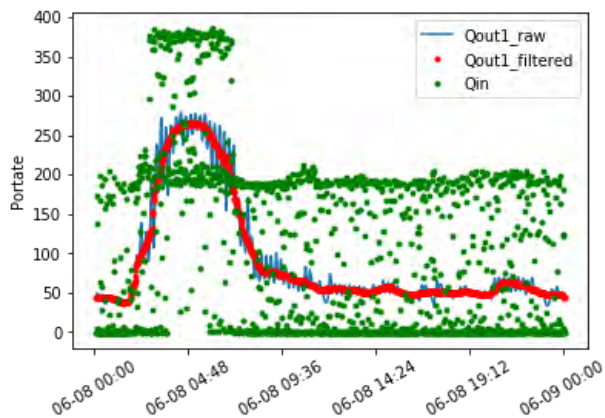
Figura 83: Portata giornaliera in ingresso linea 2
