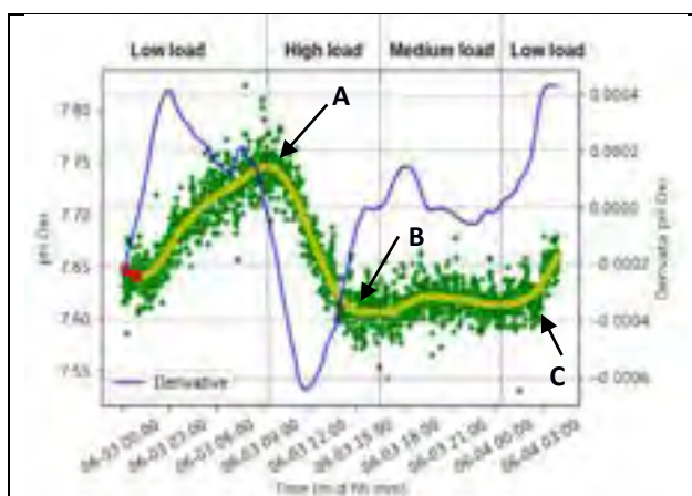
Figura 69: Andamento pH in vasca oxi del 3 giugno 2018
