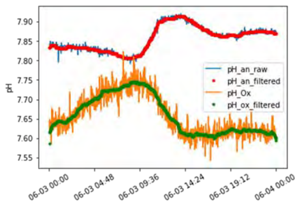
Figura 68: Rilevamento corretto funzionamento processo di denitrificazione: pH anox sempre > pH Ox
