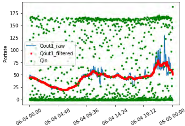
Figura 77: Portata in ingresso giornaliero linea 2
