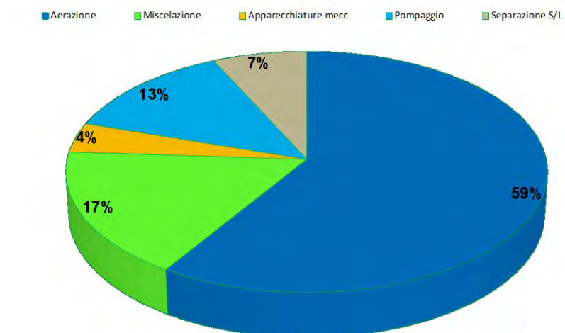
Figura 43: ripartizione percentuale dei consumi tra le diverse utenze dell'impianto nello scenario EFF1.
