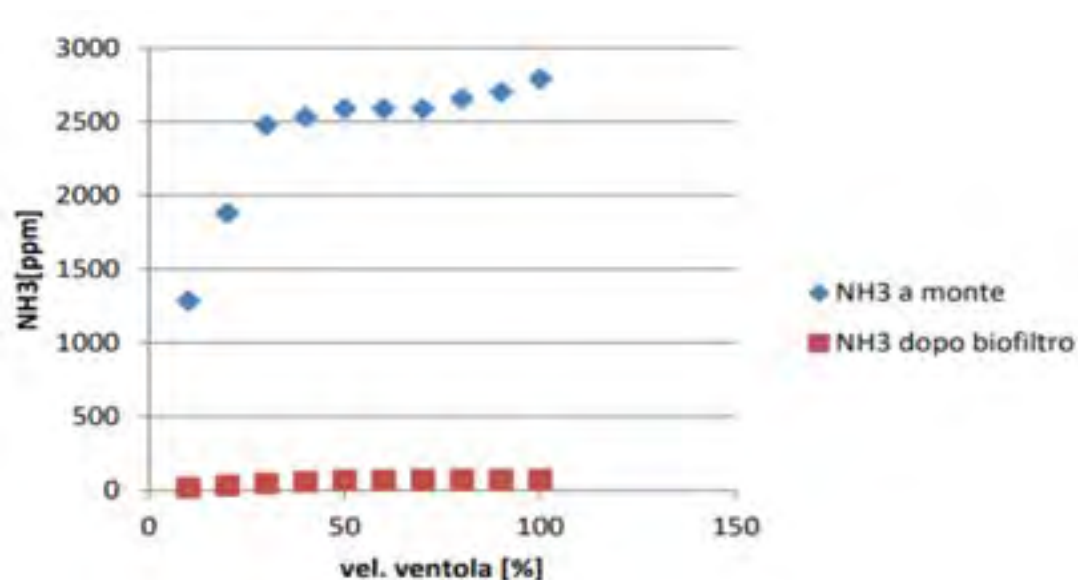
Figura 120: Concentrazioni ammoniaca prima e dopo il biofiltro al variare della velocità della ventola
