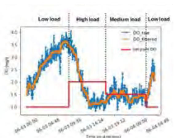
Figura 70: Andamento DO in vasca oxi del 3 giugno 2018
