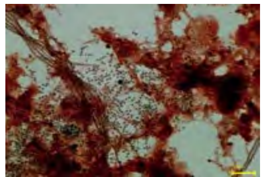
Figura 24 Flocchi di fango con microrganismo filamentoso Microthrix parvicella , evidenziato dalla colorazione di Sudan II il microrganismo e' positivo alla colorazione di Sudan evidenziato dai filamenti scuri. DIC, ingrandimento 1000X
