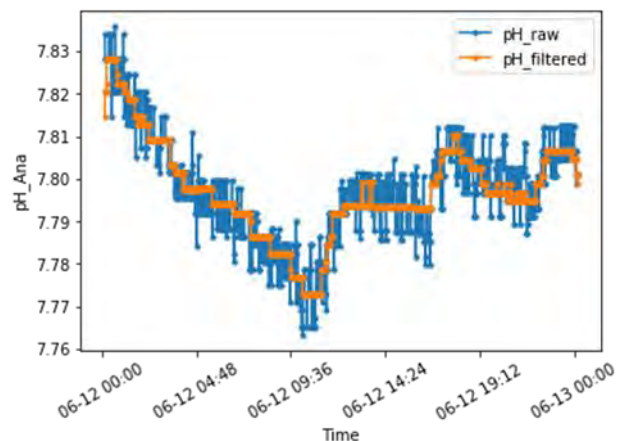
Figura 92: Andamento giornaliero pH anossico
