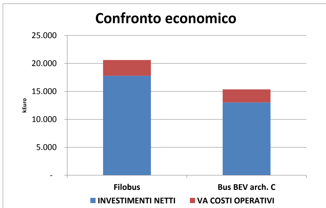
Figura 26: Confronto economico delle soluzioni tecnologiche: filobus e architettura C
