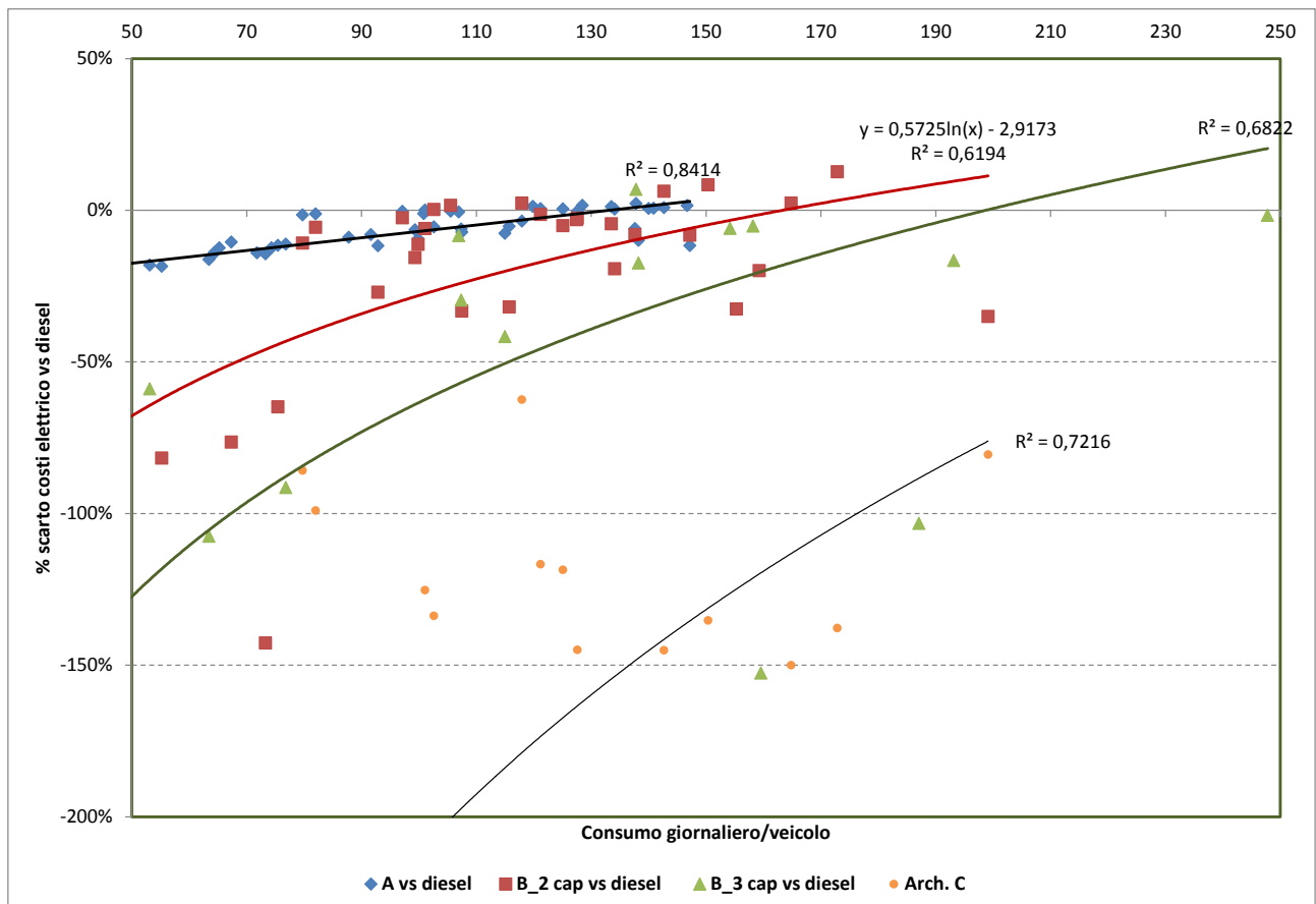
Figura 18: Correlazione tra scarto costi interni elettrico A e B vs diesel e consumo giornaliero/veicolo in presenza di effetto rete per B
