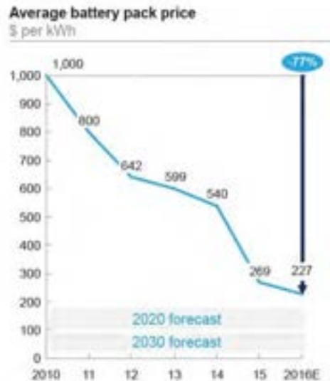
Figura 1: Prezzo medio del pacco batteria per veicoli elettrici. Fonte: McKinsey 2017
