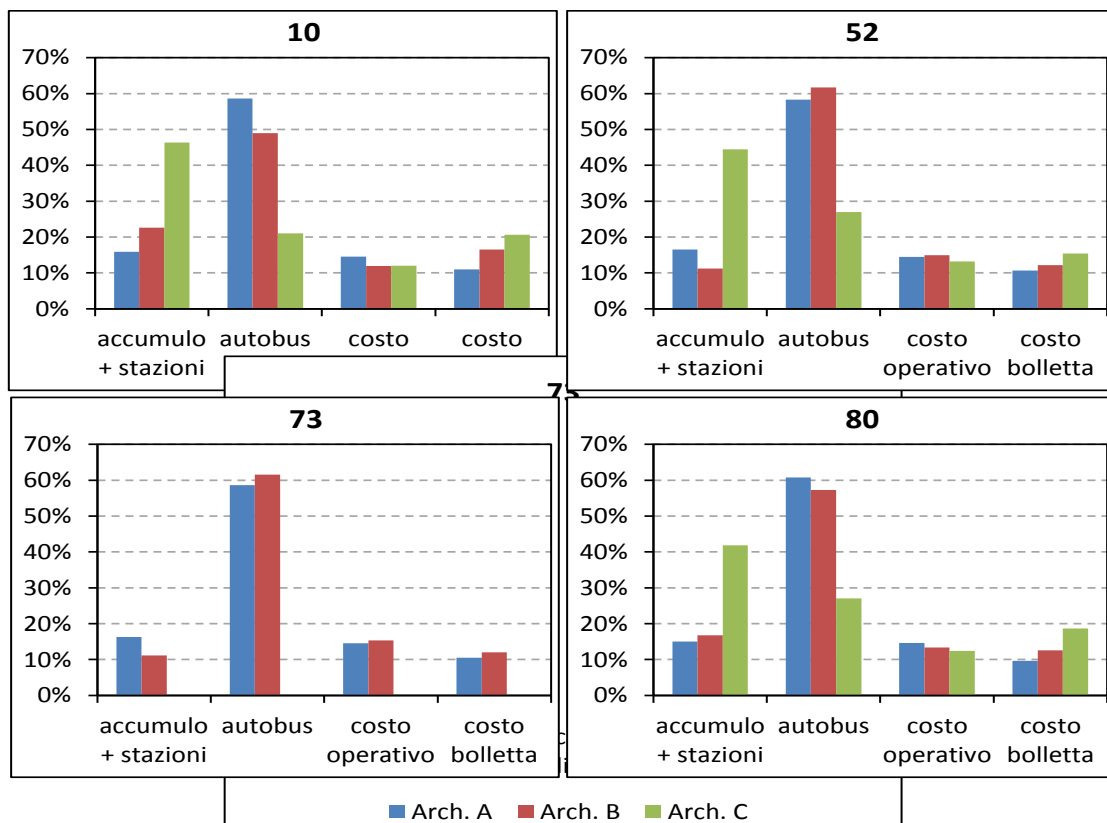
Figura 23: Percentuale tra diverse voci di costo per le varie alternative tecnologiche.
