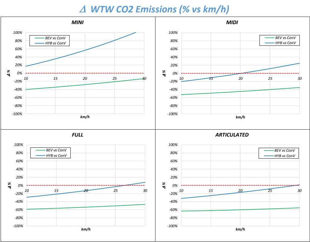
Figura 17 – Curve “pesate” di Variazioni Emissioni specifiche di CO2 WTW rispetto al caso base
