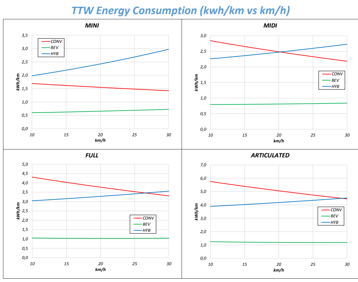
Figura 14 – Curve “pesate” di Consumo specifico di energia TTW
