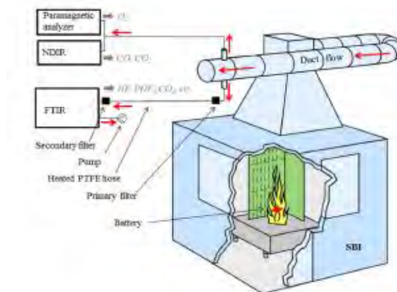
Figura 14. Apparato sperimentale per i test di abuso termico.
