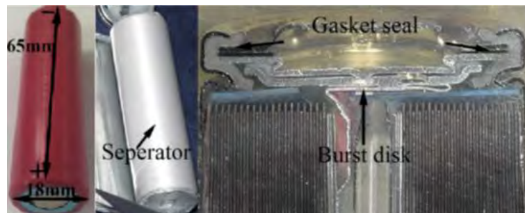
Figura 11. Struttura della batteria litio-ione
