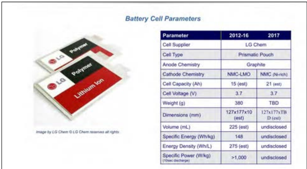
Figura 45. Celle utilizzate (Fonte: Total Battery Consulting) [22]
