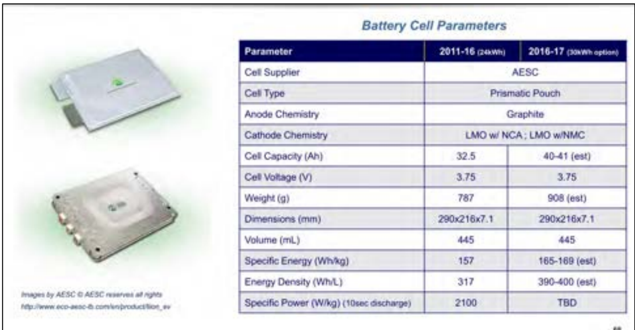
Figura 41. Celle utilizzate (Fonte: Total Battery Consulting) [22]
