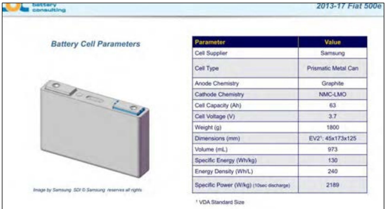
Figura 29. Celle utilizzate (Fonte: Total Battery Consulting) [22]
