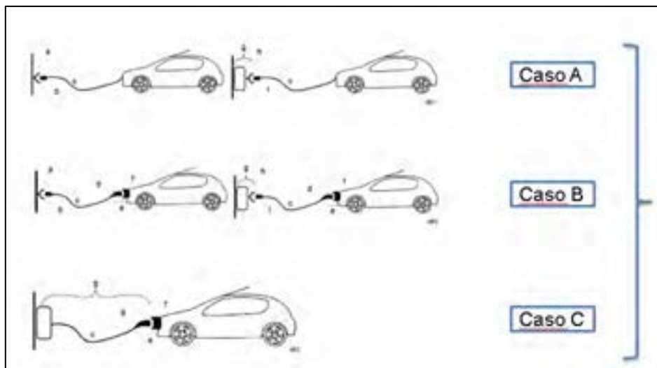
Figura 14. Tipi di Connessione (Fonte: [18 ])
