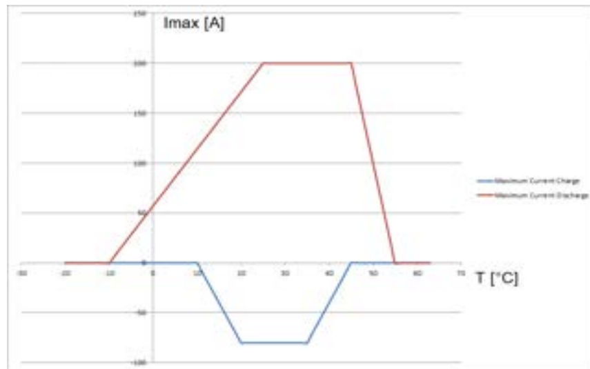
Figura 13 Curva di deterioramento della corrente massima di cella in funzione della temperatura
