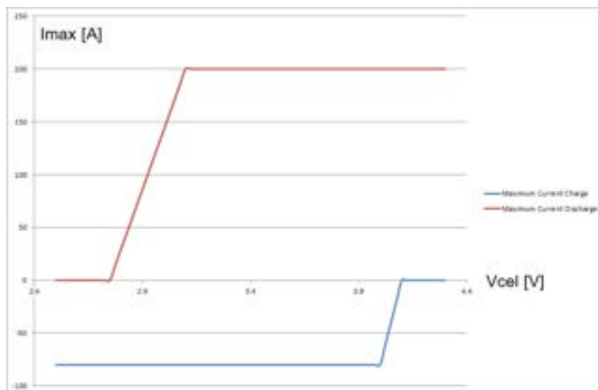
Figura 14 Curva di deterioramento della corrente massima di cella in funzione della tensione
