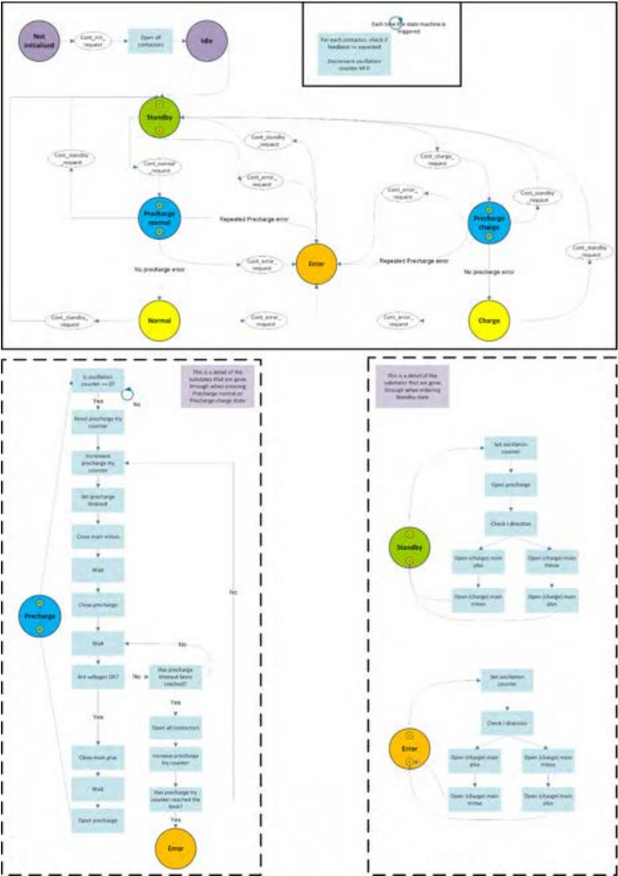
Figura 11 Stati del modulo "COUNT"
