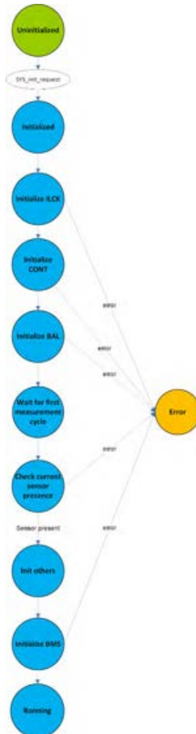
Figura 9 Stati del modulo "SYS"
