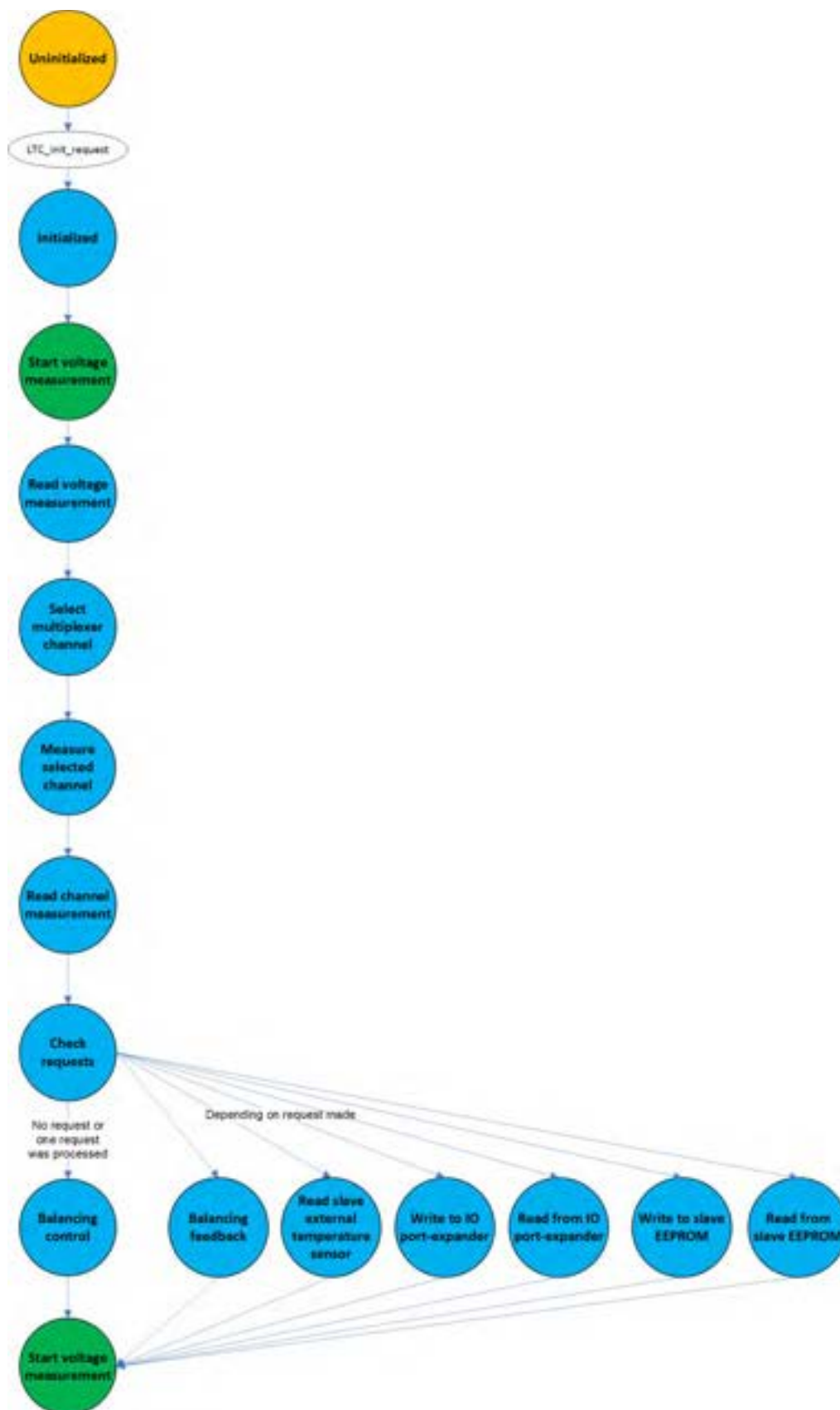
Figura 12 Stati del modulo "LTC"
