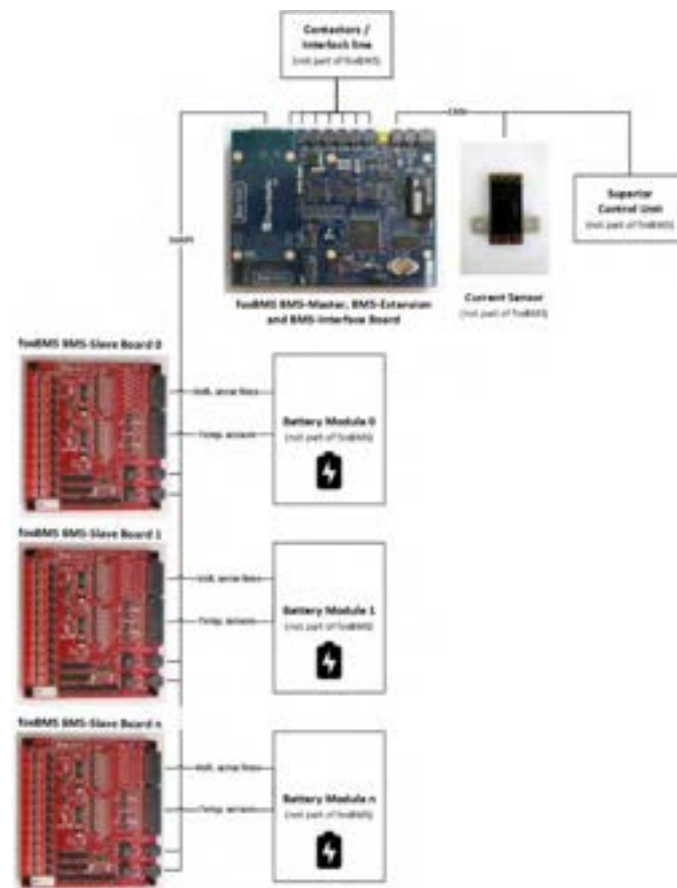
Figura 1 Architettura gerarchica del fox-BMS.
