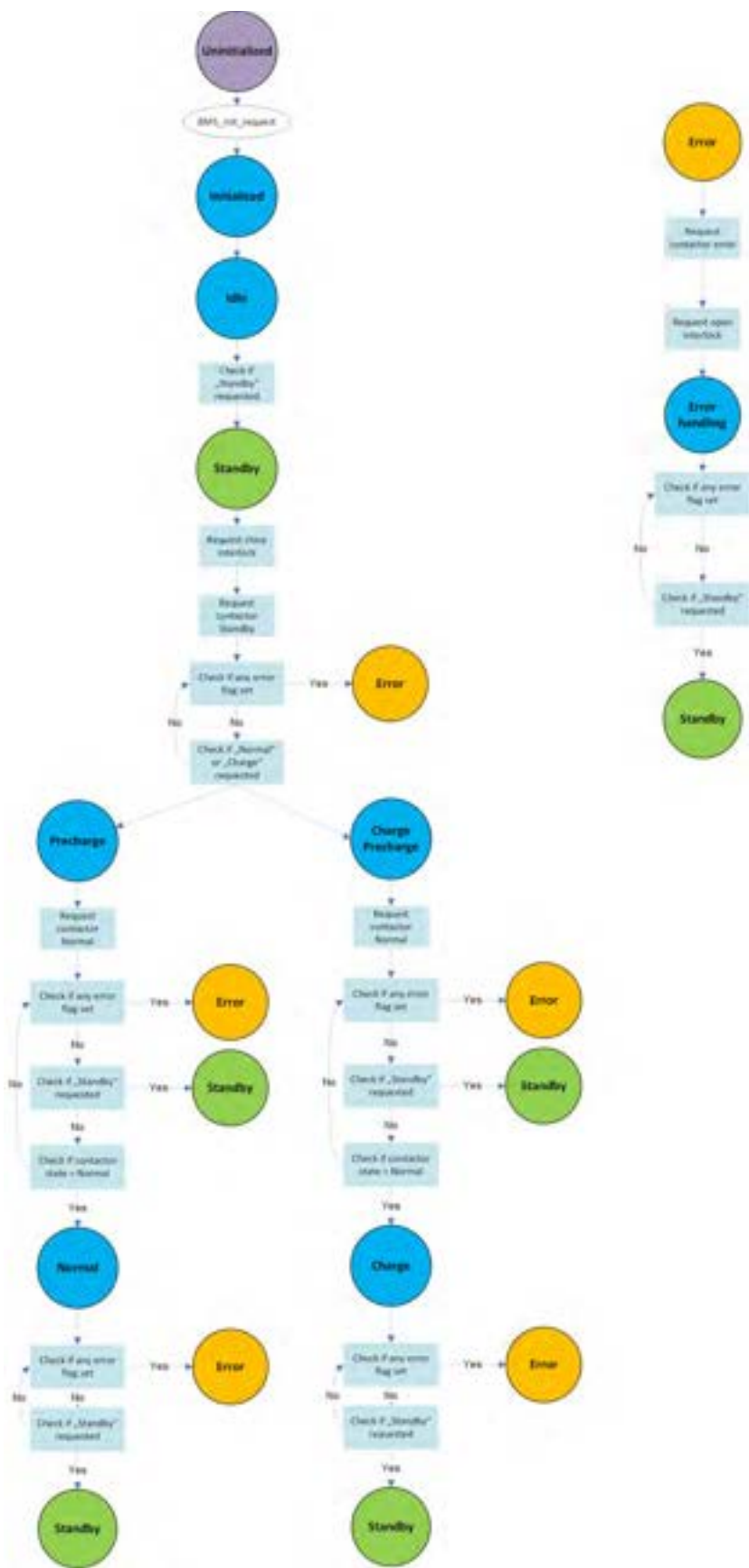
Figura 10 Stati del modulo "BMS"
