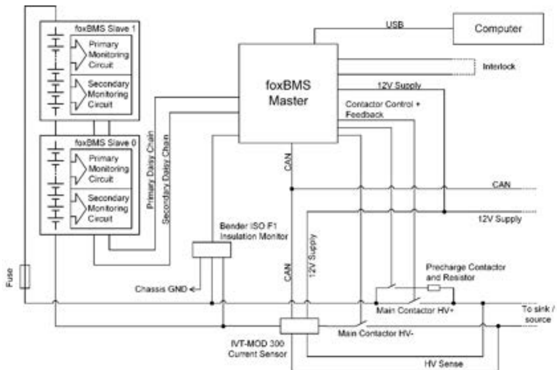
Figura 2 Configurazione del sistema fox-BMS
