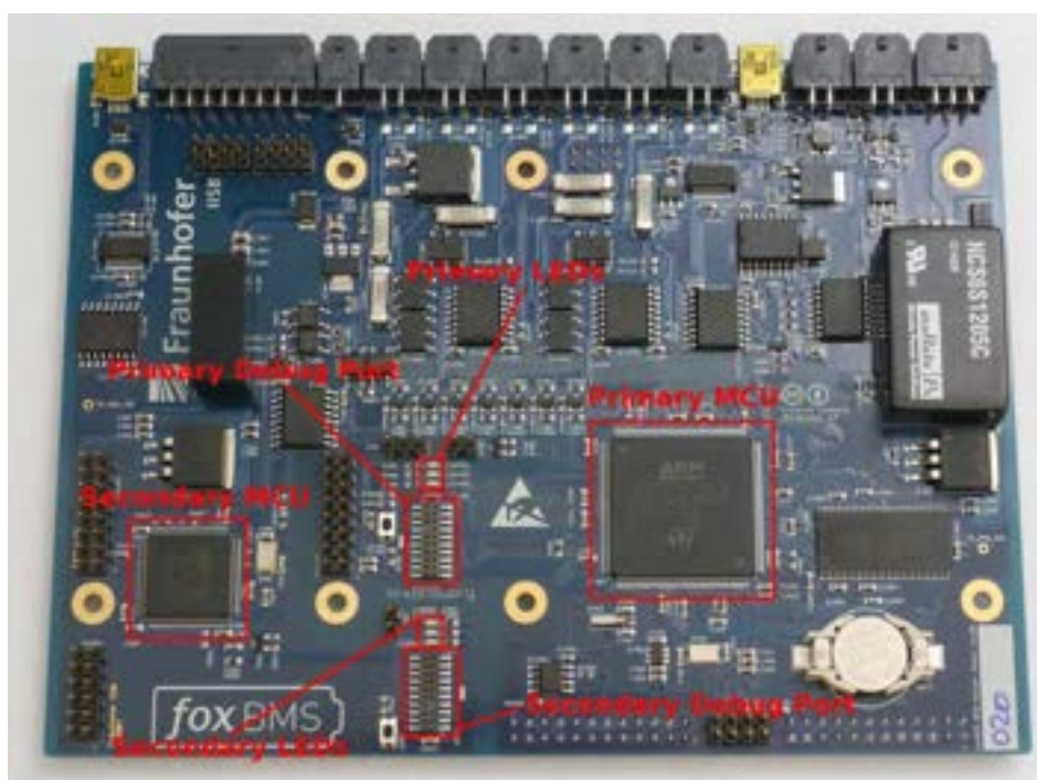
Figura 3 Circuito stampato BMS-Master
