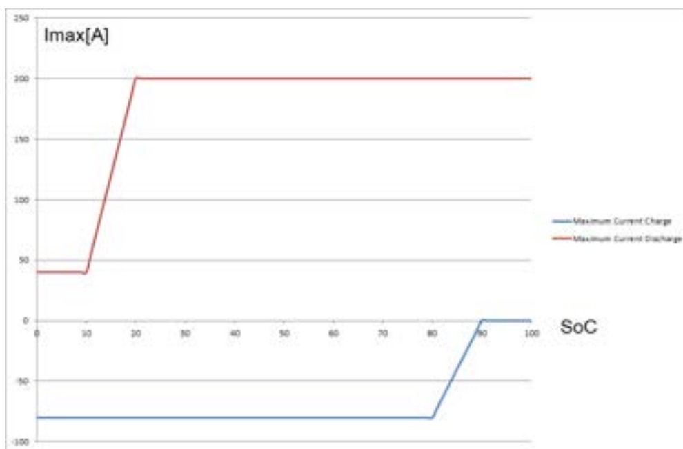
Figura 15 Curva di deterioramento massima della corrente cella in funzione dello SoC
