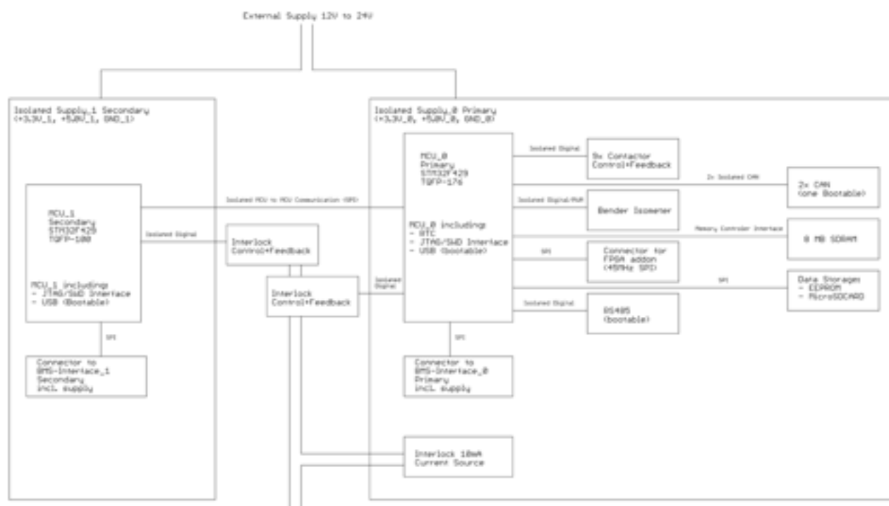
Figura 4 Architettura hardware BMS-Master.
