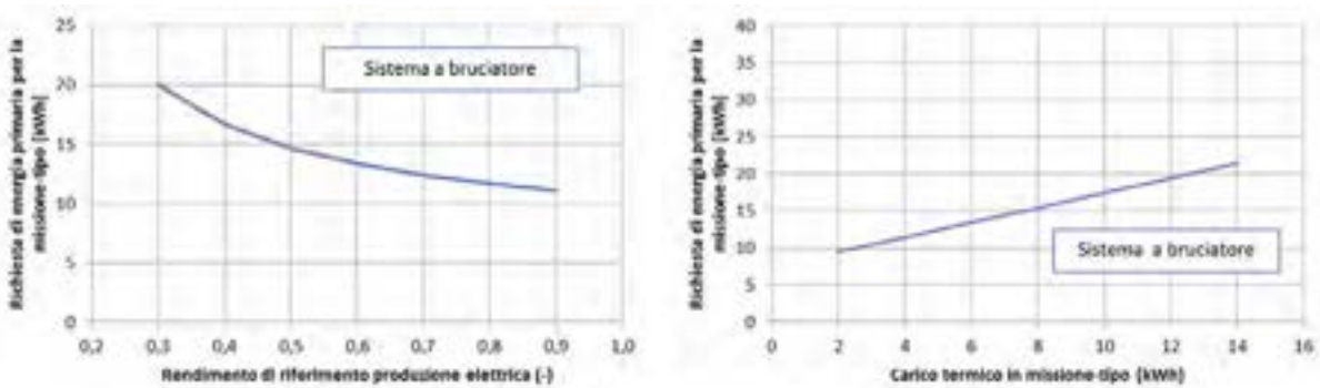
Figura 11: Sistema a bruciatore – Richiesta di energia primaria per la missione-tipo – Andamento in funzione del rendimento elettrico di riferimento, sinistra; Andamento in funzione del carico termico, destra
