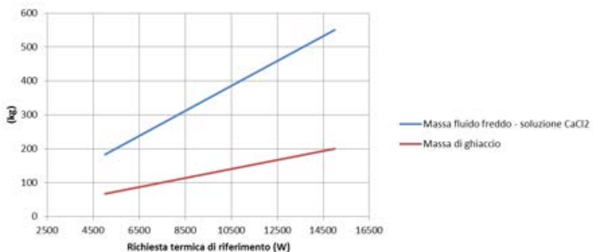
Figura 9: Andamento della massa di soluzione di cloruro di calcio \text{CaCl}_2 in accumulo al variare della richiesta termica di riferimento – Andamento della massa di ghiaccio in accumulo al variare della richiesta termica di riferimento
