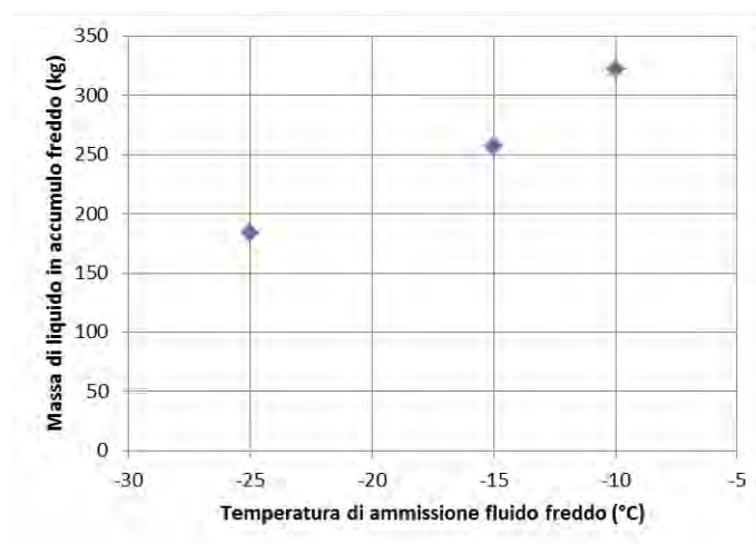
Figura 8: Andamento della massa di soluzione di cloruro di calcio \text{CaCl}_2 in accumulo al variare della temperatura minima di stoccaggio
