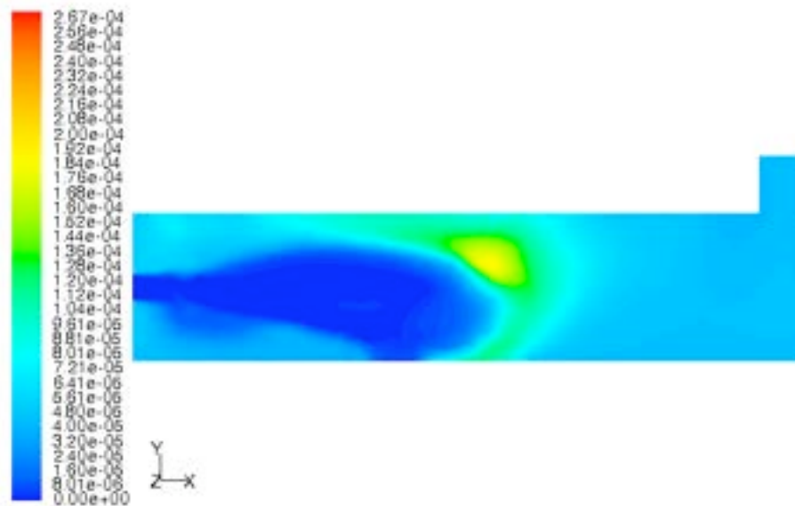
Fig. 46 Frazione di massa di OH. Incremento della portata dei gas riciclati del 100% e della temperatura a 800K. Granulometria fine. Modello FGDCV.
