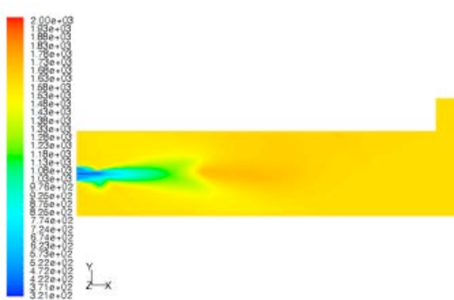
Fig. 44 Temperature (K). Incremento della portata dei gas riciccolati del 30%. Granulometria fine. Modello FGDCV.
