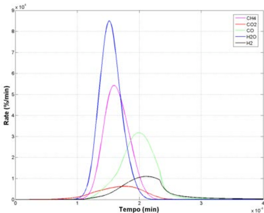
Fig. 4 Tasso di produzione delle specie gassose (4atm).
