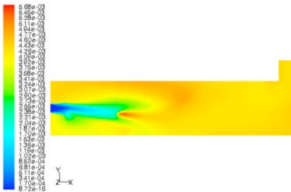
Fig. 50 Frazione di massa di SO x . Incremento della portata dei gas riciclati del 100% e della temperatura a 800K. Granulometria fine. Modello FGDVC.
