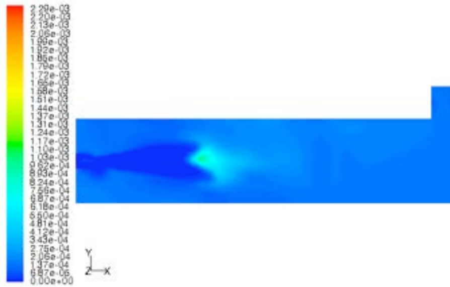
Fig. 46 Frazione di massa di OH. Incremento della portata dei gas riciclati del 30%. Granulometria fine. Modello FGDCV.
