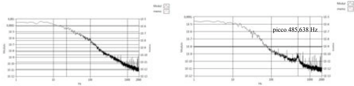
Figura 16 Spettri medi. Sinistra CH0. Destra CH1
