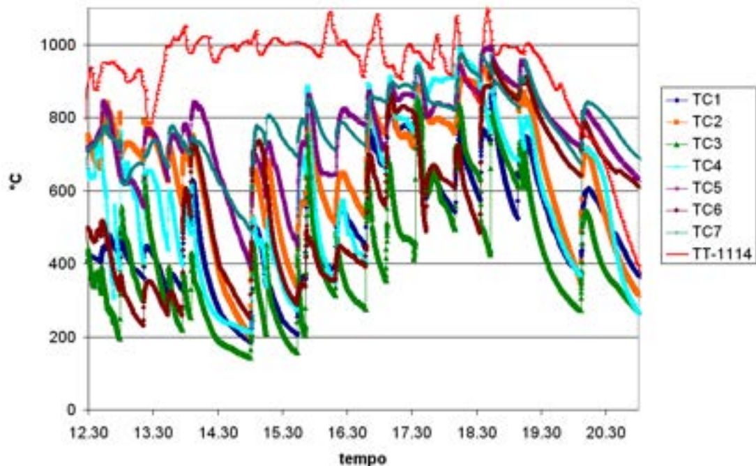
Fig. 26: Andamento nel tempo delle termocoppie alloggiate sulla griglia, avviamento del 18/05/2010
