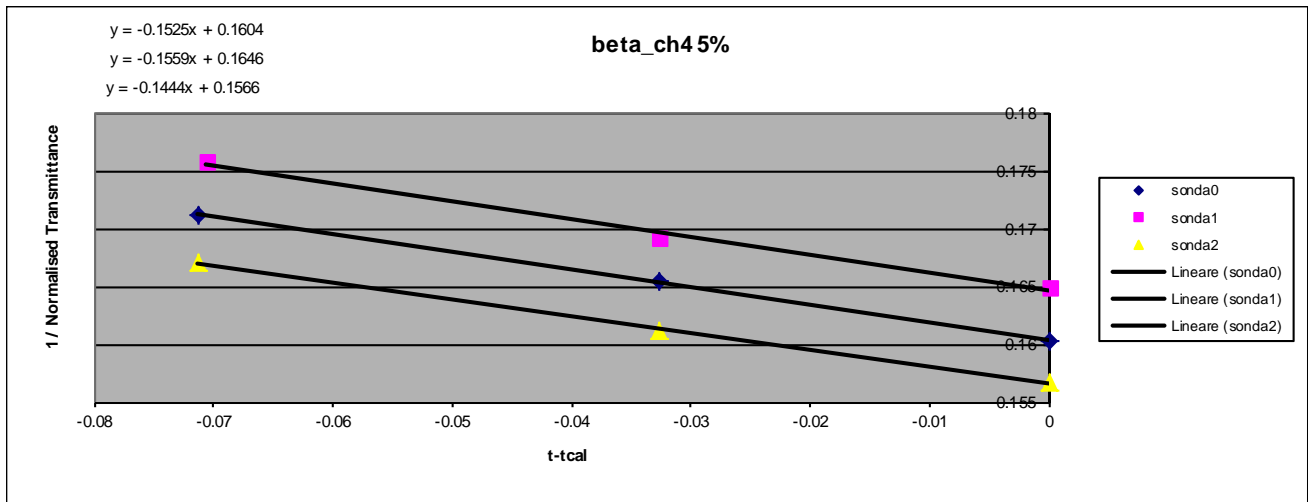
Figura 11b. Variazione dei valori di trasmittanza con la temperatura per concentrazioni di metano pari al 5% (span).
