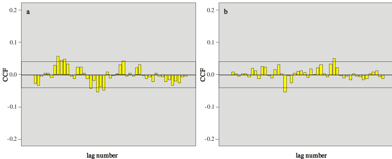
Figura 6. Per la determinazione della correlazione tra concentrazione di anidride carbonica e temperatura bisogna osservare nel grafico il superamento (positivo o negativo) dell’intervallo di confidenza rappresentato dalle 2 righe nere. Tra tutti i casi in cui questo intervallo viene superato, bisogna selezionare quello in cui questo superamento è più marcato. In questo caso questa condizione può essere osservata per un lag pari a -4 nel primo caso (profondità 1.5 m – figura a) e per un lag pari a -7 nel secondo caso (profondità 0.8 m – figura b).
