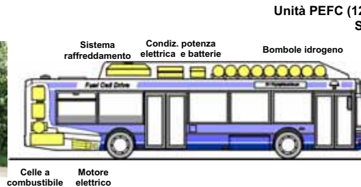
MAN - Progetto Fuel Cell Bus Potenza: 120 kW stack Siemens/ batteria Autonomia: 250 km Velocità: 80 km/h Combustibile: idrogeno (250 bar)
