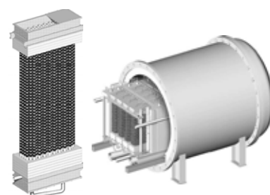
Struttura del modulo SOFC pressurizzato
