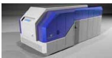
Unità da 250 kW (conceptual design) Combustibile: gas naturale, metanolo, biogas Efficienza elettrica attesa: ~ 50 %
