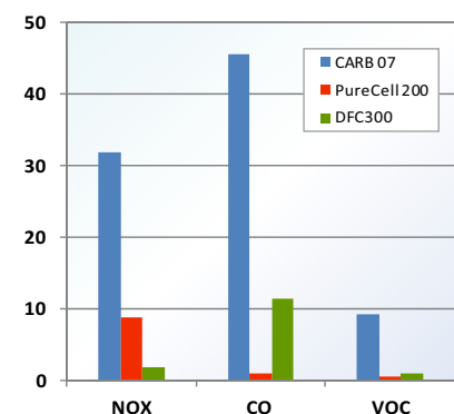
Emissioni impianti PureCell 200 e DFC300 confrontate con limiti CARB07 (g/MWh)
