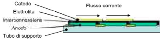
Cella Rolls-Royce
