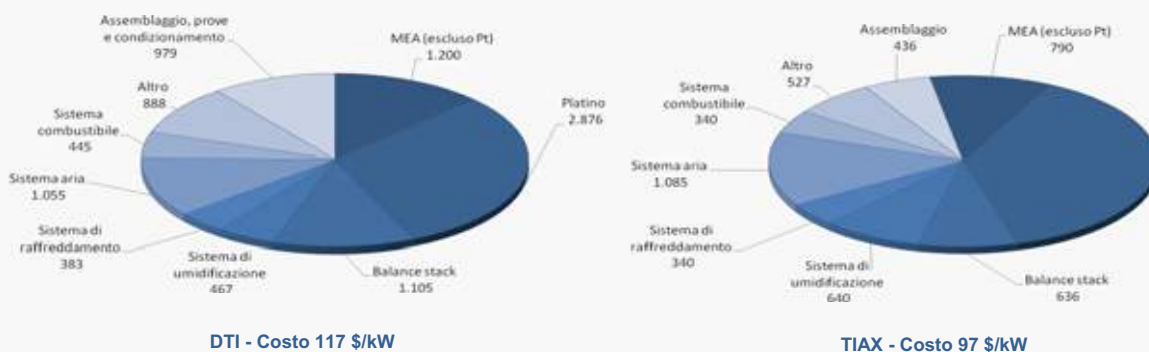
Sistema PEFC da 80 kW a idrogeno / Produzione 500.000 unità/anno (Fonte DoE, 2007)
