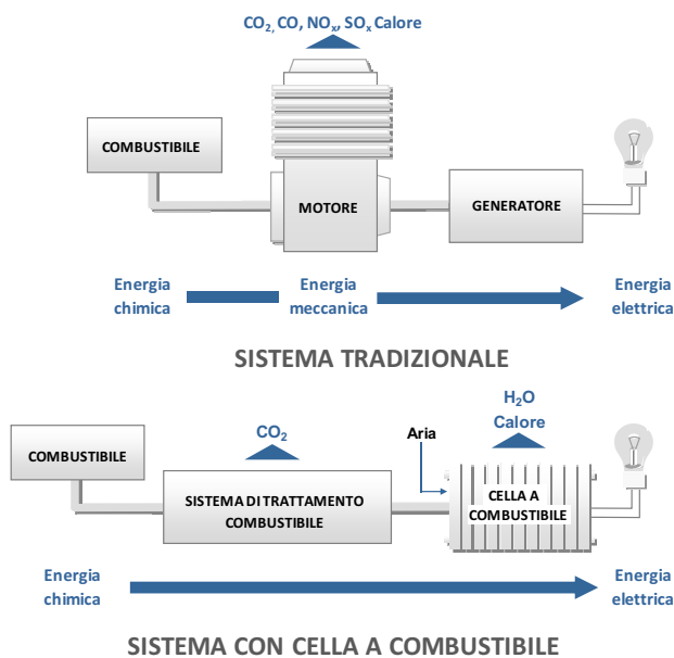
Conversione di energia - Confronto tra celle a combustibile e sistemi tradizionali
