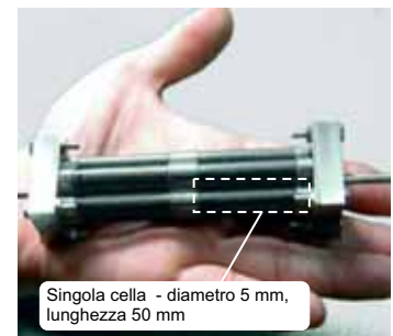
SOFC micro tubolari TOTO
