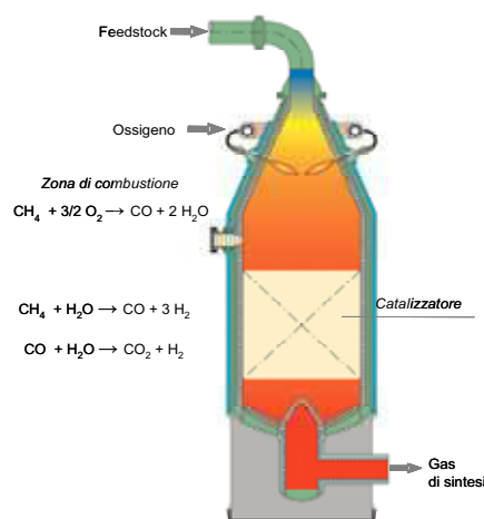
Reforming autotermico (ATR)
