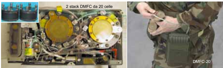
Unità portatile DMFC-20 LANL/Ball Aerospace (DARPA Palm Power Programme)
