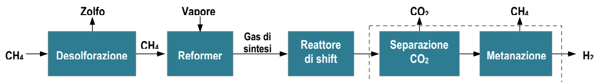
Diagramma di flusso semplificato di un impianto per la produzione di idrogeno per reforming del metano
