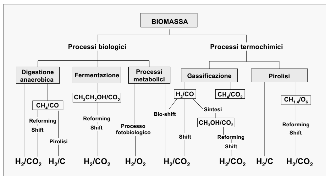
Produzione di idrogeno d biomasse
