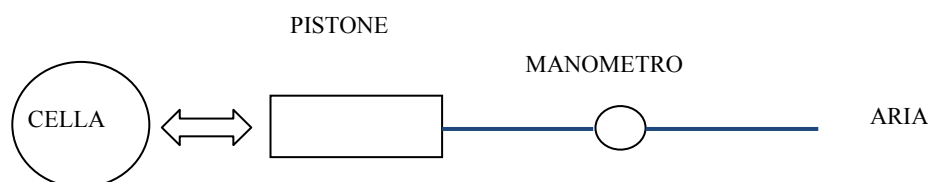
Figura 8. Schema di funzionamento del carico meccanico.
