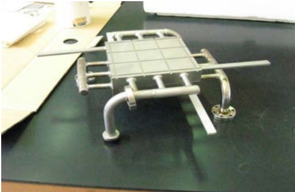
Figura 4. Monocella di tipo MCFC Ansaldo ARI.
