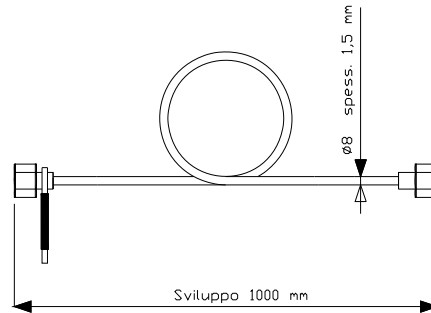
Figura 15. Serpentina flessibile.
