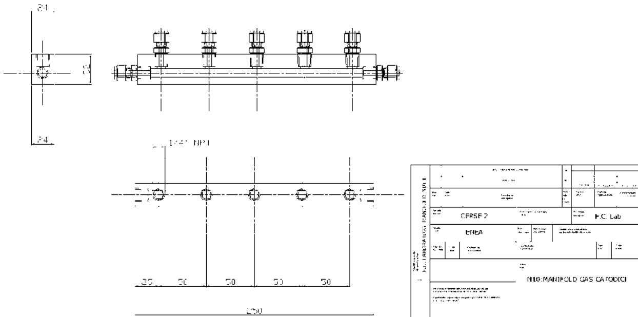
Figura 36. P&ID manifold catodico, inserito per migliorare le tenute e la miscelazione del gas catodico.
