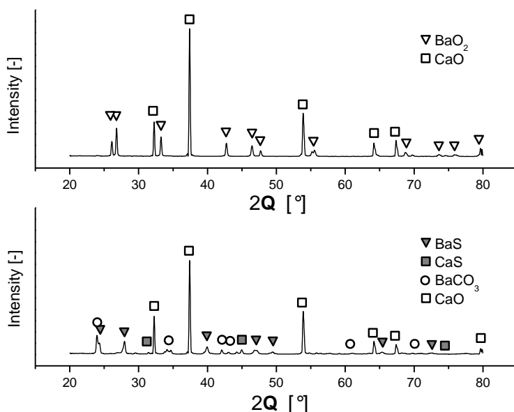
Figura 7: Analisi XRD del materiale assorbente CaBa prima e dopo il test di assorbimento di H 2 S
