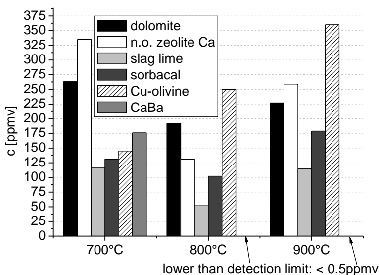
Figura 5: Concentrazione di H 2 S in uscita dal letto sorbente
