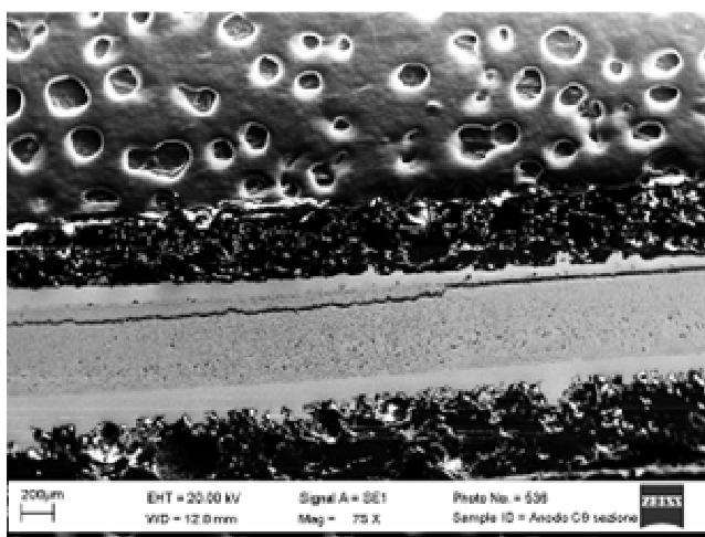
[Figura 32 75x SEM BSE Anodo C9 sezione: ben visibile la cricca]
