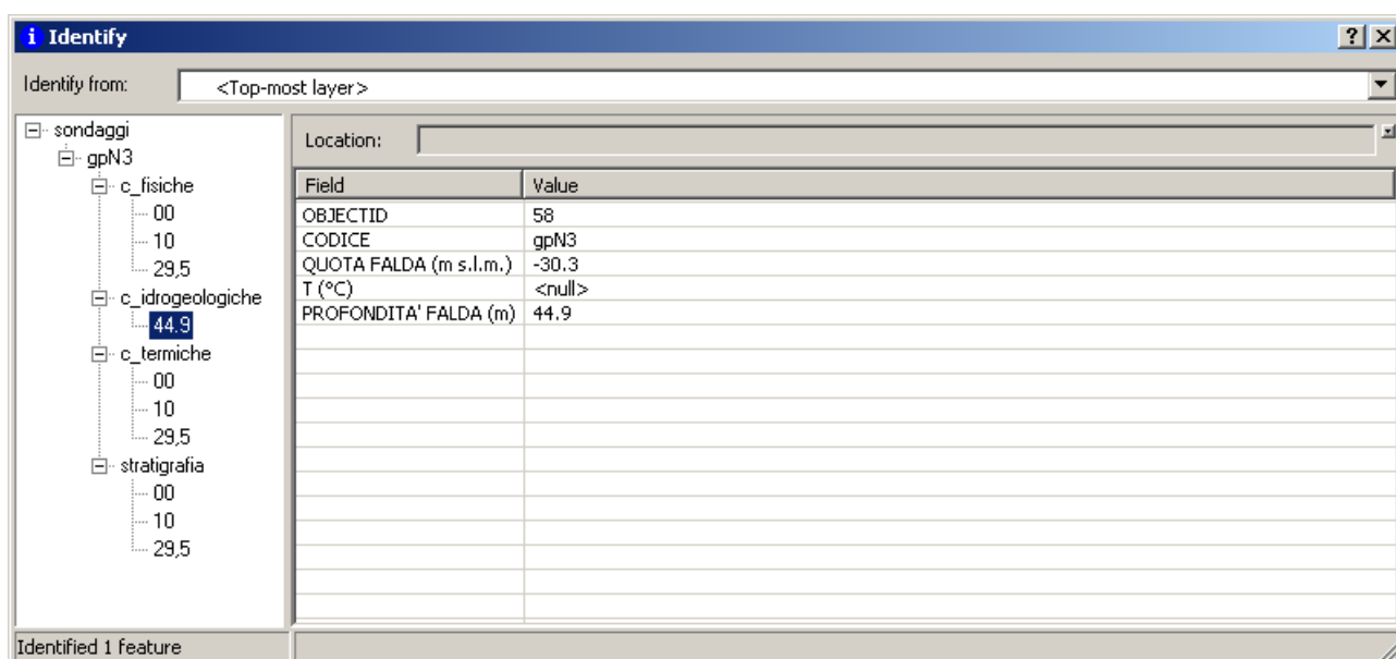
Fig.8 – attributi relativi alle caratteristiche idrogeologiche dedotte dalle descrizioni riportate nei log stratigrafici
