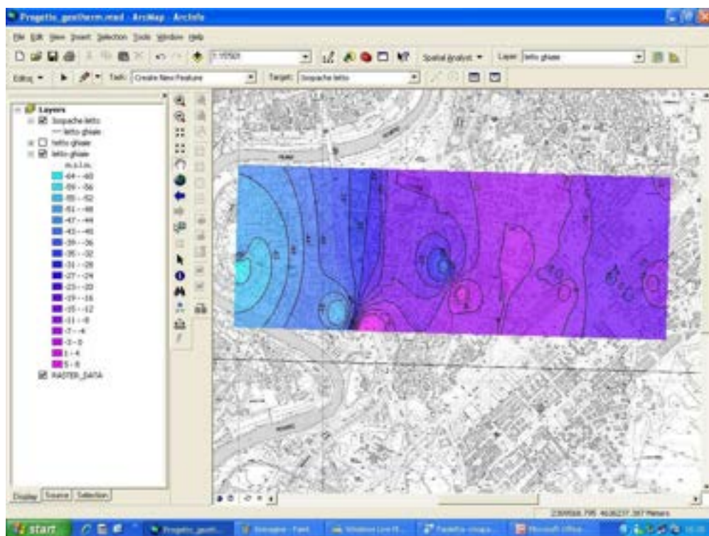
Fig.14 - distribuzione spaziale del letto dell'acquifero più produttivo e relative isobate
