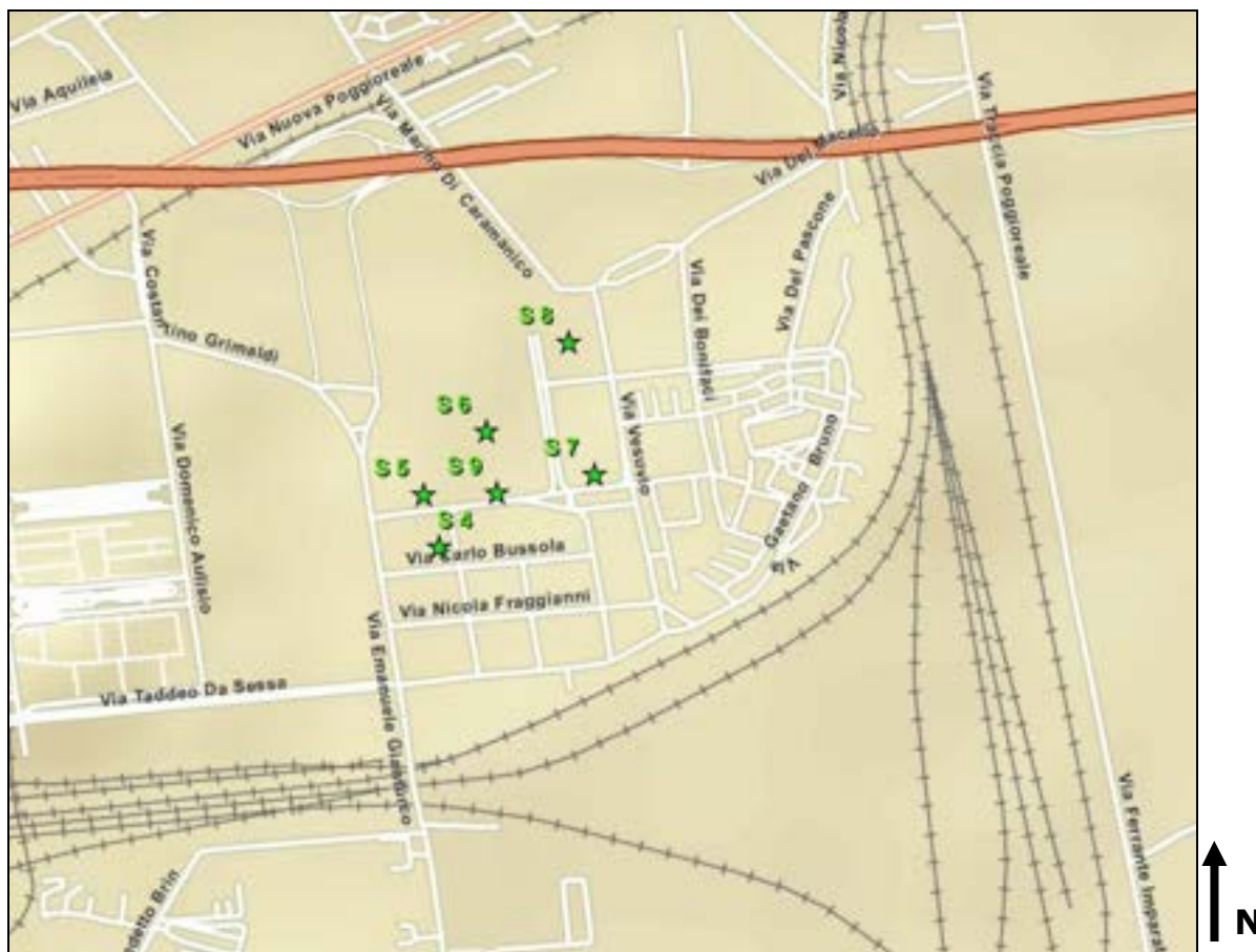
Fig.19 – ubicazione dei sondaggi geognostici nell'area del Centro Direzionale a Napoli
