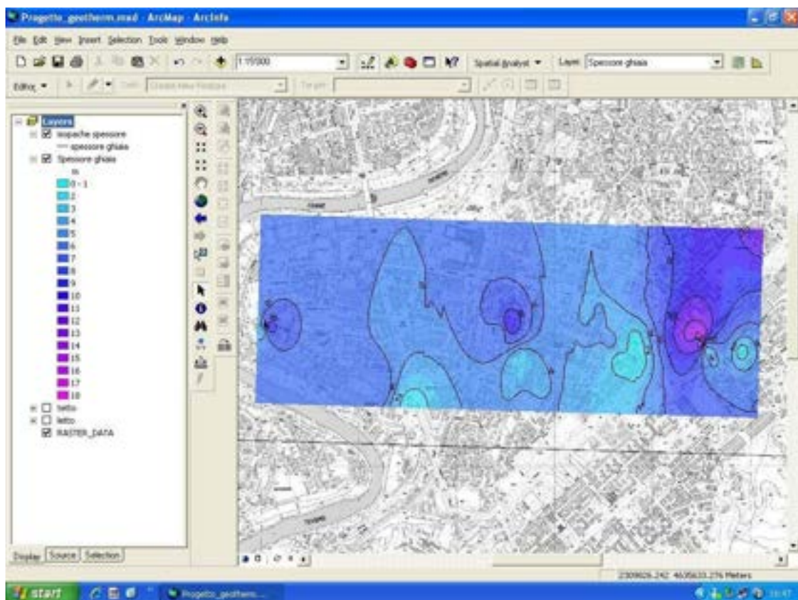
Fig.15 - distribuzione spaziale dello spessore dell'acquifero più produttivo e relative isopache
