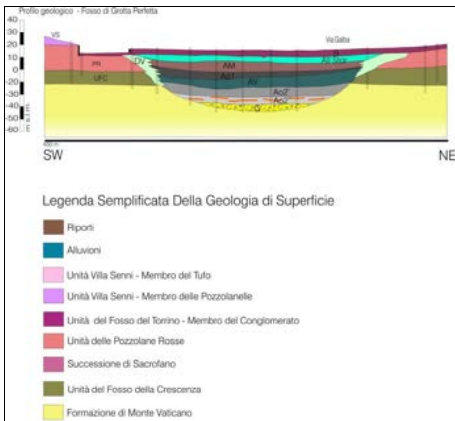
Fig. 16 - profilo geologico rappresentativo trasversale al Fosso di Grotta Perfetta
