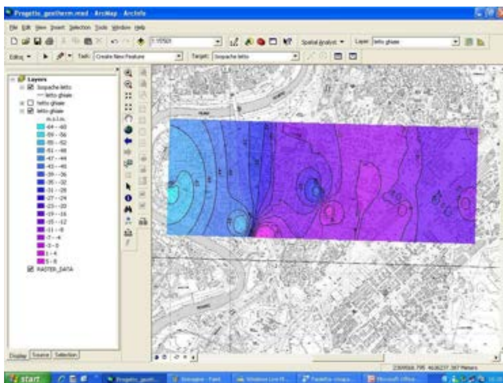
Fig.14 - distribuzione spaziale del letto dell'acquifero più produttivo e relative isobate
