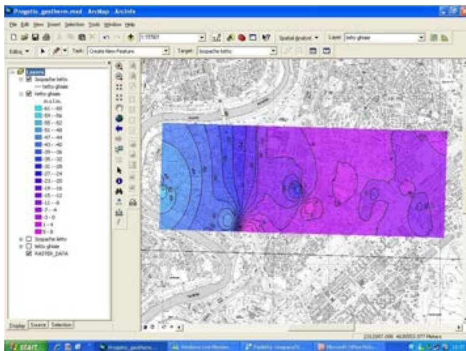
Fig.13 – distribuzione spaziale del tetto dell’acquifero più produttivo e relative isobate
