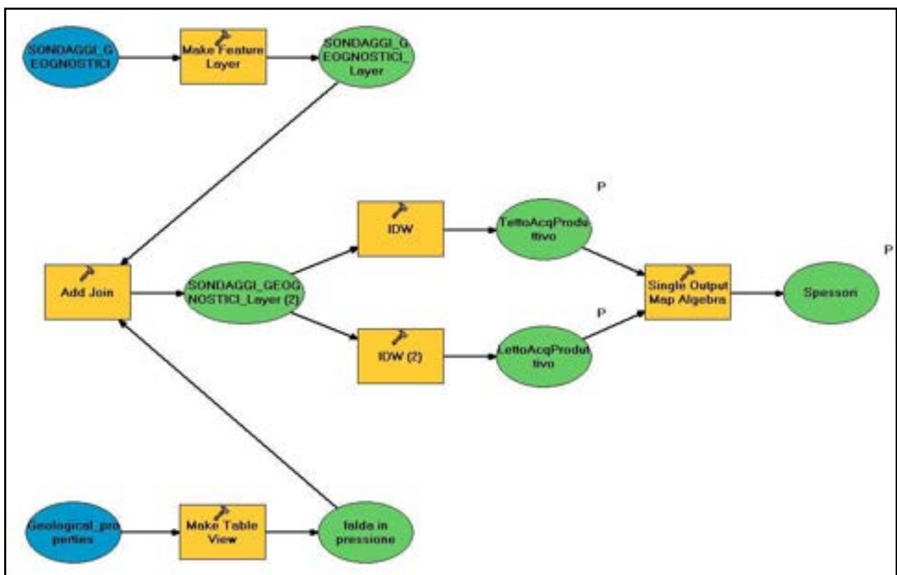
Fig.11 – modello di analisi per la ricostruzione del tetto, del letto e dello spessore dell'acquifero più produttivo.
