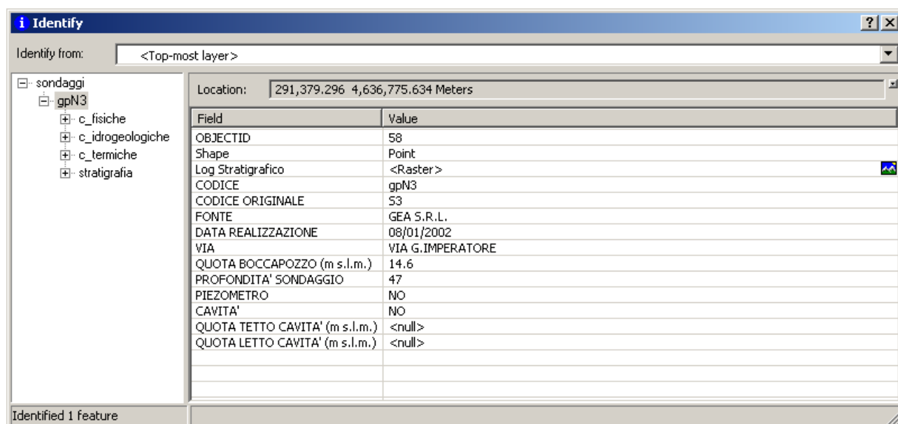
Fig.6 – attributi associati al sondaggio geognostico
