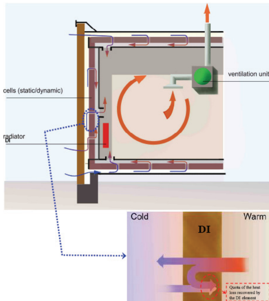
Fig. 11 – Principio di funzionamento dei DI
