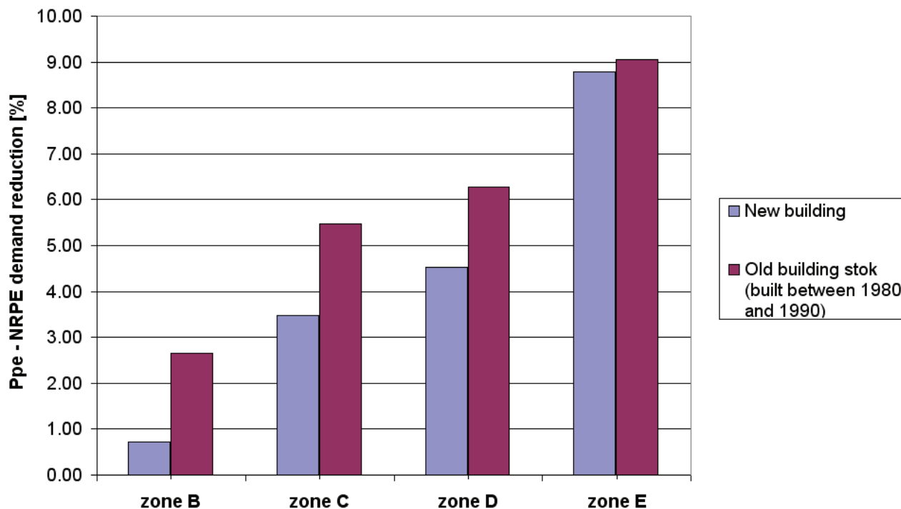
Fig. 5 – Percentuale di riduzione di NRPE per edifici esistenti ed edifici nuovi
