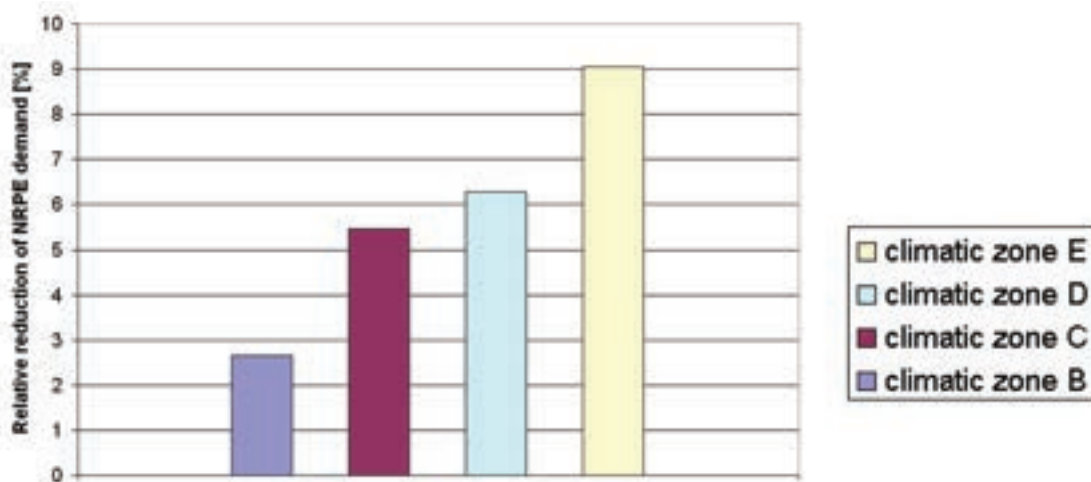
Fig. 3 – Percentuale di riduzione della domanda di NRPE indotta dal sistema CHP rispetto al sistema convenzionale: caldaia standard (per riscaldamento ed acqua calda sanitaria) e mix di generazione elettrica.
