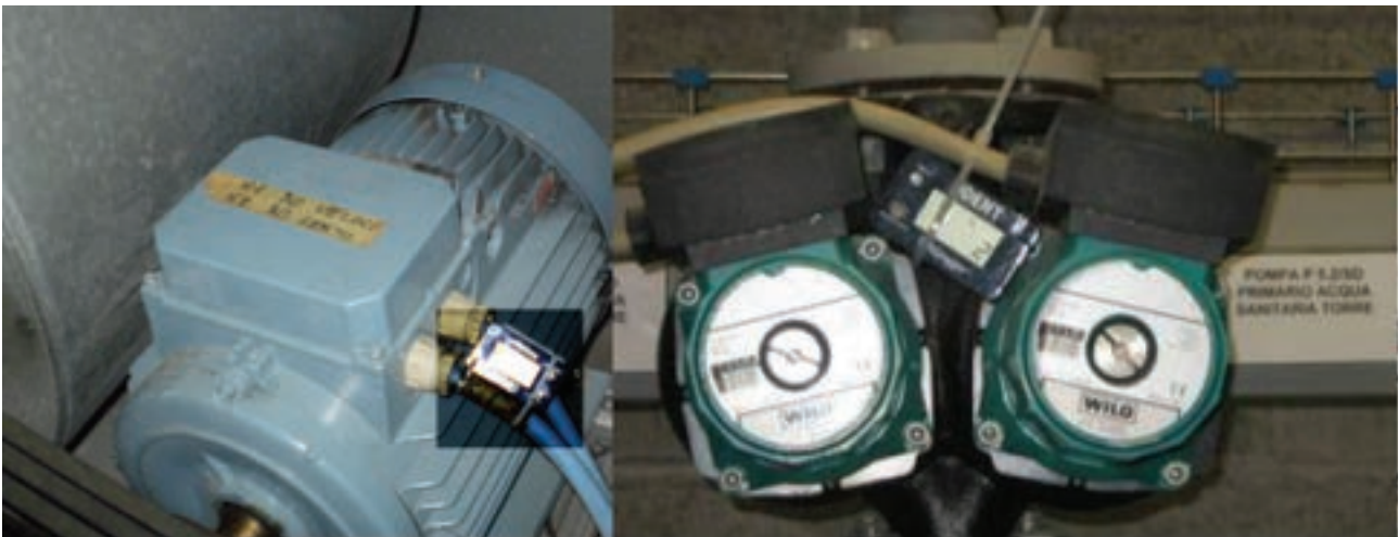
Fig. 21 - Tipiche installazioni di logger di stato. La foto di sinistra mostra un'installazione su un ventilatore di un UTA, a destra lo stesso strumento è stato applicato a delle pompe gemellari.
