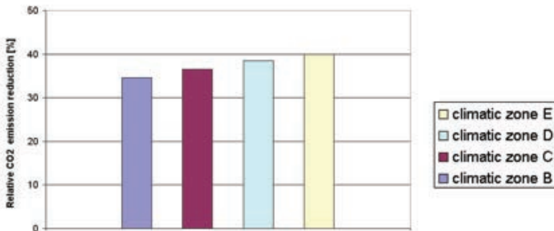
Fig. 4 – Riduzione delle emissioni di CO_2 del sistema di cogenerazione rispetto al sistema di riferimento
