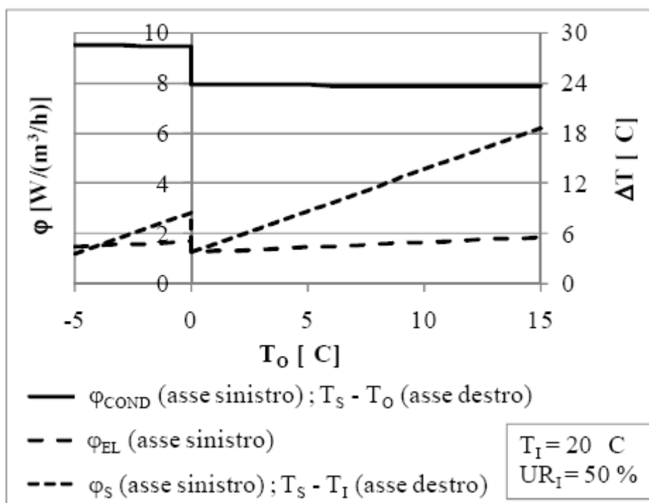
Fig. 24 - Potenza elettrica assorbita dal compressore ( \phi_{EL} ), potenza termica resa all'ambiente ( \phi_s ), potenza termica resa all'aria dalla batteria condensante ( \phi_{COND} ) per unità di portata d'aria trattata in funzione della temperatura esterna. Differenza di temperatura tra l'aria immessa e l'aria interna ( \Delta T_{s,i} ), e tra l'aria in immissione e l'aria esterna ( \Delta T_{s,o} ) in funzione della temperatura dell'aria esterna
