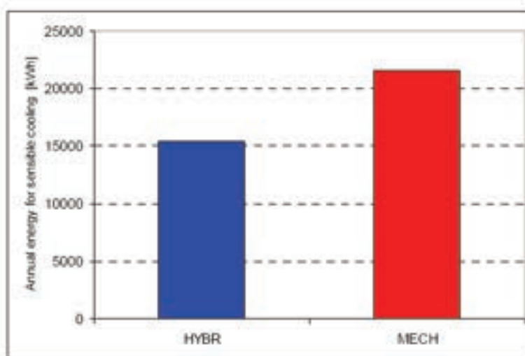
Fig. 31 - Risparmio energetico con ventilazione ibrida per il raffrescamento di una casa di cura di 3750 m 3
