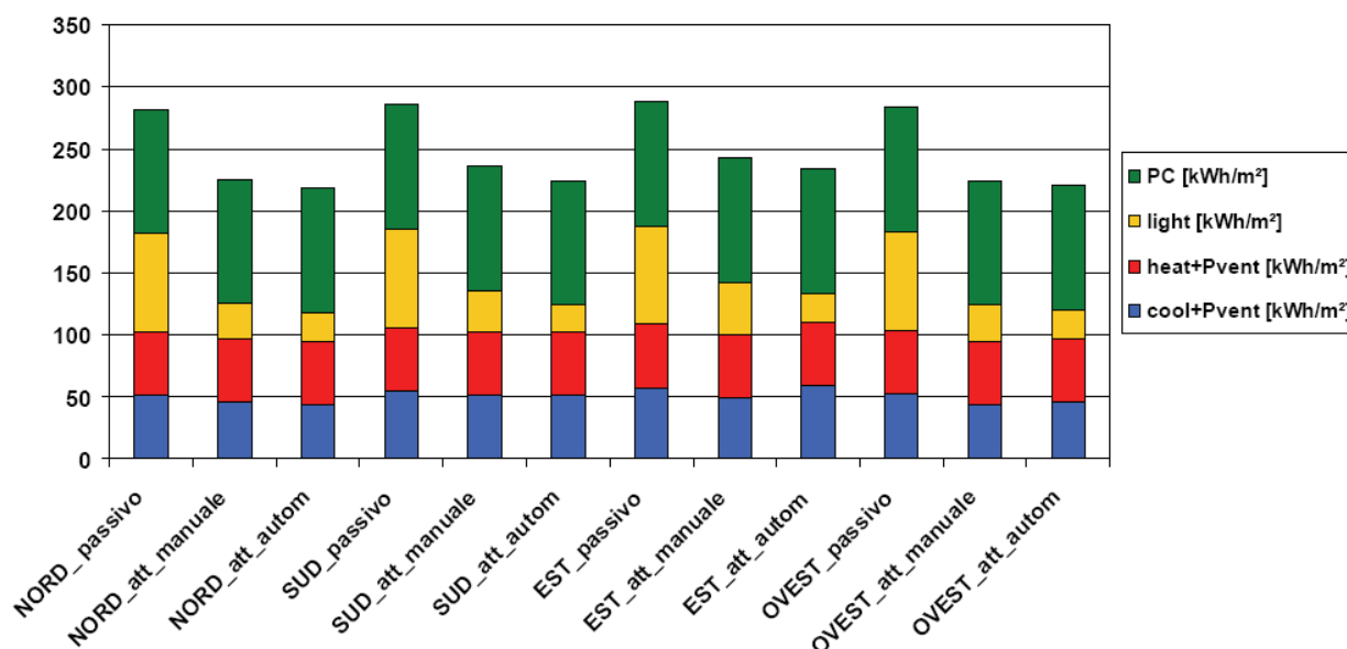
Fig. 32 - Consumi di energia primaria annuali per un ufficio con e senza sistemi BMS
