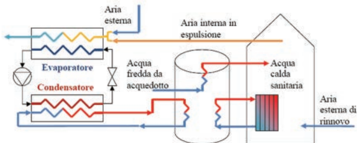
Fig. 23 - Schema di principio di una EAH aria-acqua per il riscaldamento ambientale e la produzione di acqua calda ad uso igienico sanitario
