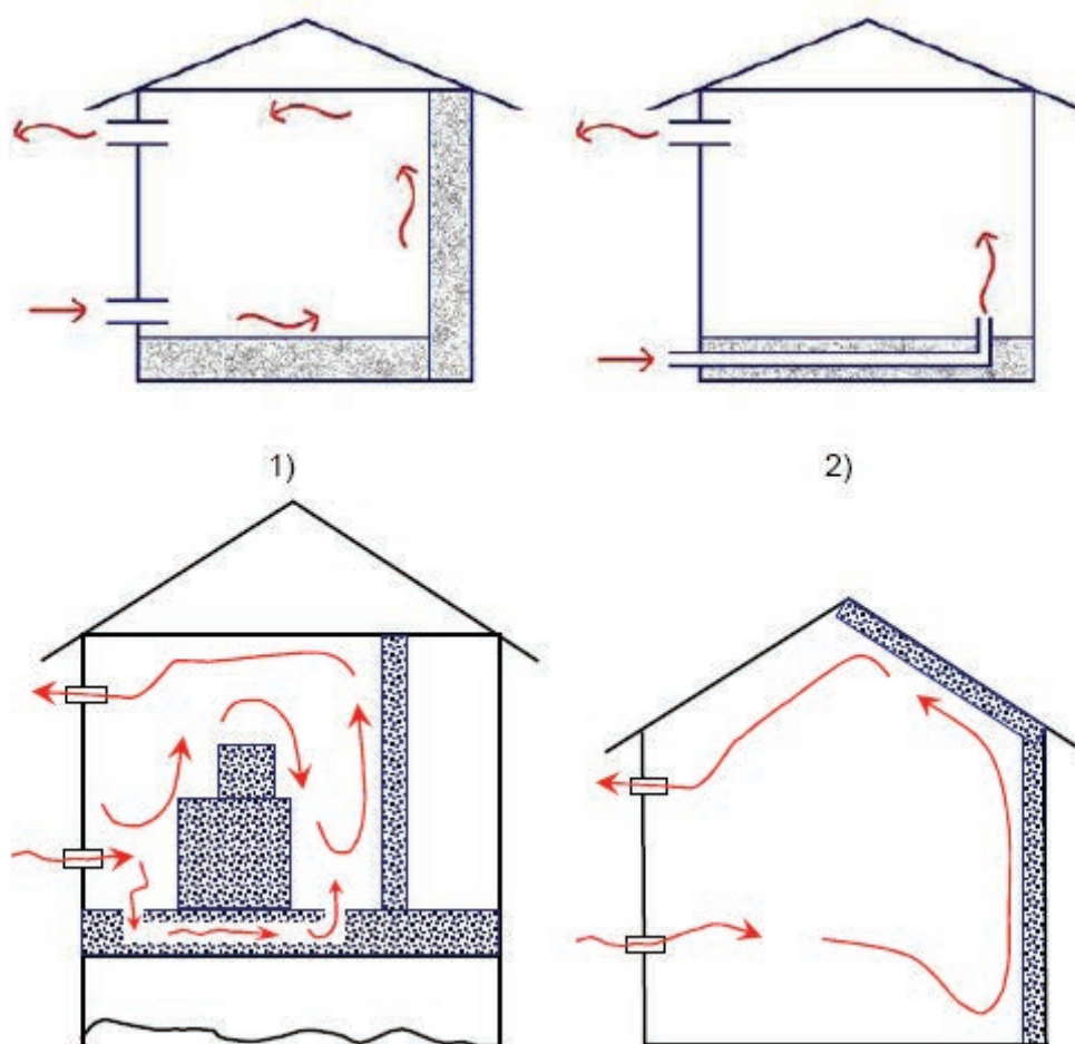
Fig. 9 – Principi di funzionamento TMA: 1) TMA – SA: l'attivazione coinvolge solo la superficie dell'elemento; 2) TMA – CA: l'attivazione coinvolge l'intera struttura dell'elemento; 3) massa termica esterna; 4) massa termica interna.
