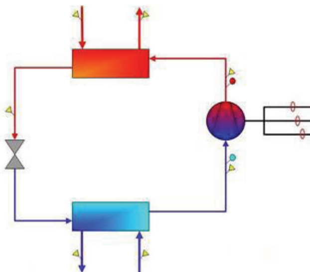
Fig. 20 - Rappresentazione schematica di un circuito a pompa di calore con i punti di misura
