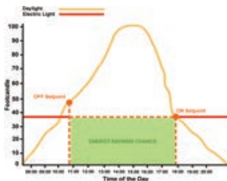
Fig. 17 - Schema di funzionamento di un sistema di controllo di daylighting del tipo on/off
