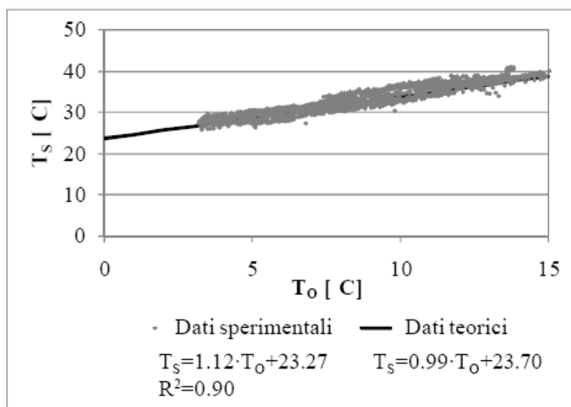
Fig. 26 - Confronto tra i dati teorici ed i dati sperimentali relativi all'andamento della temperatura di immissione ( T_s ) della EAHP in funzione della temperatura dell'aria esterna ( T_o ) in condizioni di funzionamento standard
