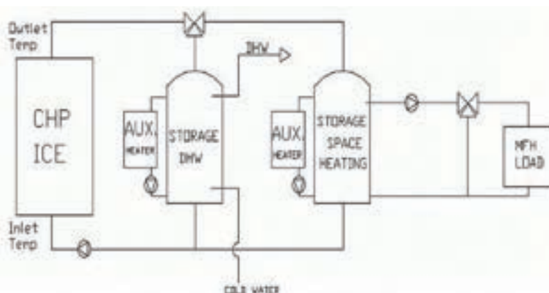
Fig. 1 – Schema dell'impianto di cogenerazione simulato
