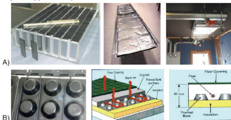
Fig. 12 - Esempio di applicazione dei PCM – A) Accumulo energetico basato sui PCM e sugli scambiatori di calore (sulla sinistra: ZAE-Bayern). B) PCM incorporate nel pavimento
