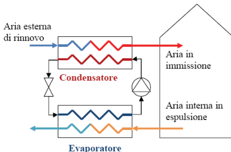
Fig. 22 - Schema di principio di una EAHP a tutt'aria esterna per il rinnovo d'aria in ambiente (funzionamento in riscaldamento)
