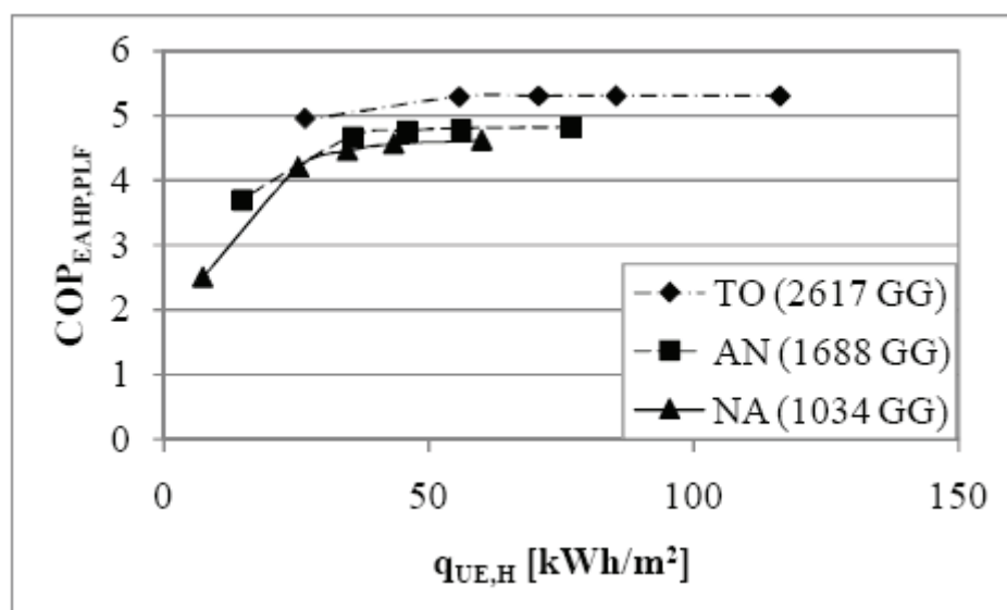
Fig. 29 - Andamento del COP della EAHP con presa in considerazione della riduzione di efficienza ai carichi parziali in funzione del fabbisogno di energia termica utile per tre diverse località
