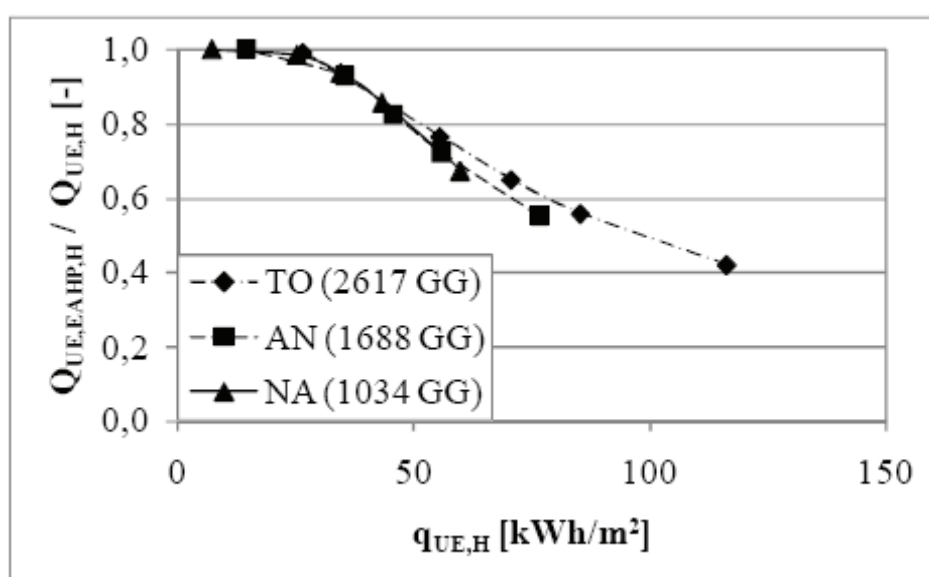
Fig. 27 - Fattore di copertura dell'energia termica utile ad opera della EAHP in funzione del fabbisogno di energia termica utile
