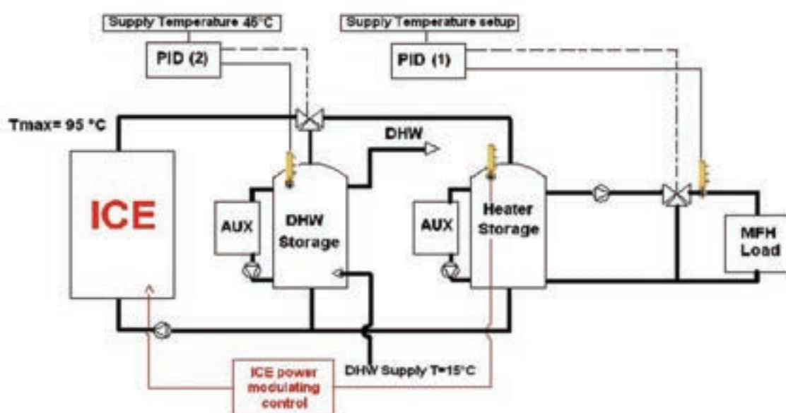
Fig. 2 – Schema di funzionamento del sistema di controllo
