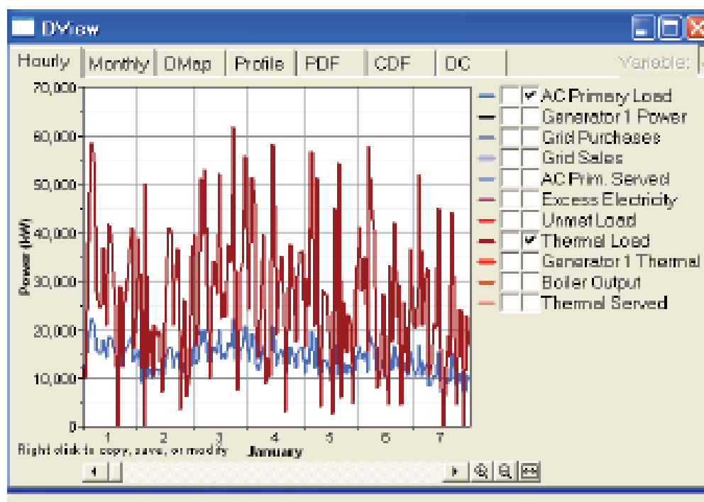
Fig. 33 - Profilo orario della domanda termica ed elettrica per il mese di gennaio
