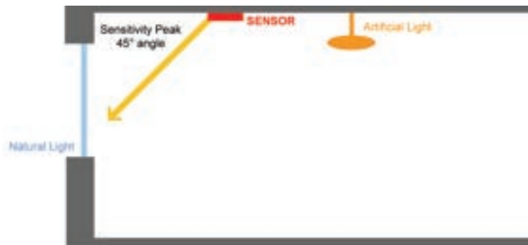
Fig. 15 - Esempio di installazione di un sistema di controllo di daylighting a loop aperto.
