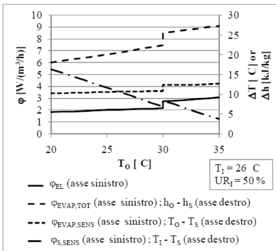
Fig. 25 - Potenza elettrica assorbita dal compressore ( \phi_{EL} ), potenza termica sensibile sottratta all'ambiente dall'aria in immissione ( \phi_{S,SENS} ), potenza termica sottratta all'aria dalla batteria evaporante, nella quota totale ( \phi_{EVAP,TOT} ) e solamente sensibile ( \phi_{EVAP,SENS} ) per unità di portata d'aria trattata in funzione della temperatura esterna. Differenza di temperatura ( T_o - T_s ) e di entalpia ( h_o - h_s ) tra l'aria in immissione e l'aria esterna e differenza di temperatura tra l'aria interna e l'aria in immissione ( T_i - T_s ) in funzione della temperatura dell'aria esterna
