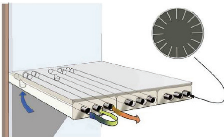
Fig. 8 - Principio di funzionamento dell'attivazione termica della massa
