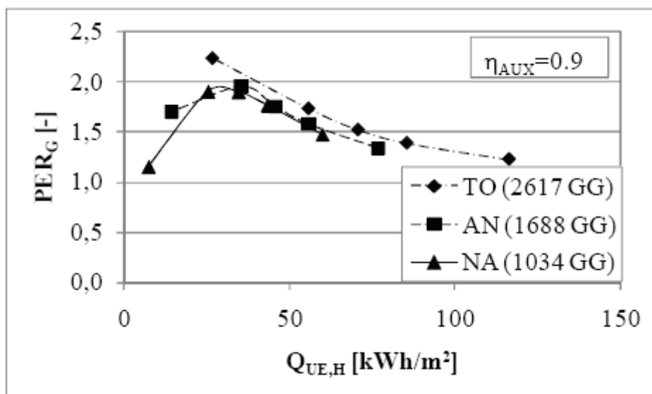
Fig. 30 - Andamento del rapporto di energia primaria globale per edifici caratterizzati da diverso fabbisogno di energia termica utile e per tre diverse località
