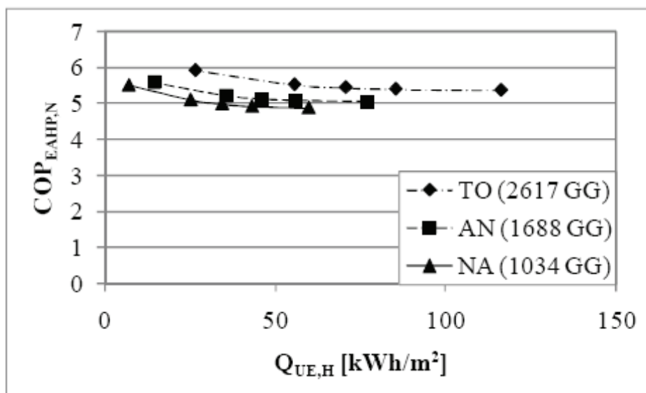
Fig. 28 - Andamento del valore nominale (al 100 % del carico) del COP della EAHP in funzione del fabbisogno di energia termica utile per tre diverse località
