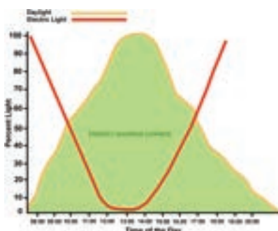
Fig. 18 - Schema di funzionamento di un sistema di controllo di daylighting con dimmer.
