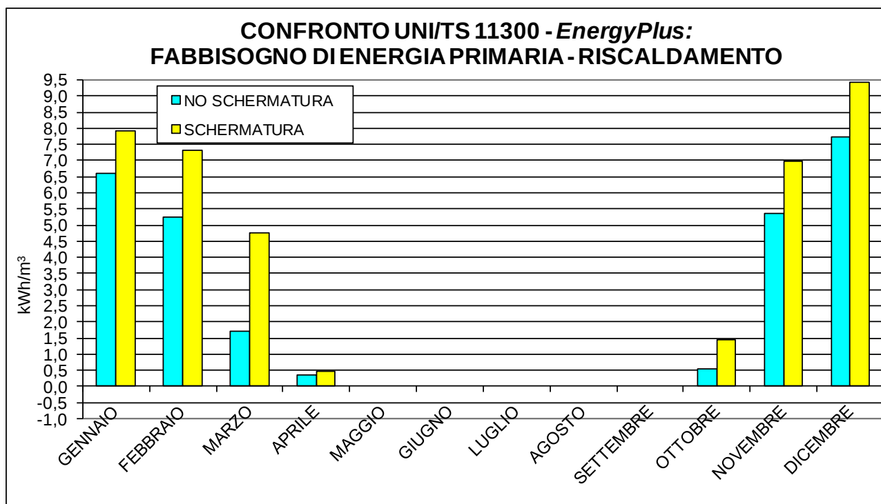
Figura 3.2.35 – Differenza tra il fabbisogno di energia primaria per il riscaldamento, in presenza ed in assenza di schermature solari, calcolato rispettivamente applicando il modello semplificato (UNI/TS 11300) e dettagliato ( EnergyPlus ): città di Torino.
