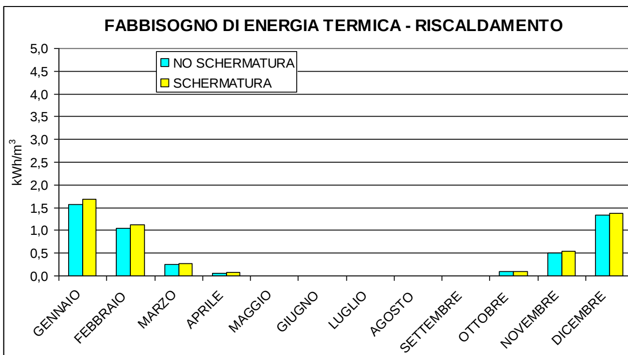
Figura 3.2.12 – Fabbisogno di energia termica per il riscaldamento, in presenza ed in assenza di schermature solari, per la città di Torino.
