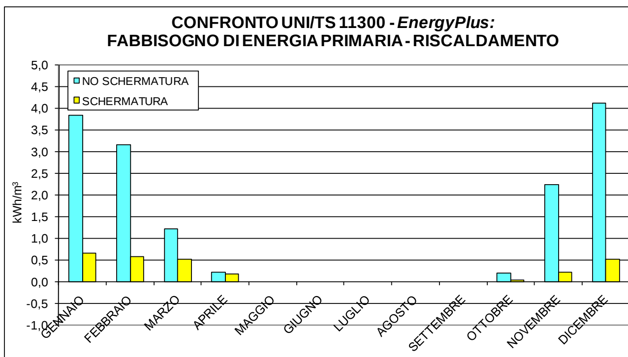
Figura 3.2.37 – Differenza tra il fabbisogno di energia primaria per il riscaldamento, in presenza ed in assenza di schermature solari, calcolato rispettivamente applicando il modello semplificato (UNI/TS 11300) e dettagliato ( EnergyPlus ): città di Palermo.
