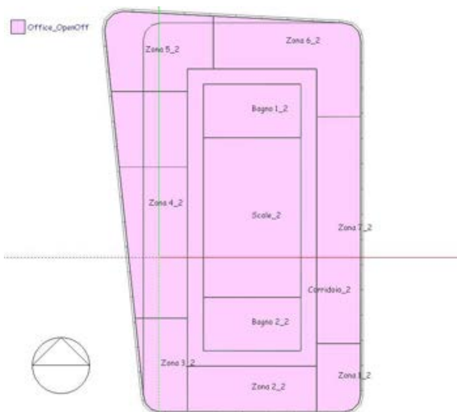
Figura 3.2.4 – Suddivisione in zone termiche della tipologia B di piano tipo.
