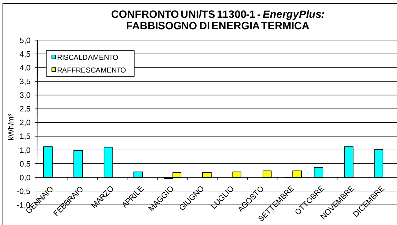
Figura 3.3.14 - Differenza tra il fabbisogno di energia termica per la climatizzazione calcolato rispettivamente applicando il modello semplificato (UNI/TS 11300-1) e dettagliato ( EnergyPlus ): città di Torino.
