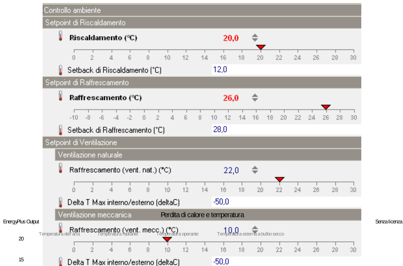
Figura 3.3.8 – Dati in ingresso alla simulazione: ventilazione meccanica, set-point.
