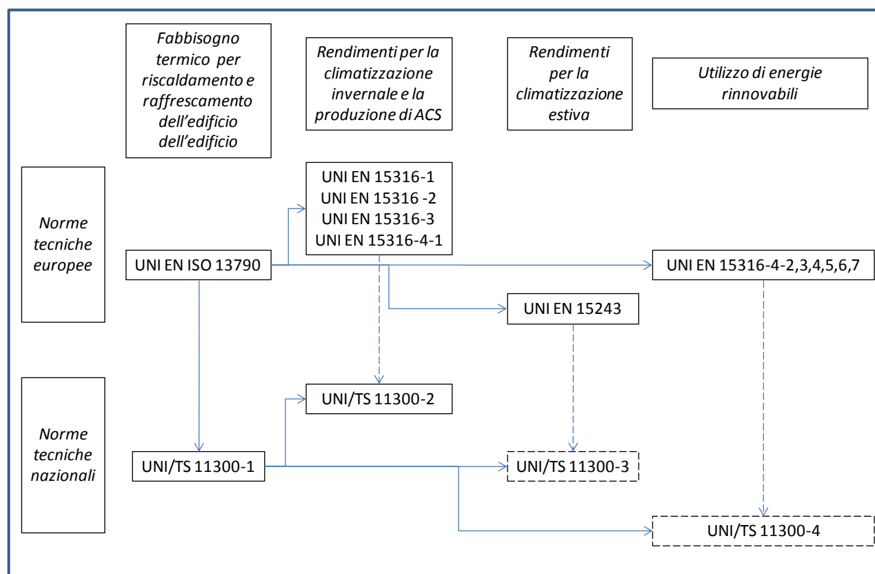
Figura 2.2 - Relazione tra la normativa tecnica europea e quella italiana per il calcolo del fabbisogno di energia per la climatizzazione degli edifici.
