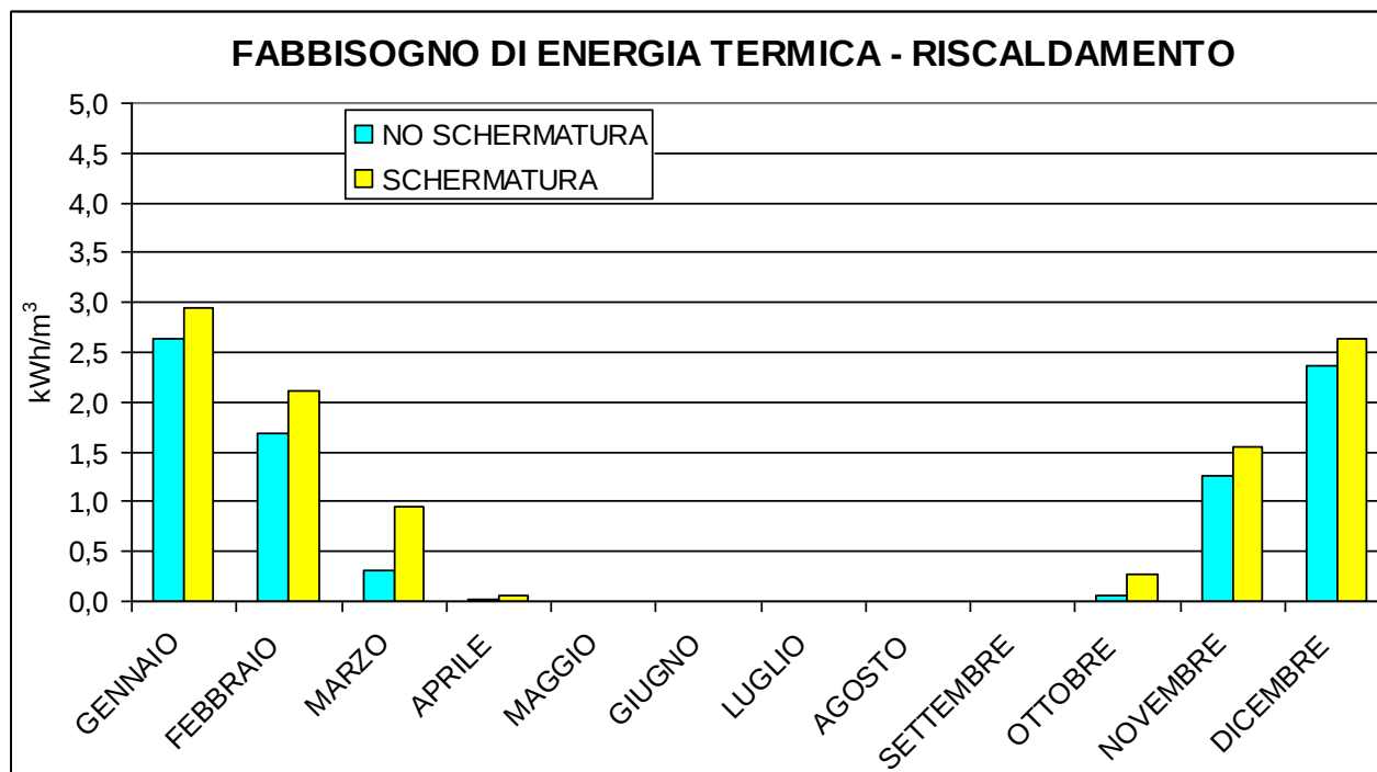
Figura 3.2.23 – Fabbisogno di energia termica per il riscaldamento, in presenza ed in assenza di schermature solari, per la città di Torino.
