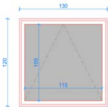
Finestra 130x120
