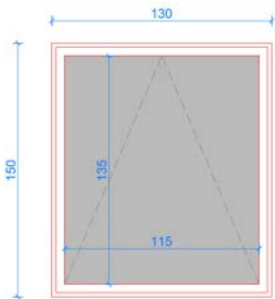
Porta-finestra 150x130
