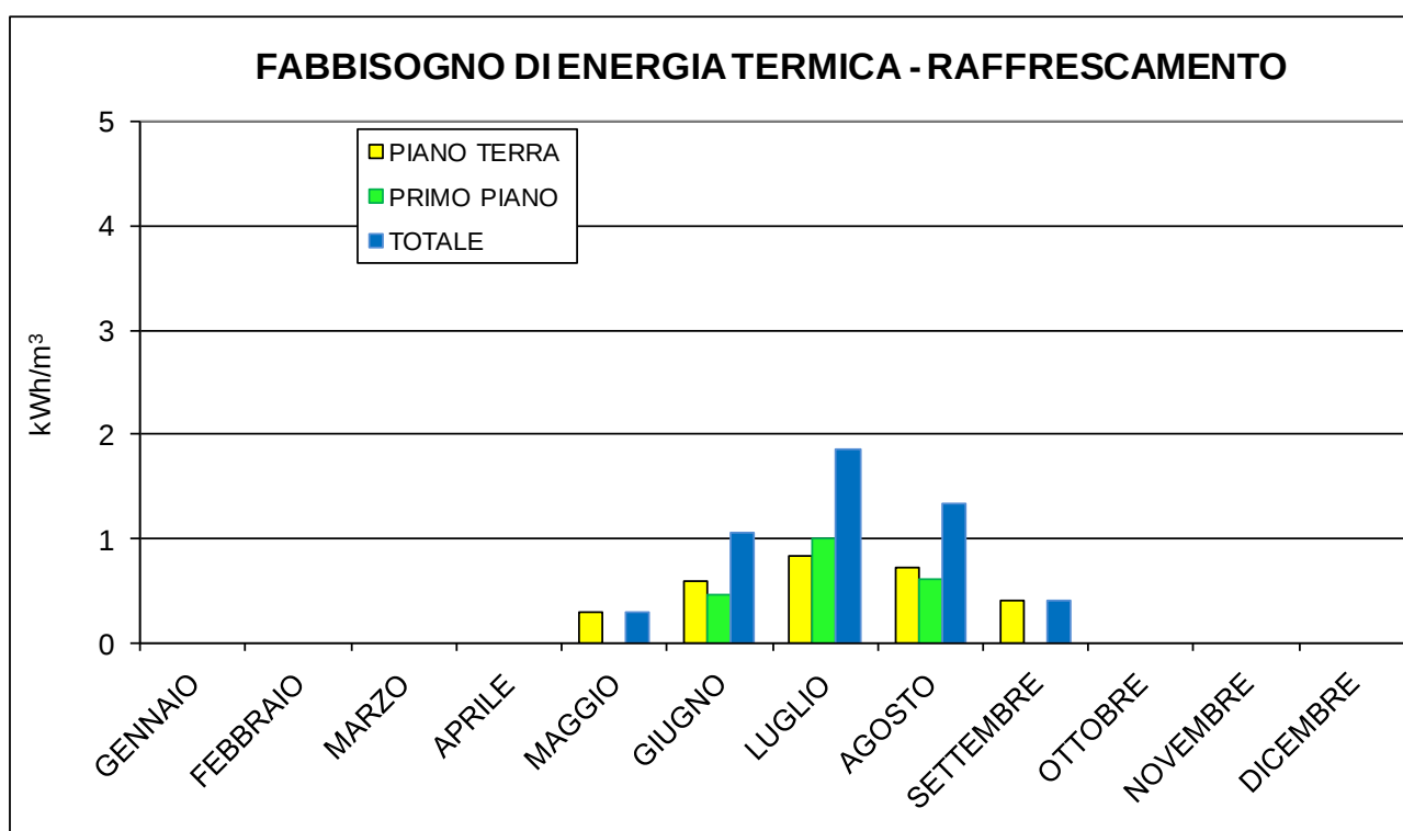
Figura 3.3.13 - Fabbisogno mensile di energia termica per il raffrescamento, in applicazione della UNI/TS 11300-1: città di Torino.
