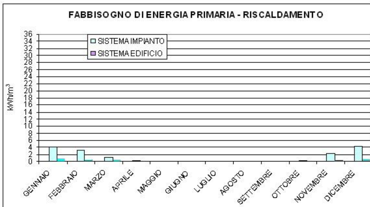
Figura 3.2.29 – Fabbisogno di energia primaria per il riscaldamento, in presenza ed in assenza di schermature solari, per la città di Palermo, in applicazione delle specifiche tecniche UNI/TS.
