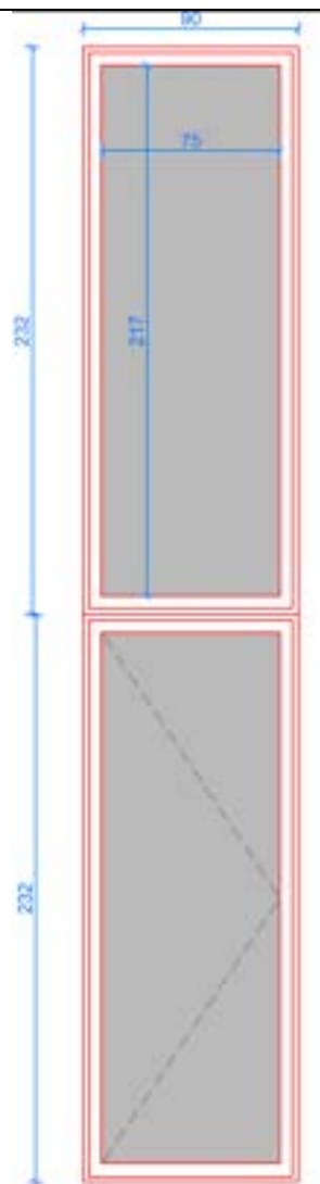
Finestra 464x90
