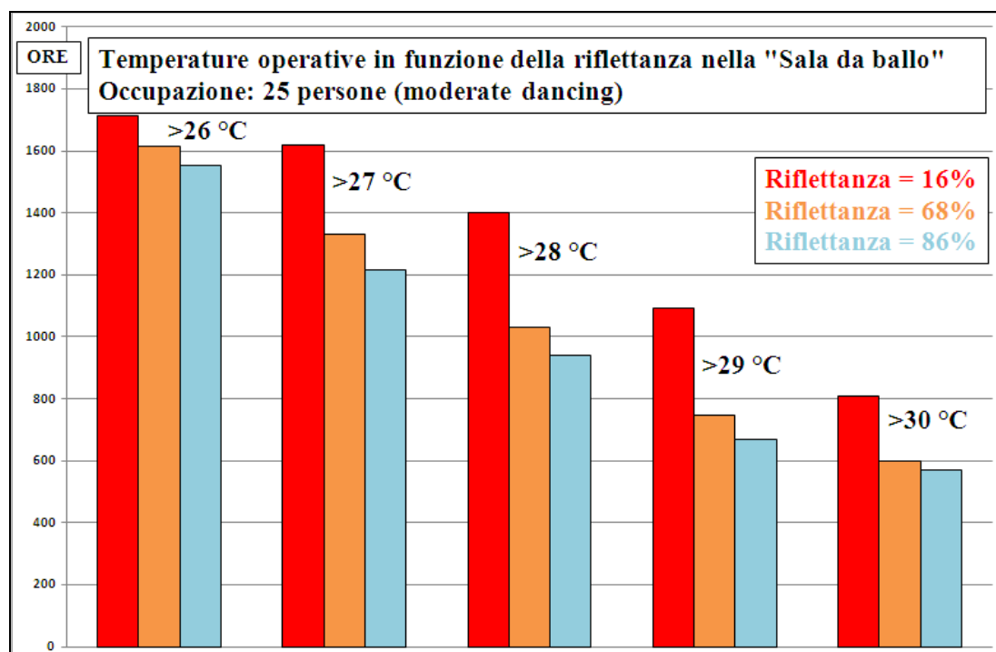
Figura 21: Temperatura operativa, profilo di occupazione 25 persone
