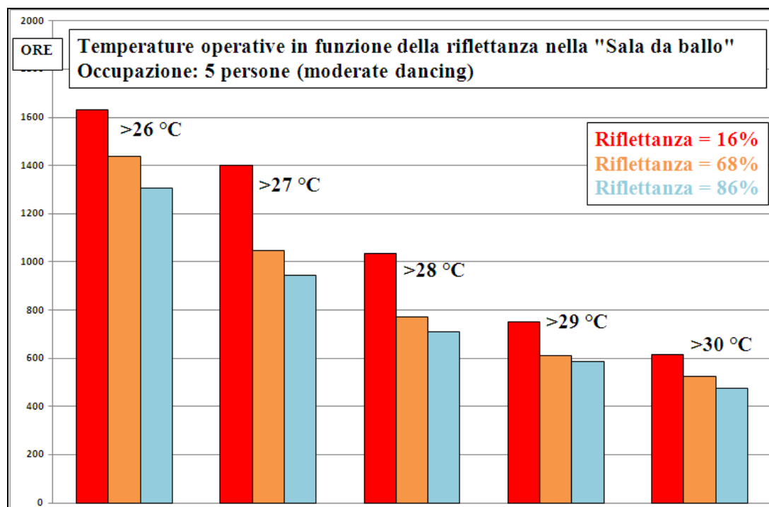
Figura 23: Temperatura operativa, profilo di occupazione 5 persone
