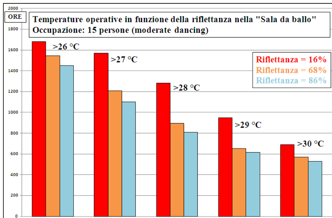
Figura 22: Temperatura operativa, profilo di occupazione 15 persone
