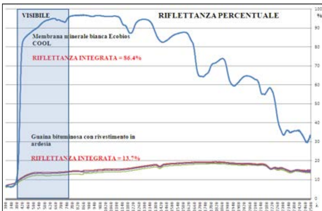
Figura 3: Confronto riflettanze della membrana Ecobios Clima e della guaina originaria montata sul tetto del Centro Sociale Culturale "Vasca Navale"
