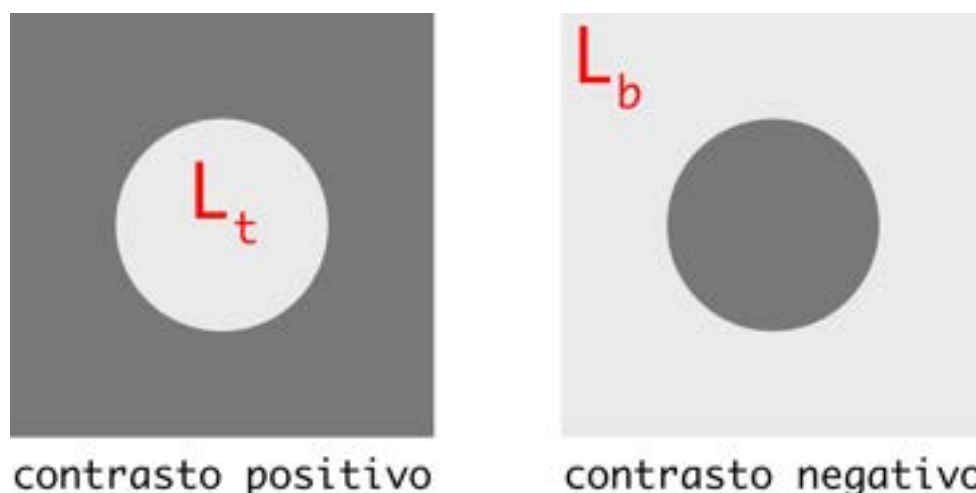
Figura 2 Condizioni di visione di un oggetto: il contrasto è positivo se la luminanza L_t dell'oggetto è superiore a quella L_b dello sfondo, il contrasto è negativo nella situazione opposta.
