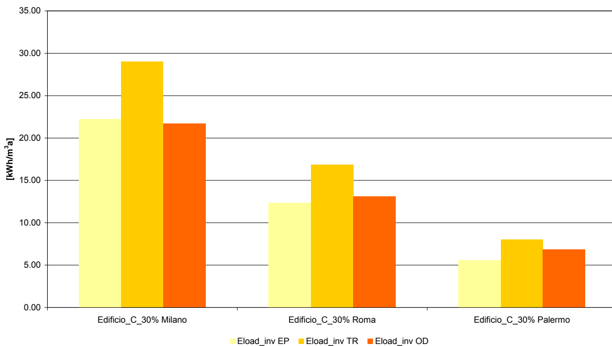
Figura 33 – Confronto tra i fabbisogni energetici invernali al m³ degli edifici C 30% simulati per Milano, Roma, Palermo
