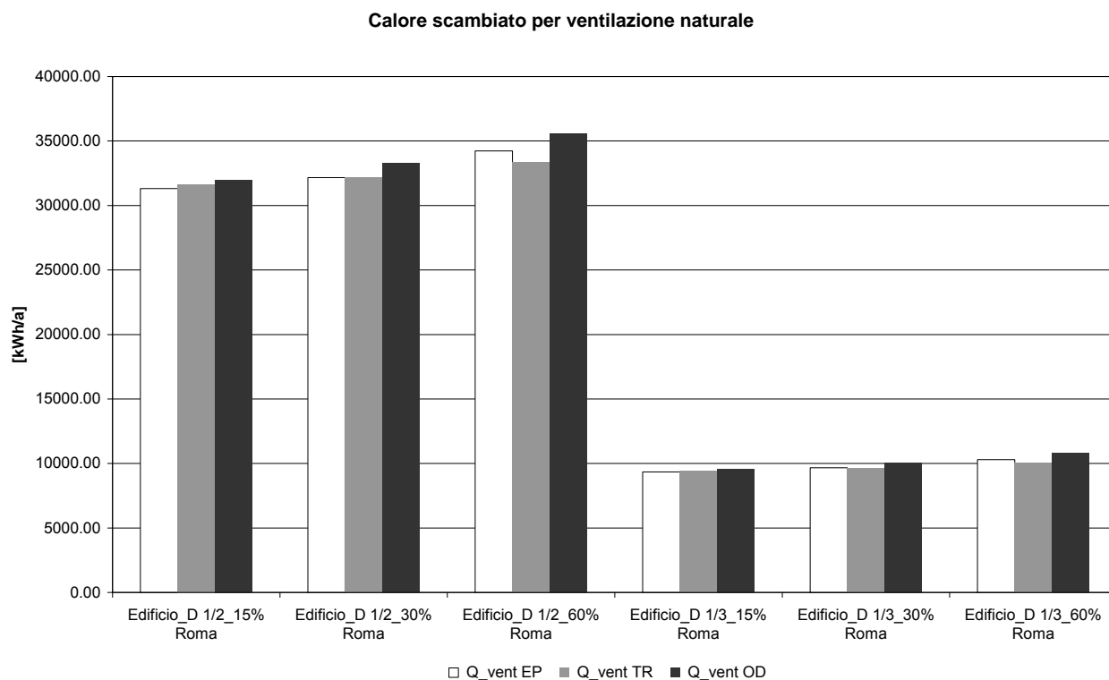
Figura 43 – Confronto tra il calore scambiato per ventilazione naturale negli edifici D 1/2 e D 1/3 con i 3 tipi differenti di vetrate simulate per Roma
