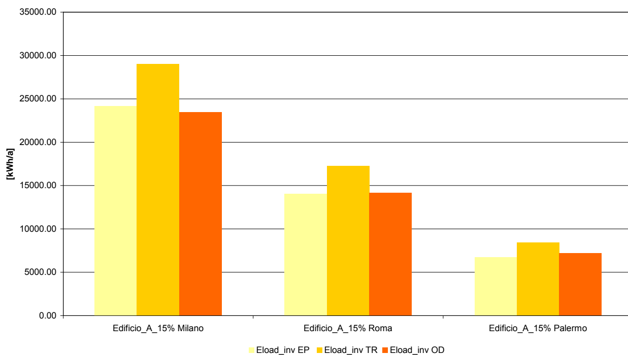
Figura 11 – Confronto tra i fabbisogni energetici invernali degli edifici A 15% simulati per Milano, Roma, Palermo
