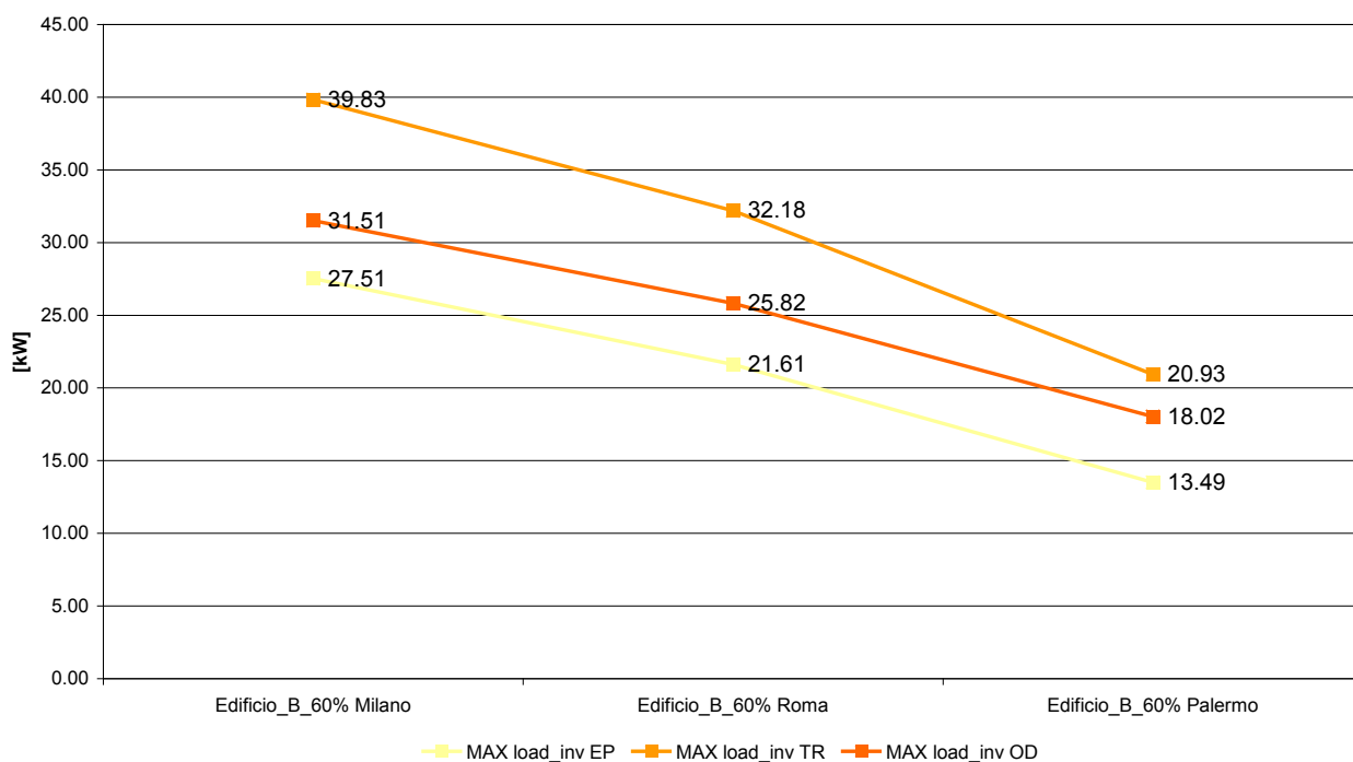
Figura 21 – Confronto tra le potenze di picco invernali degli edifici B 60% simulati per Milano, Roma, Palermo
