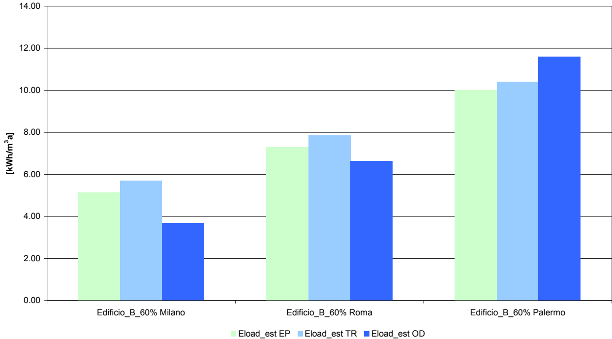
Figura 25 – Confronto tra i fabbisogni energetici estivi al m 3 degli edifici B 60% simulati per Milano, Roma, Palermo
