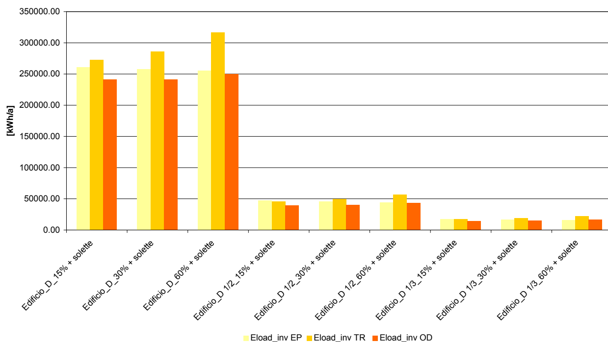
Figura 46 – Confronto tra i fabbisogni energetici invernali degli edifici D, D 1/2 e D 1/3 con massa interna e con i 3 tipi differenti di vetrate simulate per Roma
