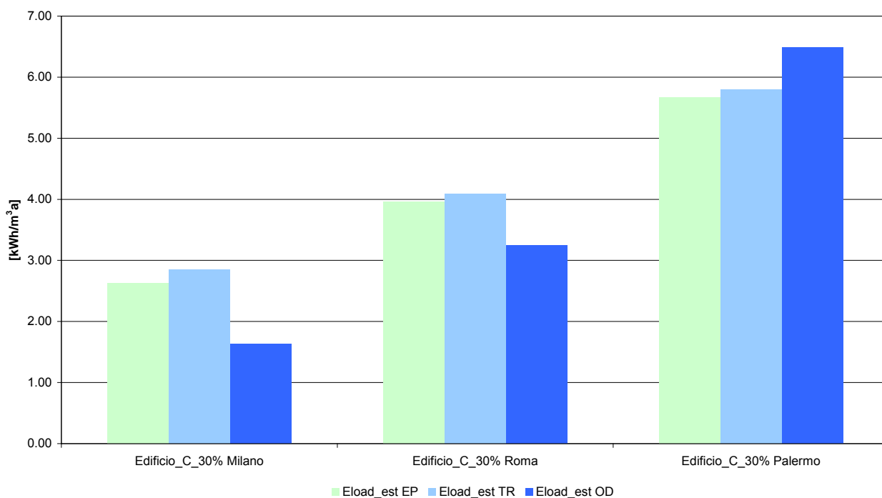
Figura 34 – Confronto tra i fabbisogni energetici estivi al m³ degli edifici C 30% simulati per Milano, Roma, Palermo
