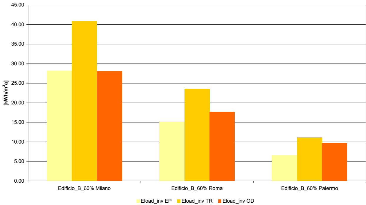
Figura 24 – Confronto tra i fabbisogni energetici invernali al m 3 degli edifici B 60% simulati per Milano, Roma, Palermo
