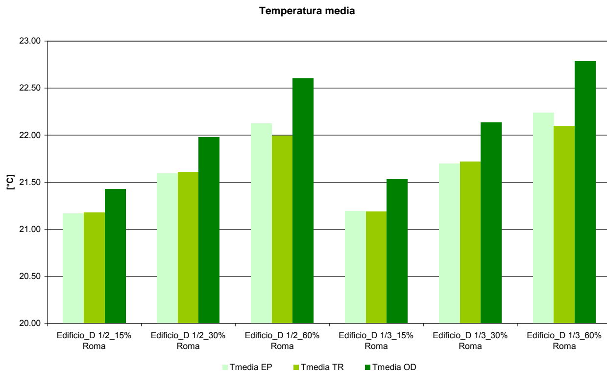
Figura 42 – Confronto tra la temperatura media interna negli edifici D 1/2 e D 1/3 con i 3 tipi differenti di vetrate simulate per Roma
