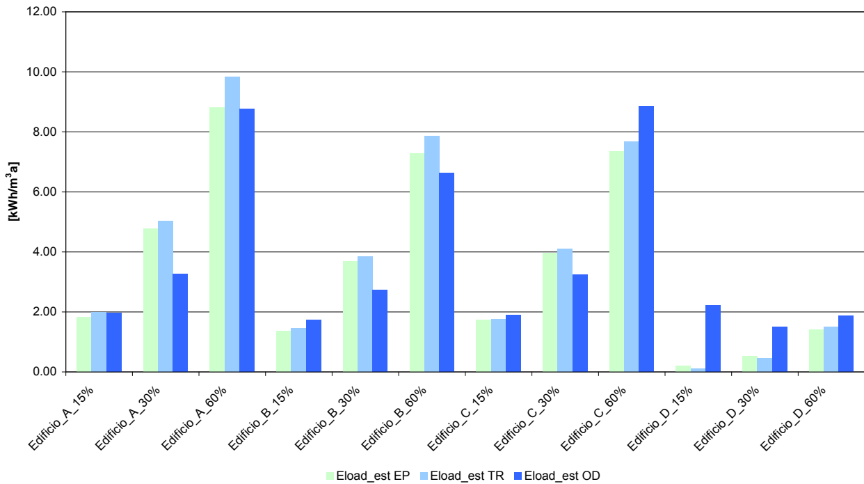
Figura 7 – Confronto tra i fabbisogni energetici estivi al m 3 delle 12 tipologie di edifici simulate per Roma
