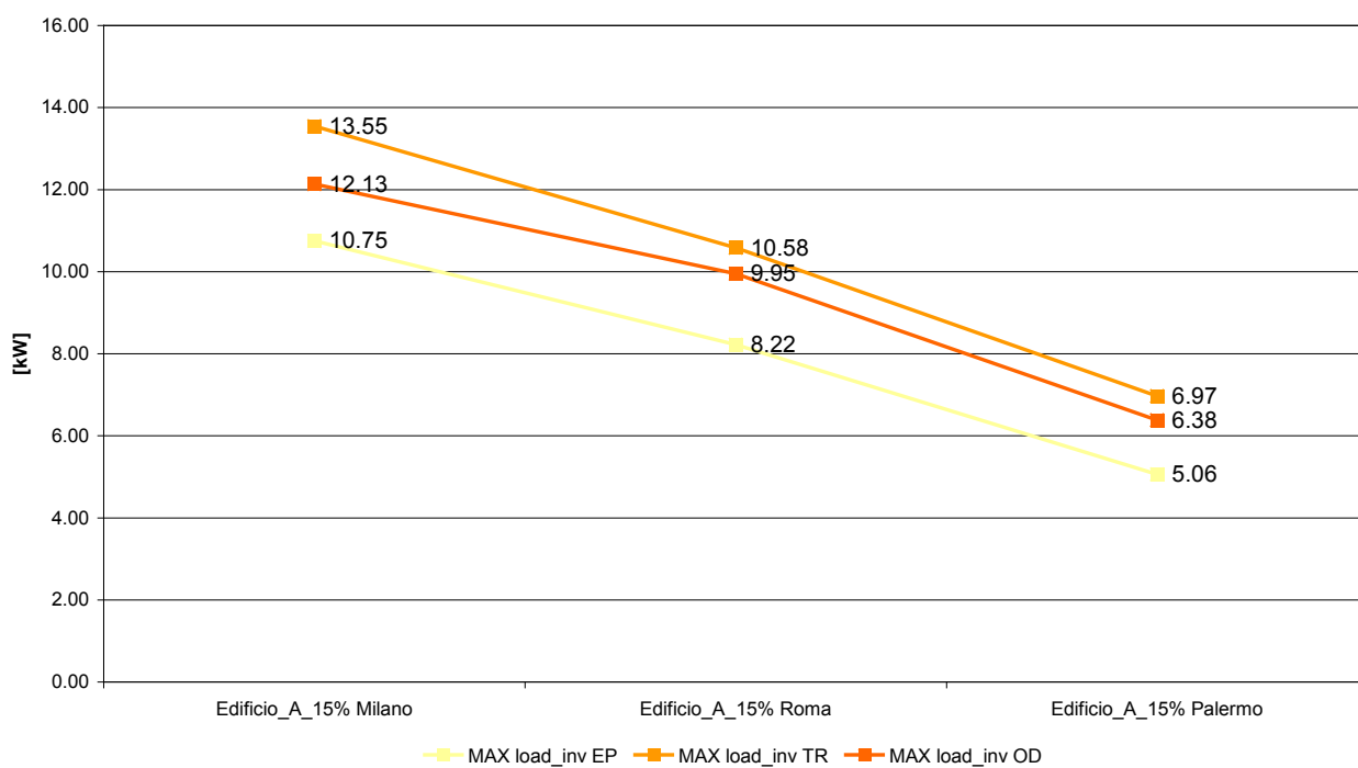
Figura 12 – Confronto tra le potenze di picco invernali degli edifici A 15% simulati per Milano, Roma, Palermo
