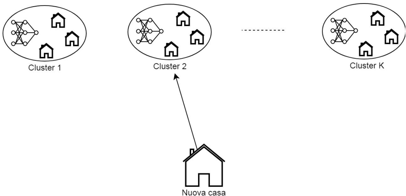
Figura 30: strategia di clustering per la disaggregazione del consumo elettrico
