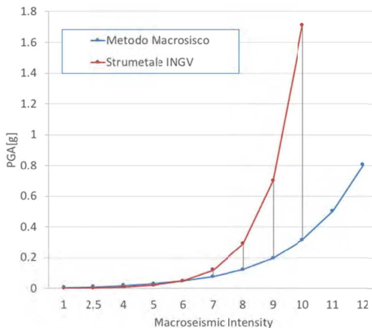
Figura 16. Correlazione tra Intensità e PGA: assunta dal metodo macrosismico (in rosso); assunta per ottenere l'intensità macrosismica strumentale (utilizzata nella mappa in Figura 1a).
