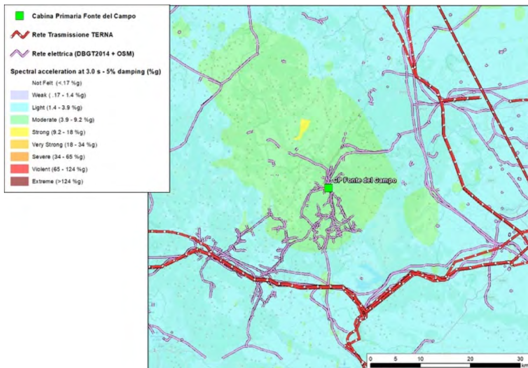
Figura 4. Mappe di scuotimento in PSA03 (T=3s, smorzamento 5%) per il Terremoto di Amatrice (Italia Centrale) del 24/08/2016 da [2] e approssimata localizzazione di componenti della rete elettrica.
