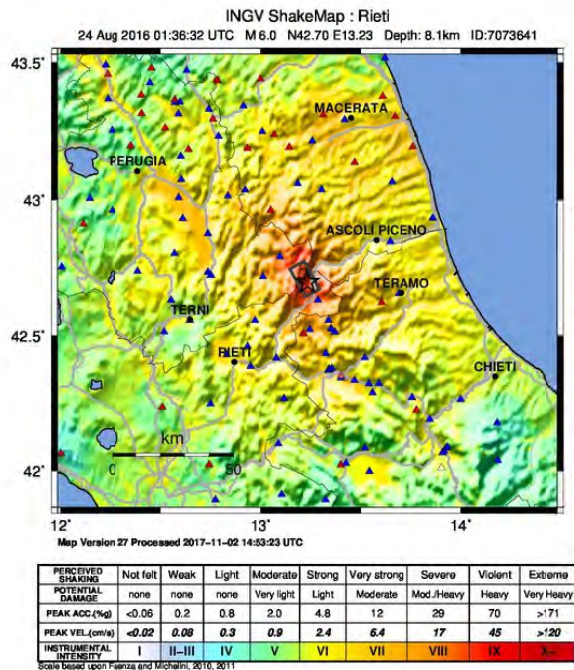
Figura 1. Zona colpita dal terremoto di Amatrice: a) mappa dello scuotimento del terremoto [2]; b) localizzazione degli impianti AT e MT interessati dall'evento sismico (estratte da[4]).
