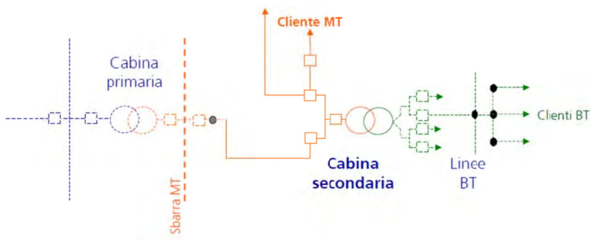
Figura 10. Schema base di una rete di MT e BT
