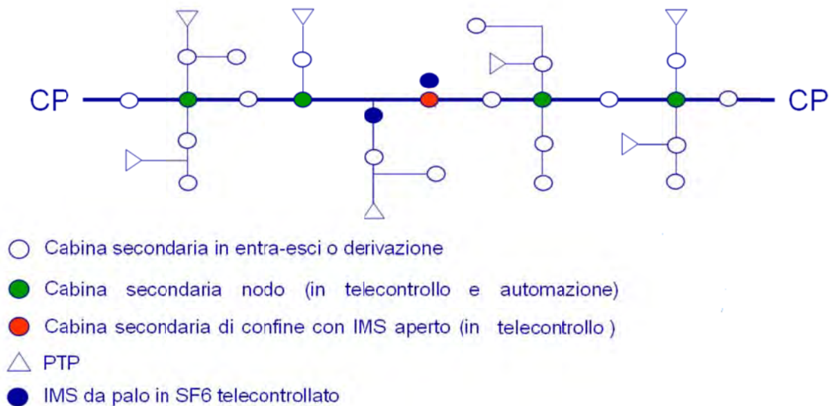
Figura 12. Schemi linea MT: a) schema Dorsale di MT (dove CP sta per Cabina Primaria, PTP Posto di Trasformazione su Palo; IMS interruttore di manovra sezionatore)
