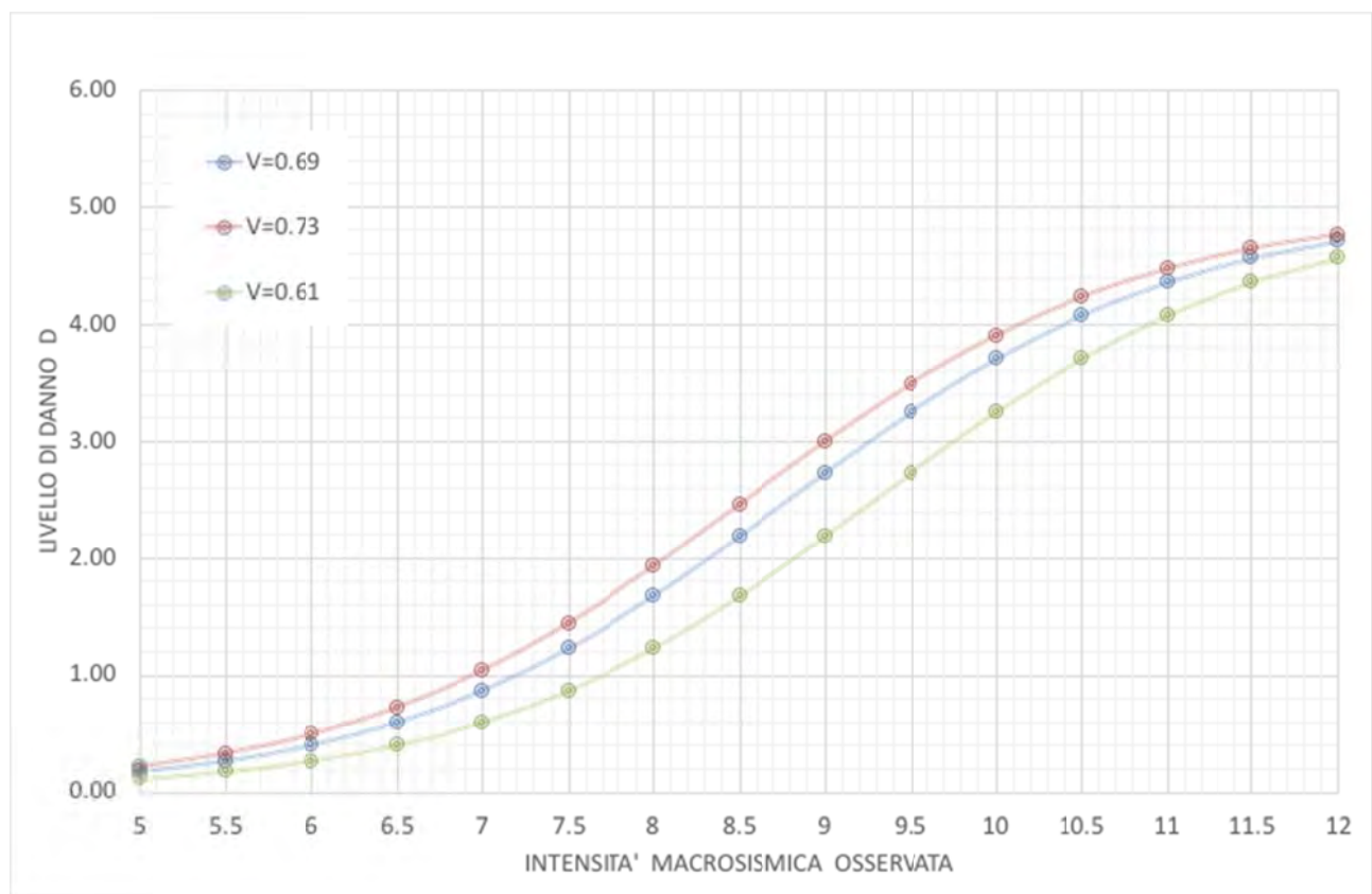
Figura 15. Curve di vulnerabilità secondo il metodo macrosismico [7] per diversi valori dell'indice di vulnerabilità V
