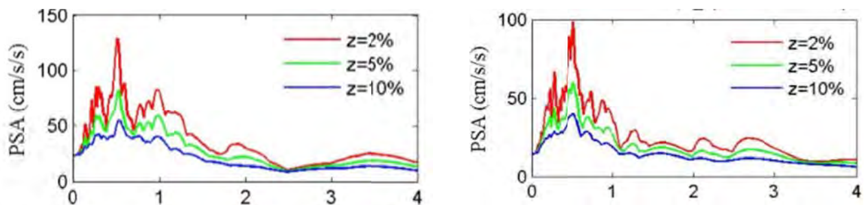
Figura 2. Stazione ANT (Rep=34.3km): a) componente Est-Ovest; b) componente Nord-Sud (da [3]).
