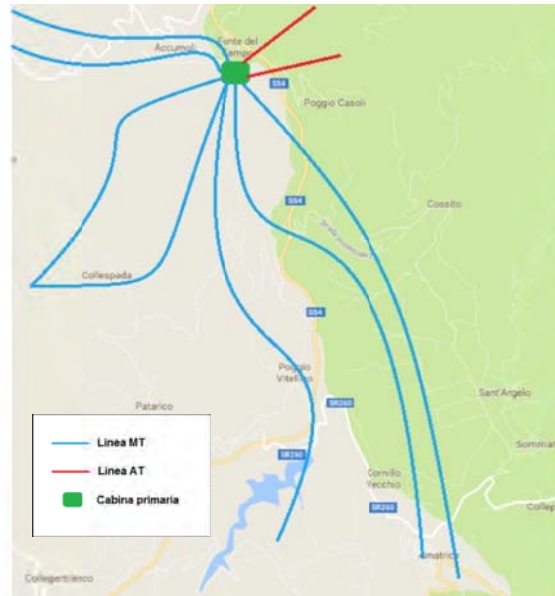
Figura 1. Zona colpita dal terremoto di Amatrice: a) mappa dello scuotimento del terremoto [2]; b) localizzazione degli impianti AT e MT interessati dall'evento sismico (estratte da[4]).
