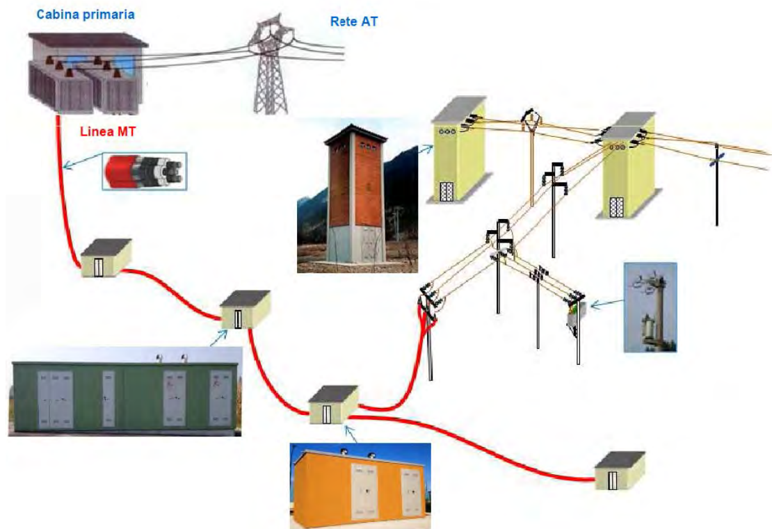
Figura 11. Diverse tipologie di cabine secondarie riconoscibili in una linea MT
