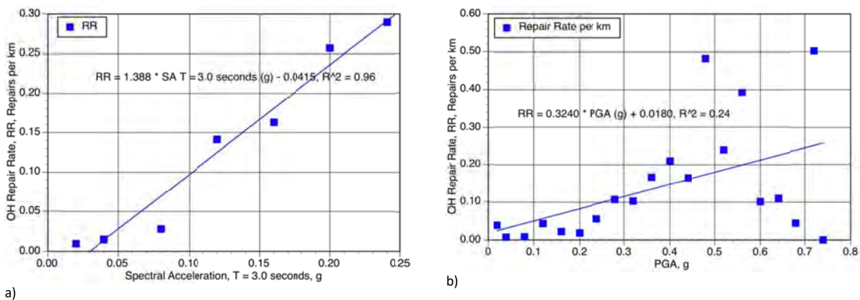
Figura 17. Modelli assunti in CIPCast per la previsione del danno sisma-indotto alle linee aeree: in funzione di PSA03; b) in funzione di PGA[g] (da [15])
