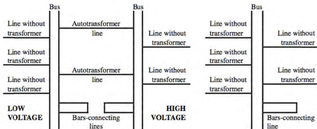
Figura 14. Layout generici di macro-componenti per una sottostazione di trasformazione (a sinistra) e una sottostazione di sola distribuzione (a destra) [7][14]
