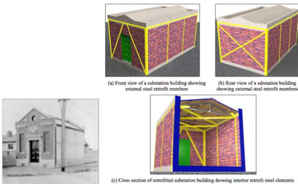
Figura 19. Sottostazioni per la trasformazione da MT a BT gestite da Orion a Christchurch in Nuova Zelanda: a) esempio di sottostazione considerata edificio storico; b) schema del rinforzo sismico adottato per 150 sottostazioni [19]
