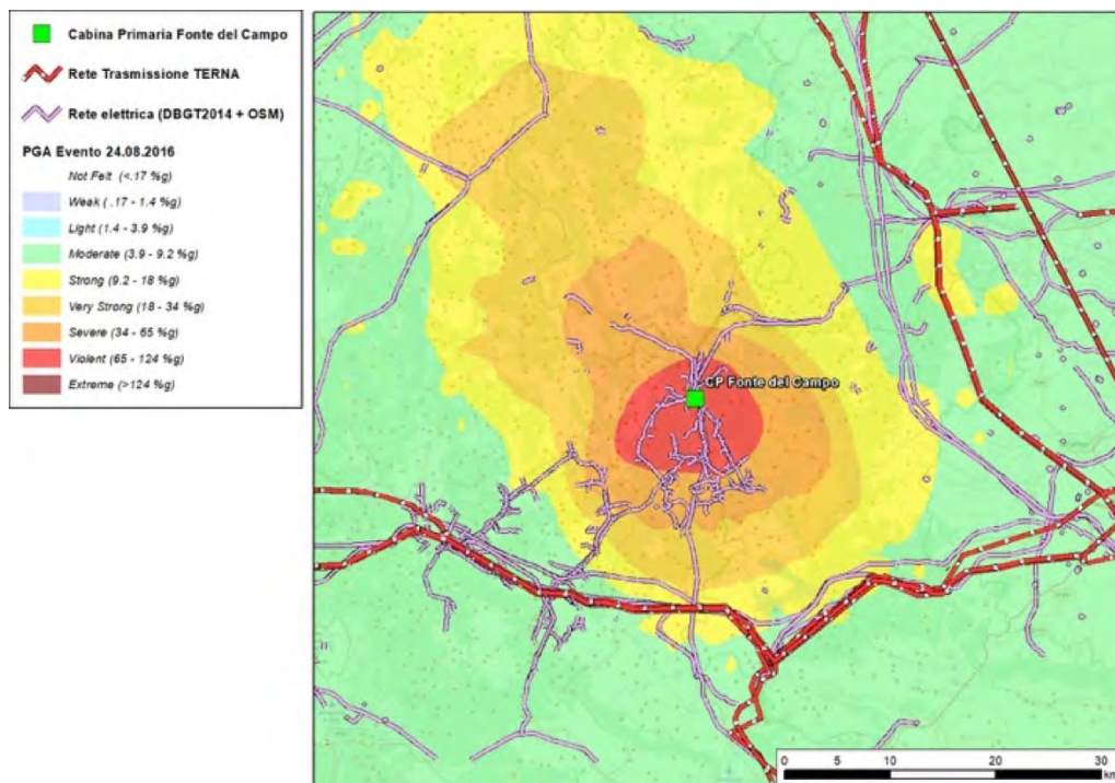
Figura 3. Mappe di scuotimento accelerazione di picco PGA [%g] per il Terremoto di Amatrice (Italia Centrale) del 24/08/2016 da [2] e approssimata localizzazione di componenti della rete elettrica
