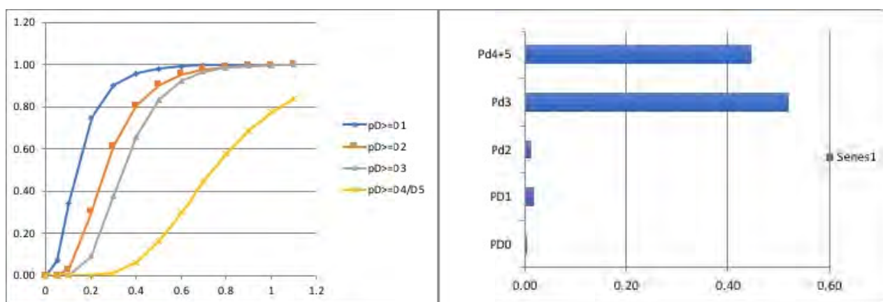
Figura 13. Curve di fragilità per sottostazioni elettriche, secondo HAZUS[8]: a) Probabilità di superamento (probabilità cumulata) dei diversi livelli di danno in funzione dello scuotimento del suolo in termini di PGA[g]; b) Distribuzione di Probabilità di Danno per PGA=0.7
