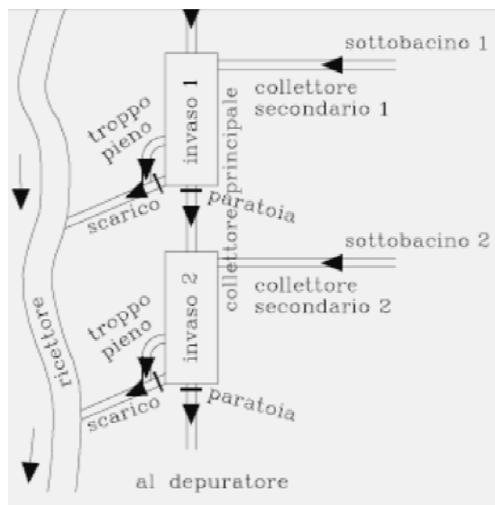
Figura 6.7: schemi relativi al posizionamento degli invasi sulla rete, in serie (immagine a sinistra) e con schema a "Y" (immagine a destra) [A. Campisano e U. Sanfilippo "Controllo in tempo reale dei sistemi di fognatura"]
