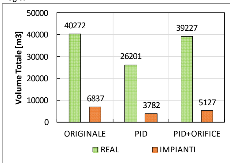
Figura 4.17: grafico relativo al volume totale inviato al ricettore per ogni rete analizzata ponendo a confronto lo scenario reale rispetto a quello con l'installazione degli impianti per il recupero e il riuso delle acque meteoriche
