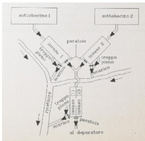
Figura 6.7: schemi relativi al posizionamento degli invasi sulla rete, in serie (immagine a sinistra) e con schema a "Y" (immagine a destra) [A. Campisano e U. Sanfilippo "Controllo in tempo reale dei sistemi di fognatura"]
