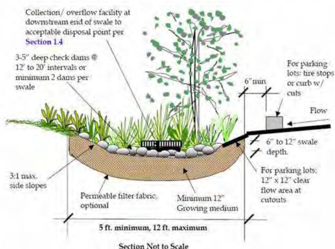
Figura 2.17: Esempio di un canale inerbito [http://www.ci.sandy.or.us]
