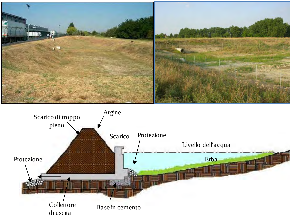
Figura 2.8: esempi di bacini asciutti [Maglionico, 2004] e relativa sezione schematica [NVPDC, 2002]
