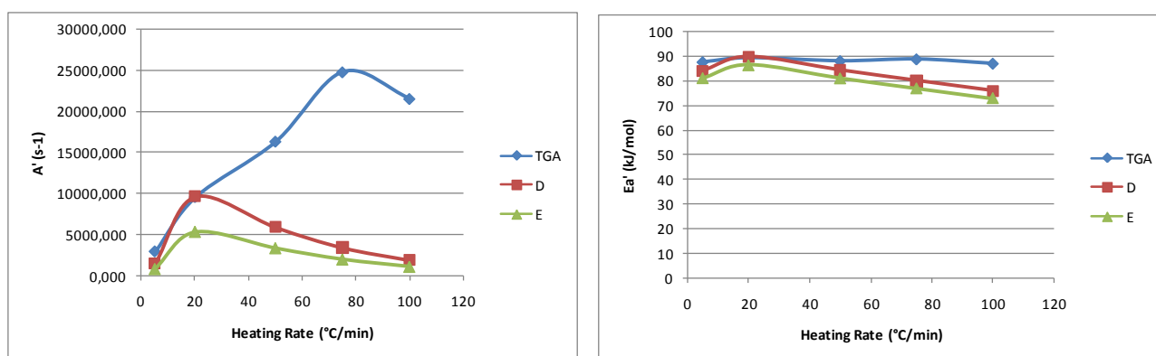
Fig 16.- Fattore pre-esponenziale (Ao' ( \text{s}^{-1} )) ed energia di attivazione Ea (J/mol) ottenuti con i dati sperimentali (TGA) e simulati (D-E) nell'intervallo di temperatura tra 300 – 450 ^{\circ}\text{C}
