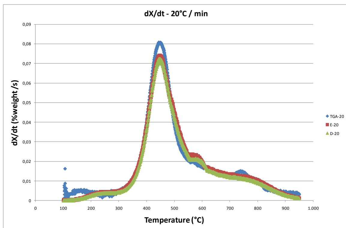
Fig. 8.- Confronto tra le velocità di devolatilizzazione (% peso/s) in funzione della temperatura (°C): dati sperimentali (blu), e simulati con metodo D (rosso) ed E (verde) a 20°C/min
