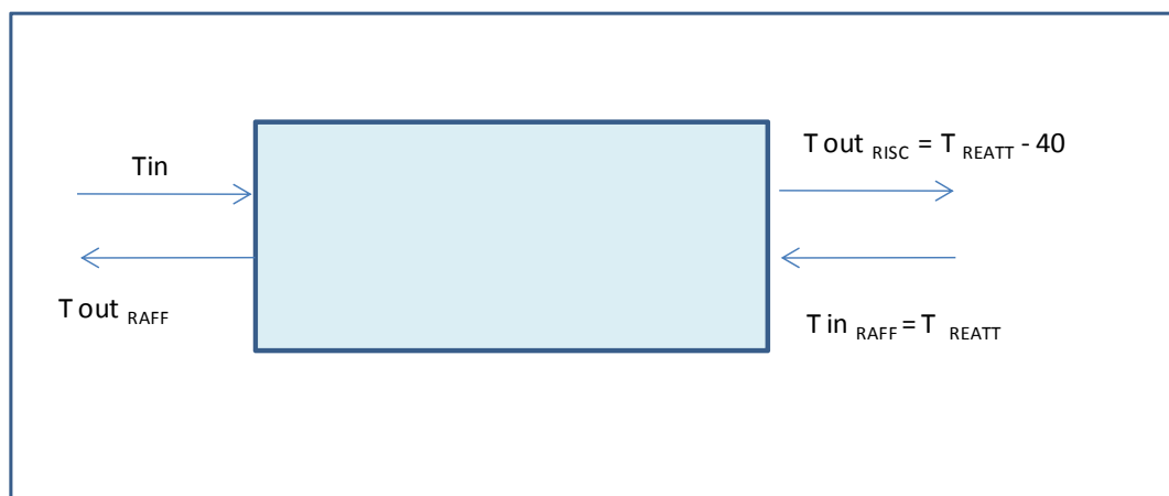
Figura 45. Schema di processo dello scambiatore D (vedi
