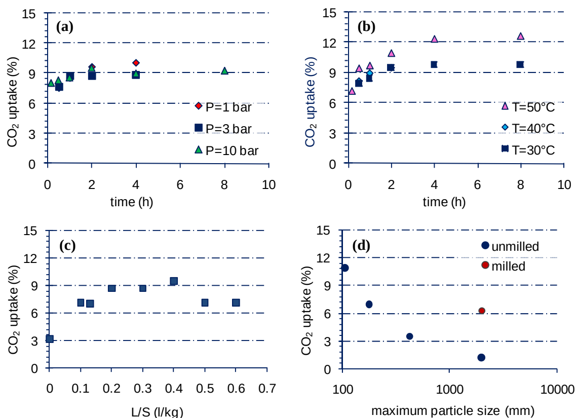
Figura 56. Effetto dei parametri operativi sul sequestro di CO 2 misurato per la miscela: a) effetto della pressione, b) effetto della temperatura c) effetto del rapporto L/S, d) effetto della granulometria
