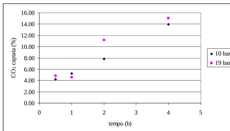
Figura 61. CO 2 sequestrata in fase acquosa a 100°C
