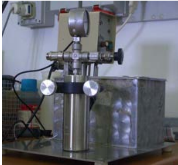
Figura 53. Reattore in acciaio e bagno termostatico utilizzati per le prove di carbonatazione ad umido
