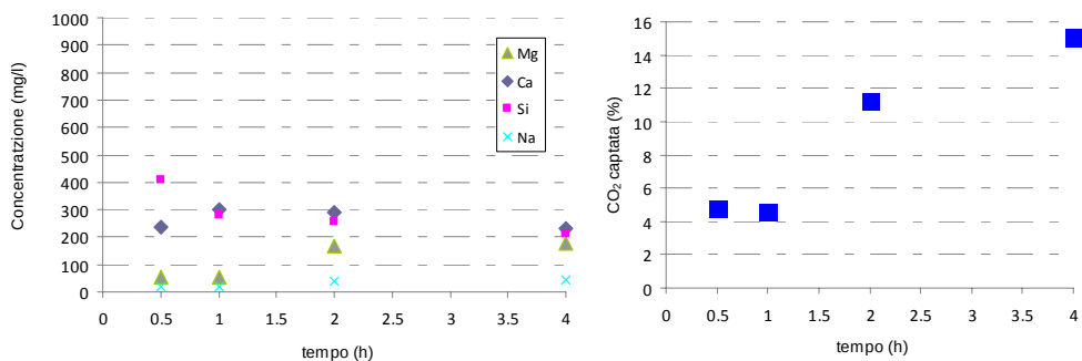
Figura 62. Concentrazione dei macroelementi nella soluzione di processo
