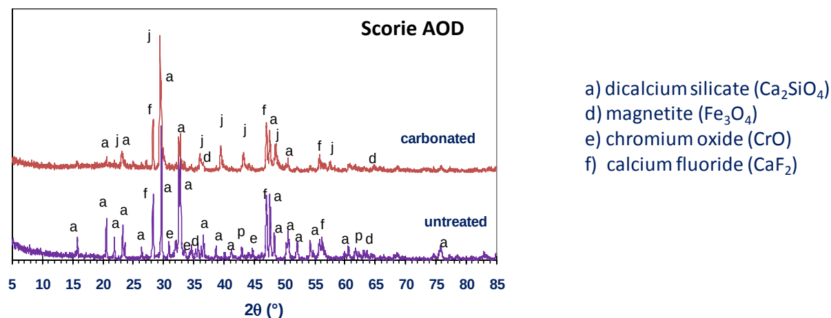
Figura 67. Effetto del trattamento di carbonatazione testato ( L/S=0.4 l/kg; T=50 °C; p=3 bar; t=2 ore) sulla mineralogia delle scorie EAF e AOD
