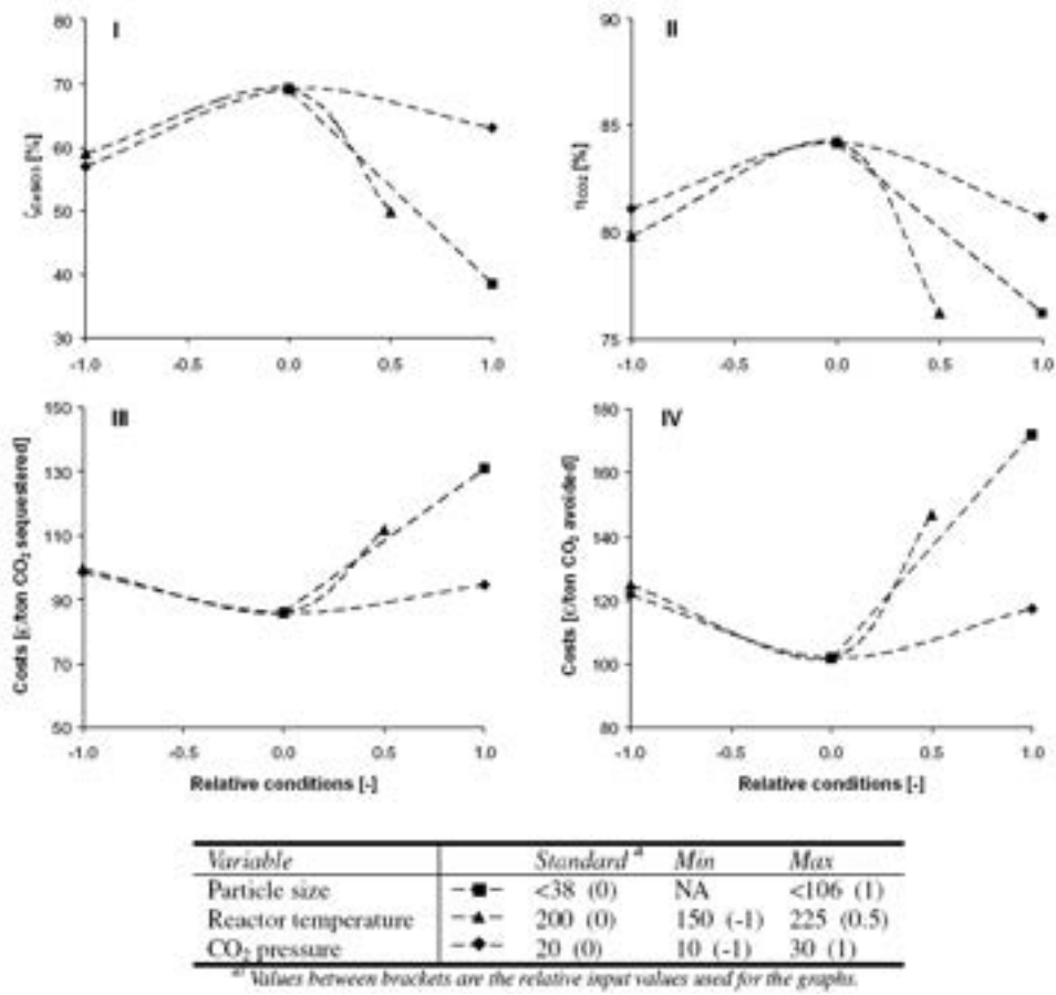
Figura 7: Influenza dei parametri operativi sui risultati di esperimenti di carbonatazione condotti sulla wollastonite (Huijgen et al., 2006b)
