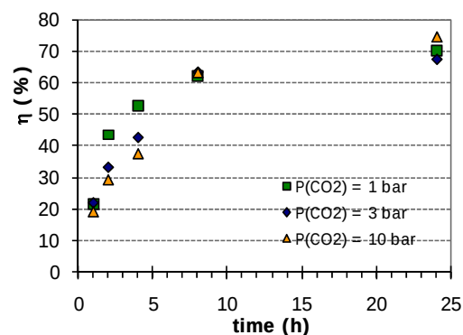
Figura 11: Influenza della pressione di \text{CO}_2 sul rendimento di conversione ottenuto con le ceneri APC
