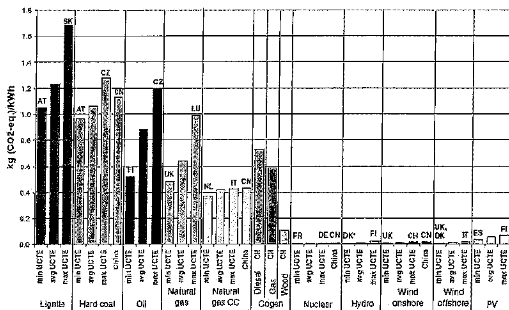
Figura 10: Emissioni di gas serra a seconda della filiera energetica selezionata espresse in \text{kgCO}_2\text{eq/kWh} [17]
