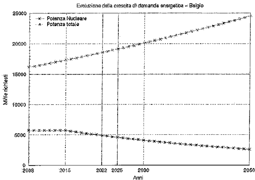
Figura 22: Andamento del totale della potenza installata per produzione elettrica, della potenza nucleare installata e della frazione di nucleare in Belgio fra il 2008 e il 2050 - Scenario LOW
