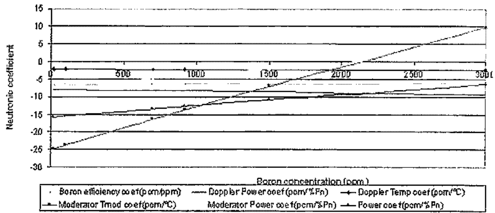
Figura 29 - Core a ciclo unico: coefficienti neutronici a EOI in assenza di Xe
