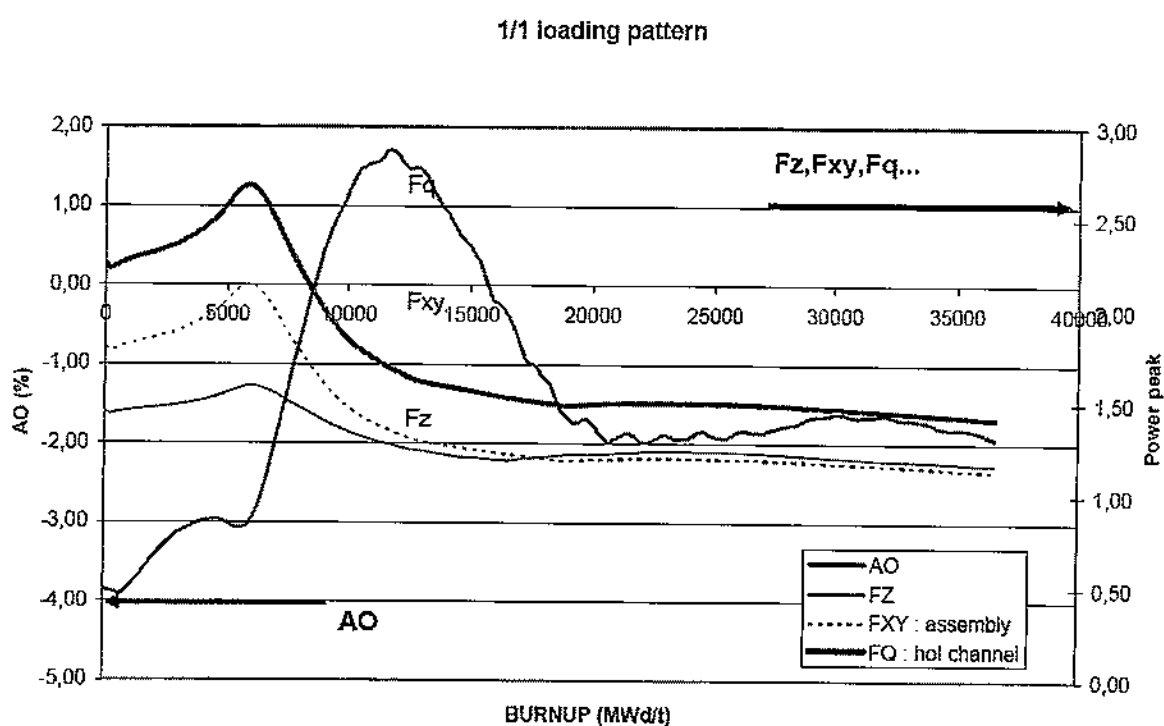
Figura 25 - Core a ciclo unico: F_q , F_{xy} , F_z ed axial offset
