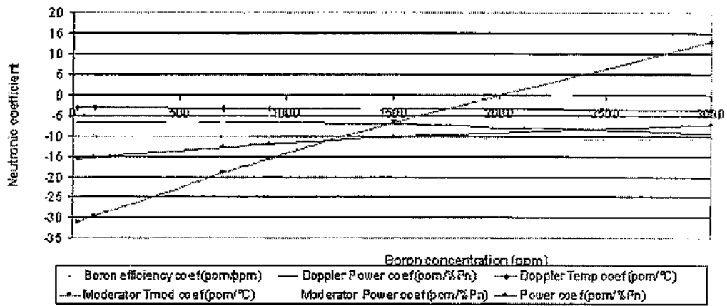
Figura 30 - Core a ciclo unico: coefficienti neutronici a EOI in presenza di Xe
