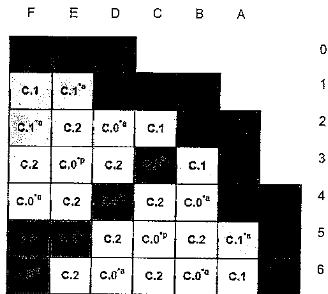
Figura 8 - Core a 4 cicli di ricarica: mappa di caricamento (* RCCA attivi, *p RCCA passivi)
