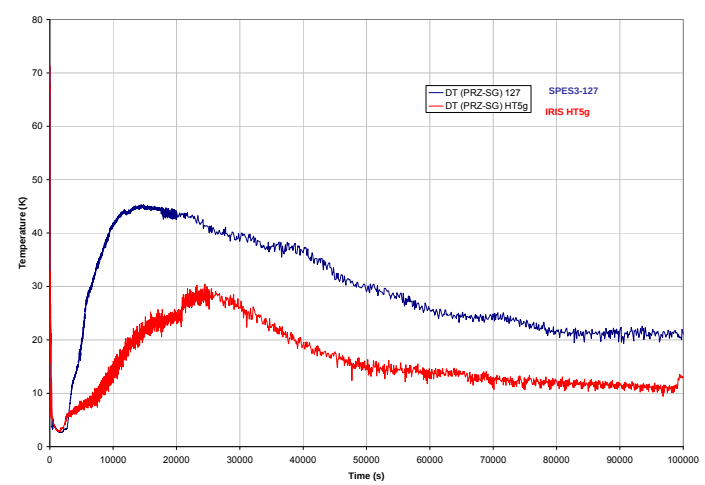
Fig.A10. 2 T (PRZ) – T (SG)
