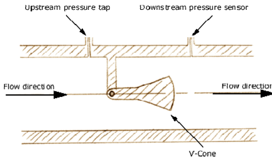
Fig. 37: V-cone flowmeter
