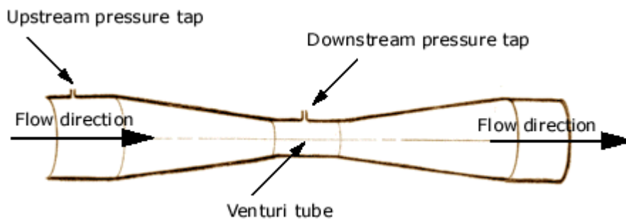
Fig. 32: Venturi tube
