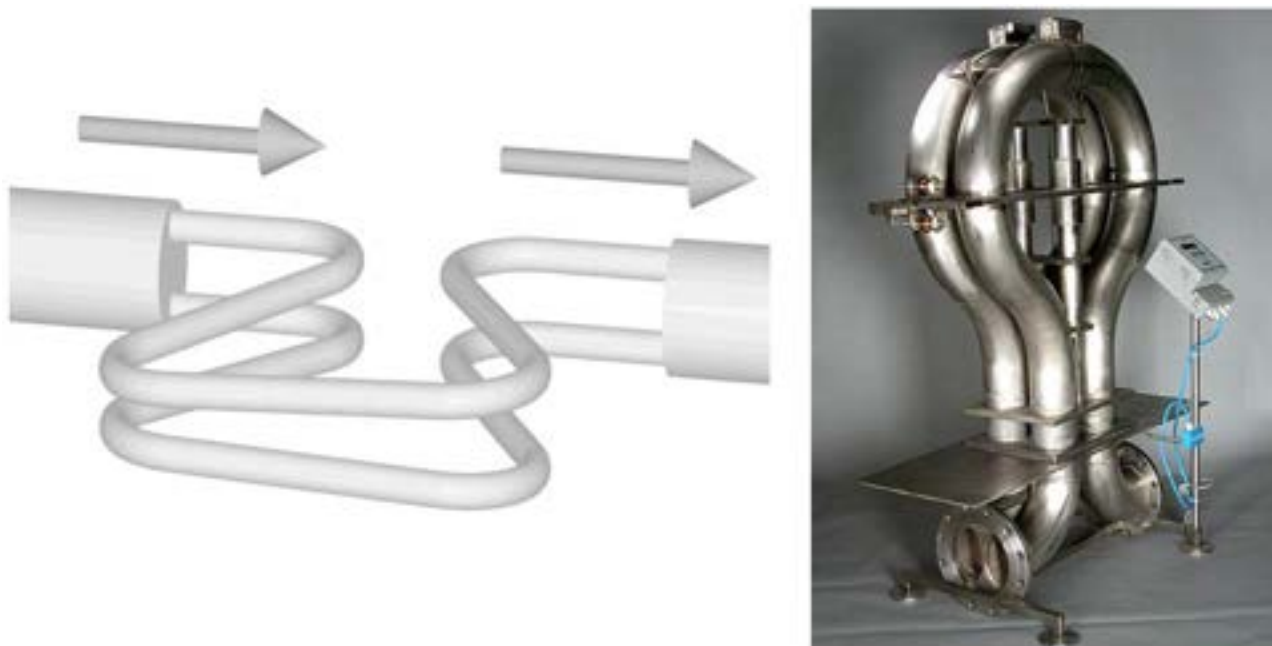
Figura 11: Misuratore di portata ad effetto Coriolis
