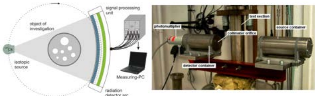
Figura 18: Gammadensitometro e semplice rappresentazione del funzionamento
