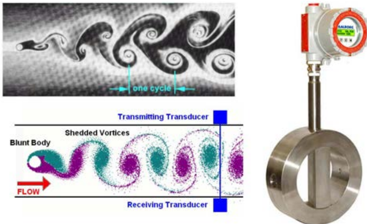
Figura 10: Misuratore di portata a generazione di vortici e funzionamento
