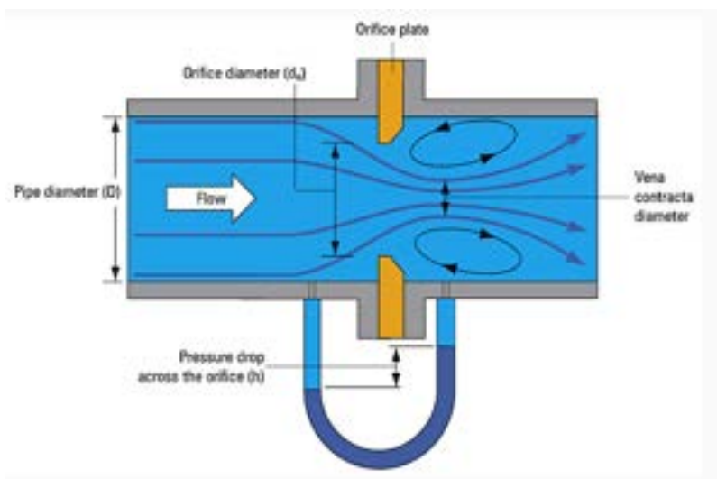
Figura 7: Diaframma con manometro ad U
