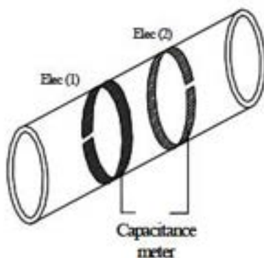
Figura 20: Tipica configurazione della sonda capacitiva integrale ad anelli o capacitive wire
