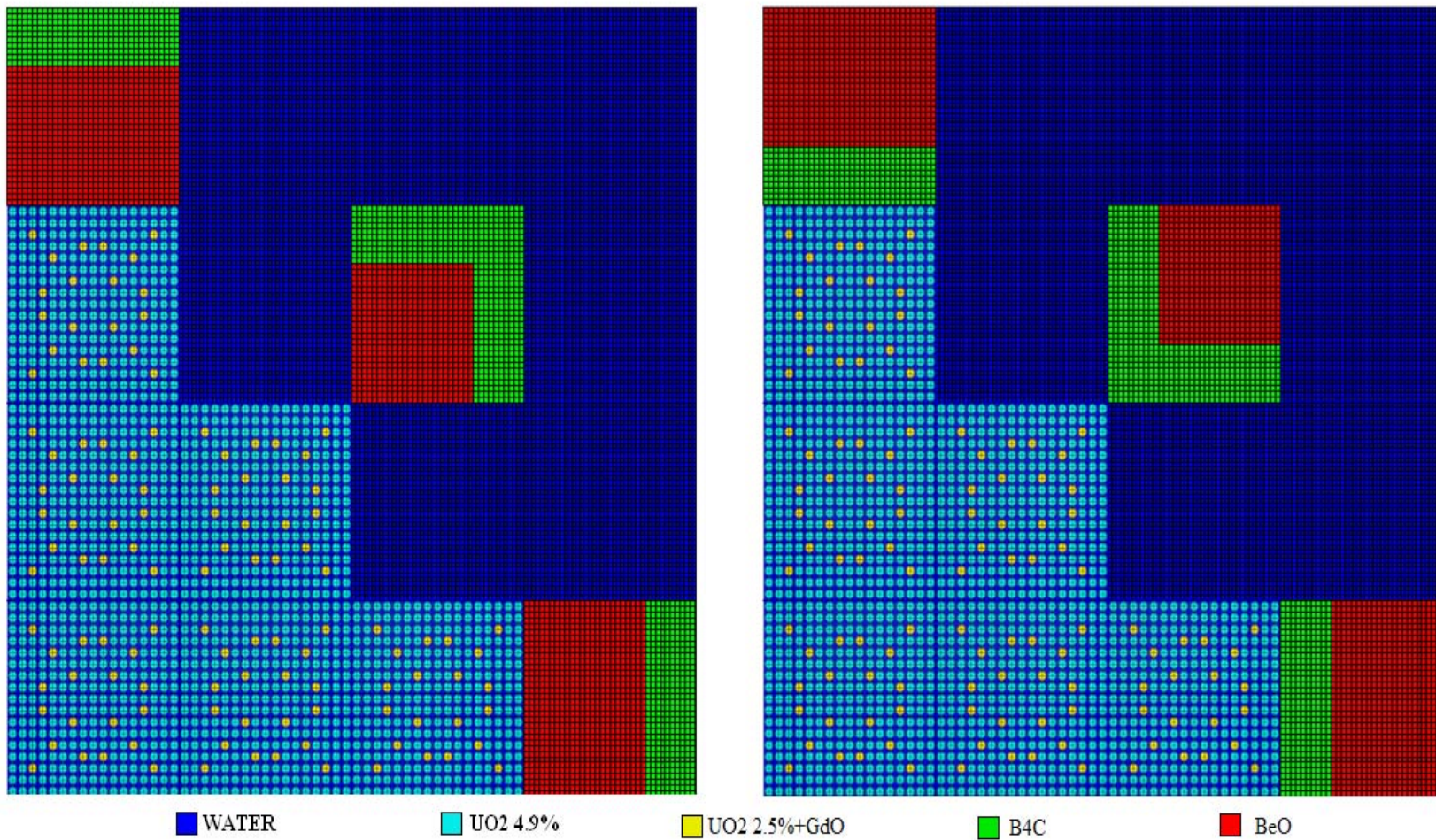
Figura 4.1 – Core “C-1” in funzionamento “normale” (sx) e “controllo” (dx)
