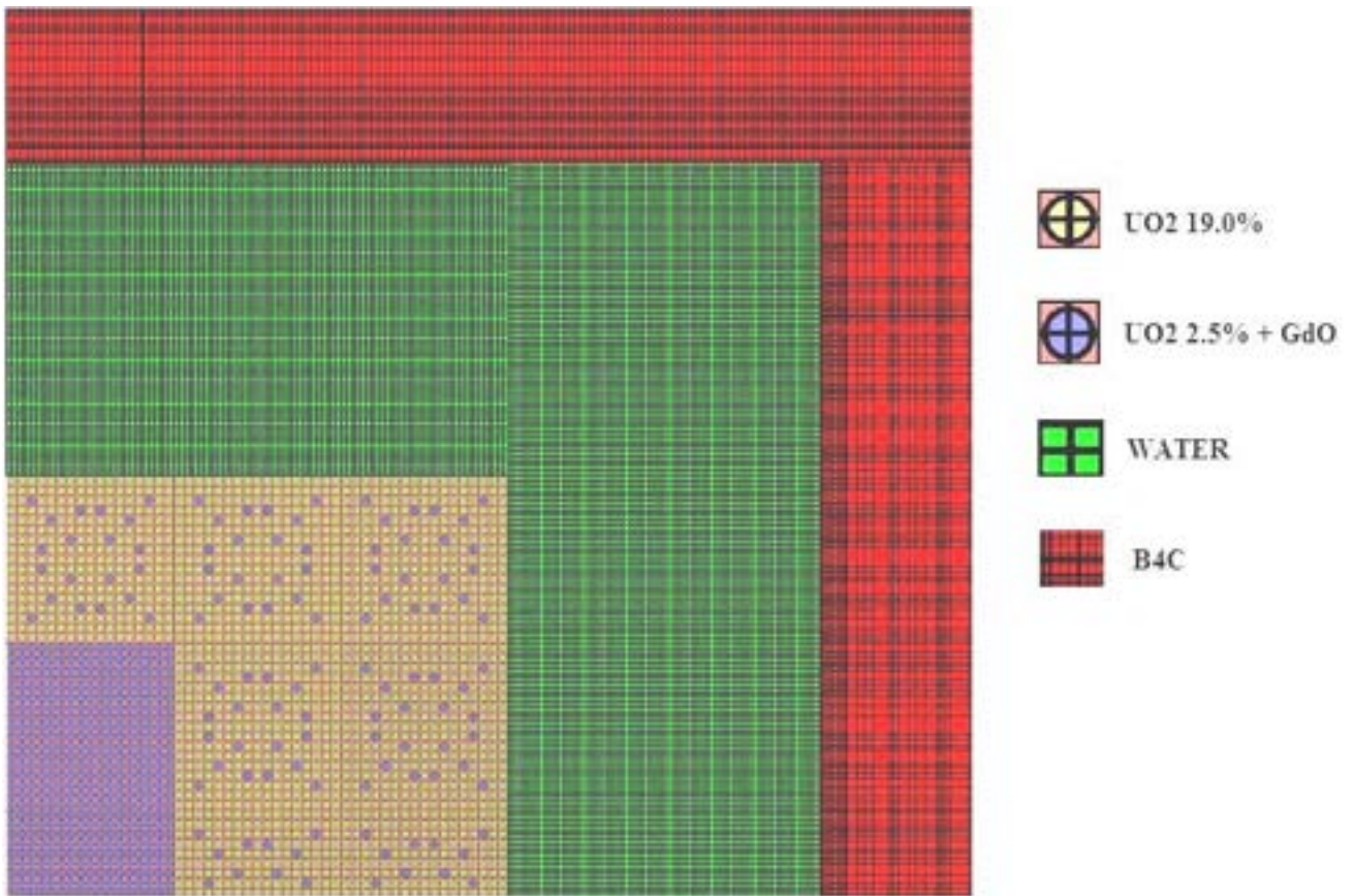
Figura 5.5 – Modello “E-2” nel funzionamento “normale”
