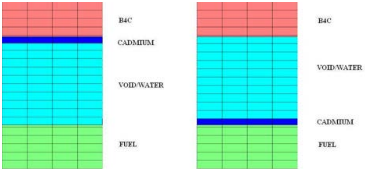
Figura 5.1 – Schematizzazione in NEWT del LINER – A (sx) e LINER – B (dx) con 3 cm di ossido di cadmio
