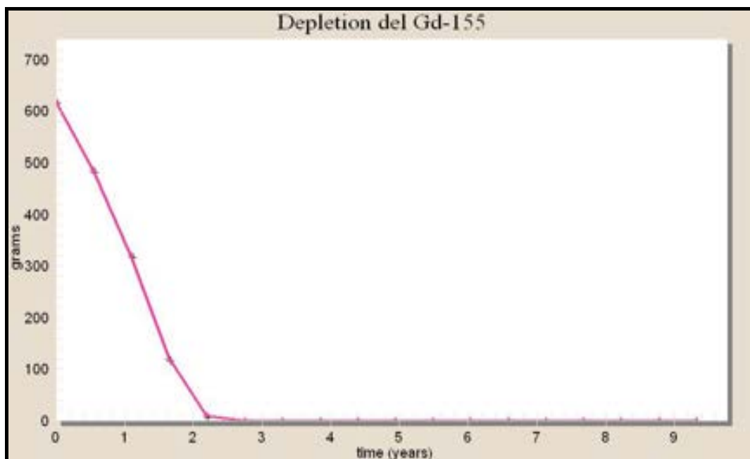
Figura 2.3 – Bruciamento del ^{155}\text{Gd} nelle barrette con veleni bruciabili del fuel assembly “17x17”
