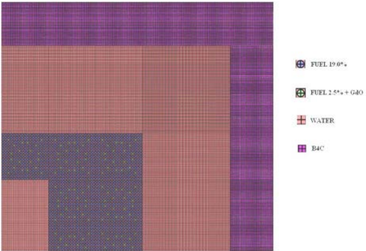
Figura 5.4– Modello “E-1” nel funzionamento “normale”
