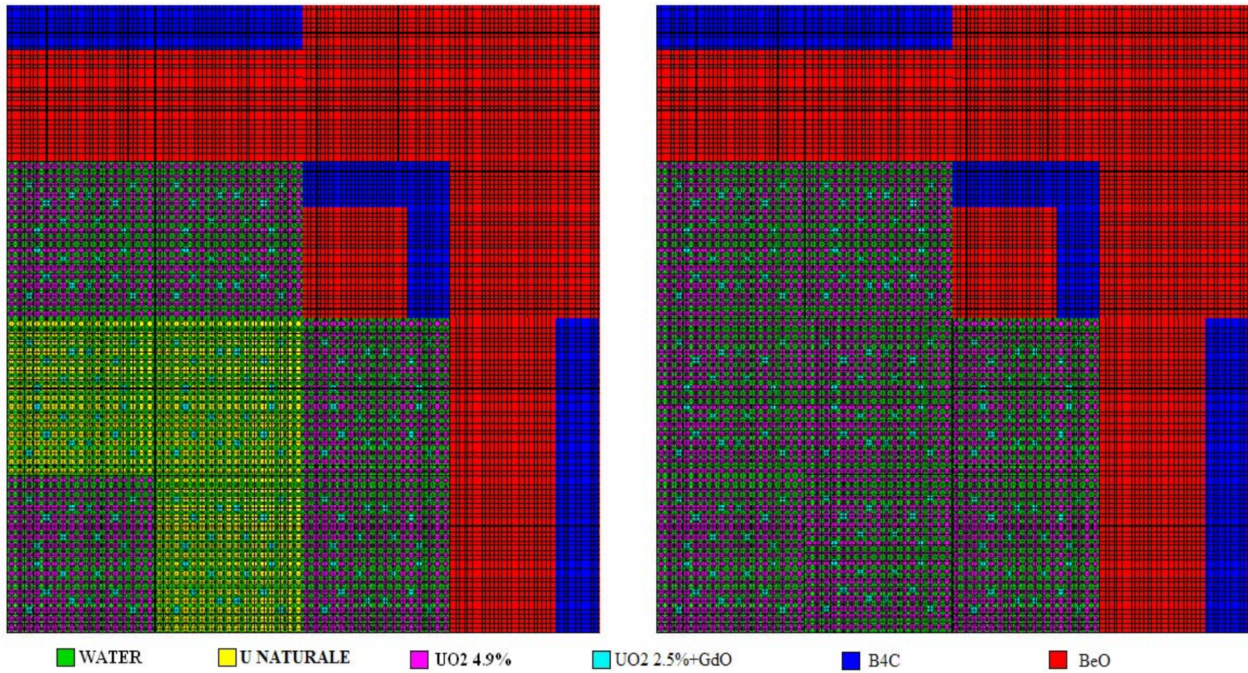
Figura 4.2 – Core “C-3-A” e “C-3-B” nel funzionamento “normale”
