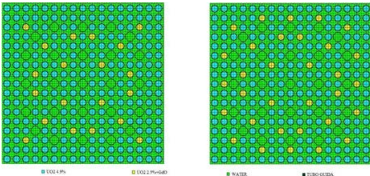
Figura 2.1 – Schematizzazione in NEWT del fuel assembly “17x17” con 20 e 32 Gd 2 O 3 rods
