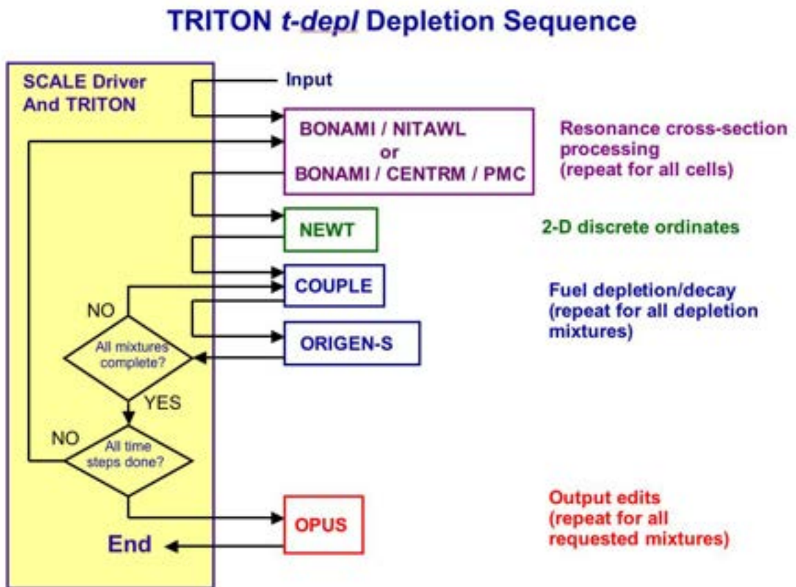
Figura B.1. – Diagramma di flusso della sequenza t-depl per i calcoli di bruciamento
