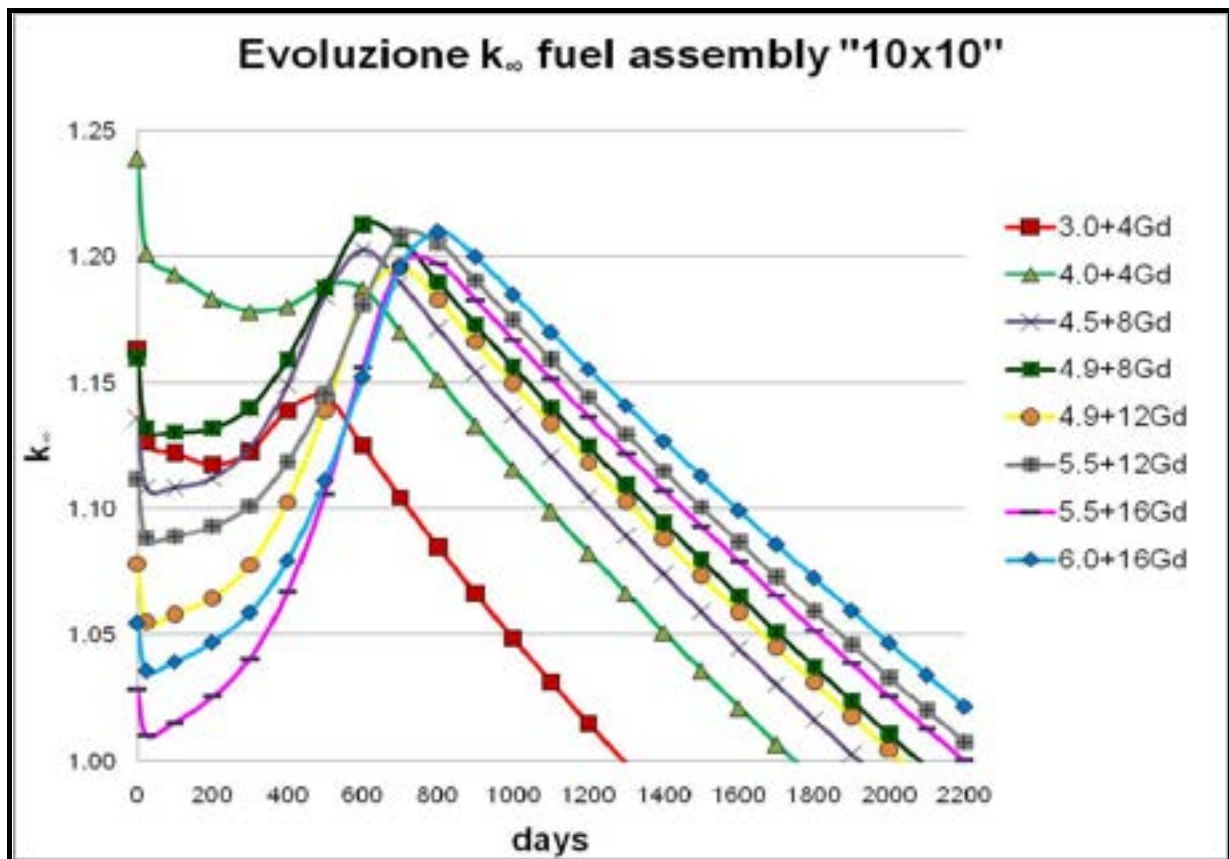
Figura 3.2 – Evoluzione k_{\infty} negli elementi di combustibile “10x10”
