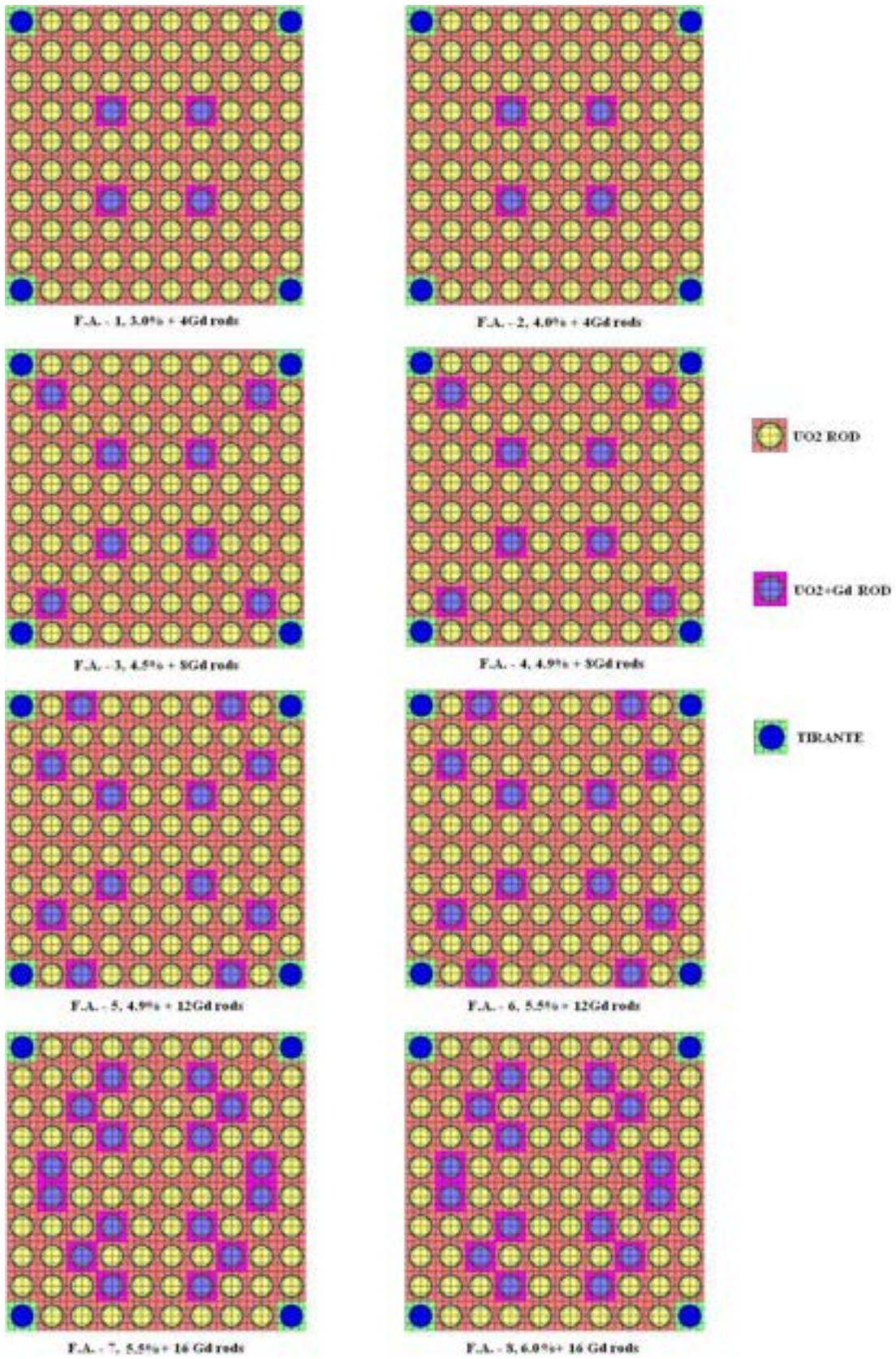
Figura 3.1 – Rappresentazione in NEWT degli elementi di combustibile “10x10”
