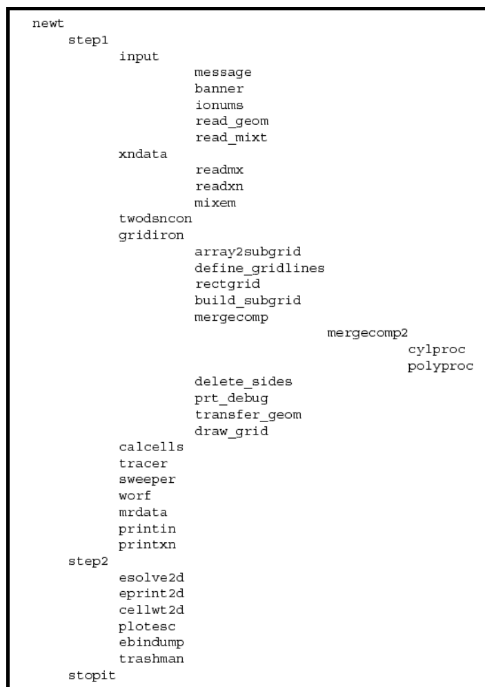
Figura A.1 – Diagramma di flusso delle principali subroutine di NEWT
