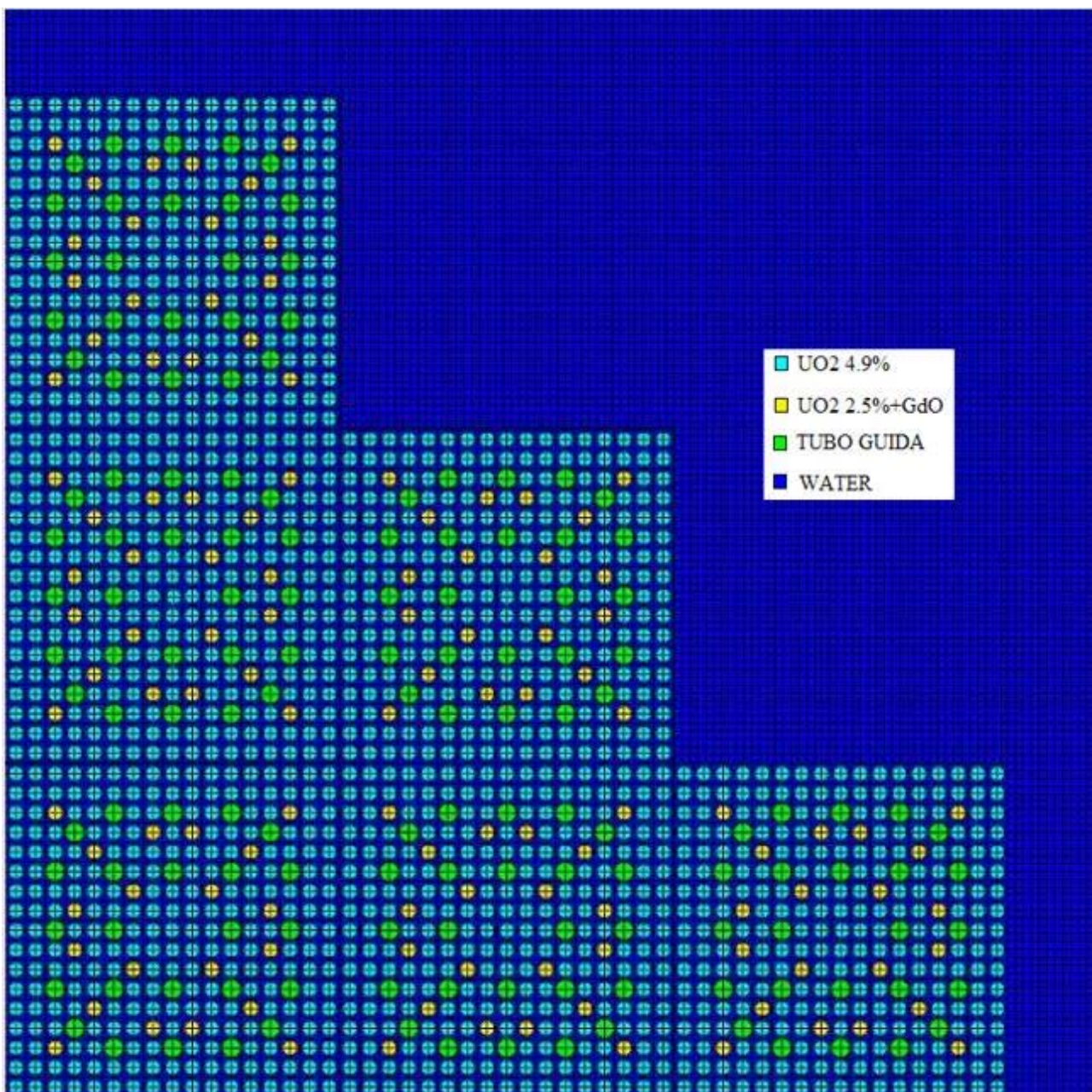
Figura 2.4 – Modello core “A-1” con fuel assembly “17x17” (barre estratte)
