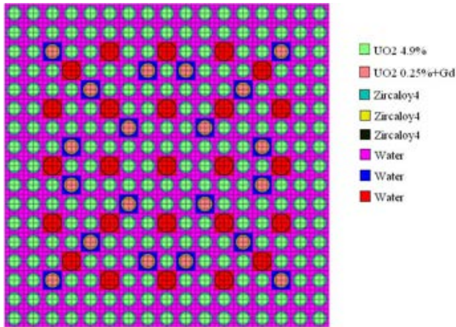
Figura B.2 – Rappresentazione del fuel assembly di riferimento in NEWT
