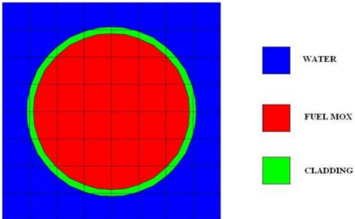
Figura A.2 – Schematizzazione in NEWT della pin di combustibile MOX
