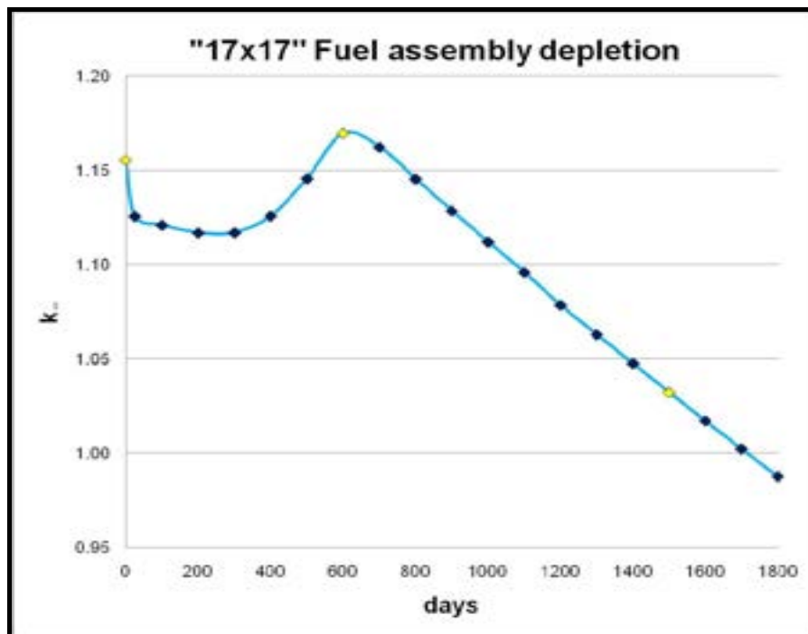
Figura B.3 – Andamento del k_{\infty} nel burn-up del fuel assembly di riferimento
