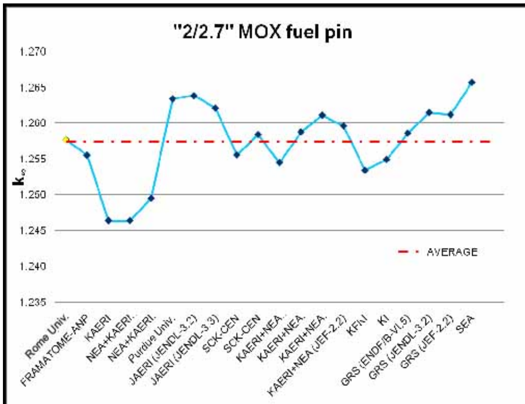
Figura A.5 – Confronto k ∞ pin di combustibile 2/2.7 (MOX)
