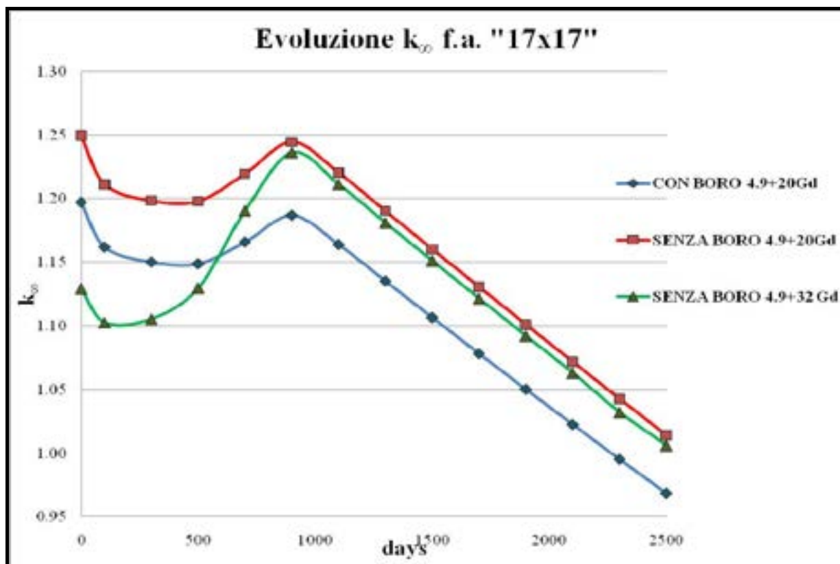
Figura 2.2 – Evoluzione k_{\infty} in un fuel assembly “17x17” con e senza boro disciolto
