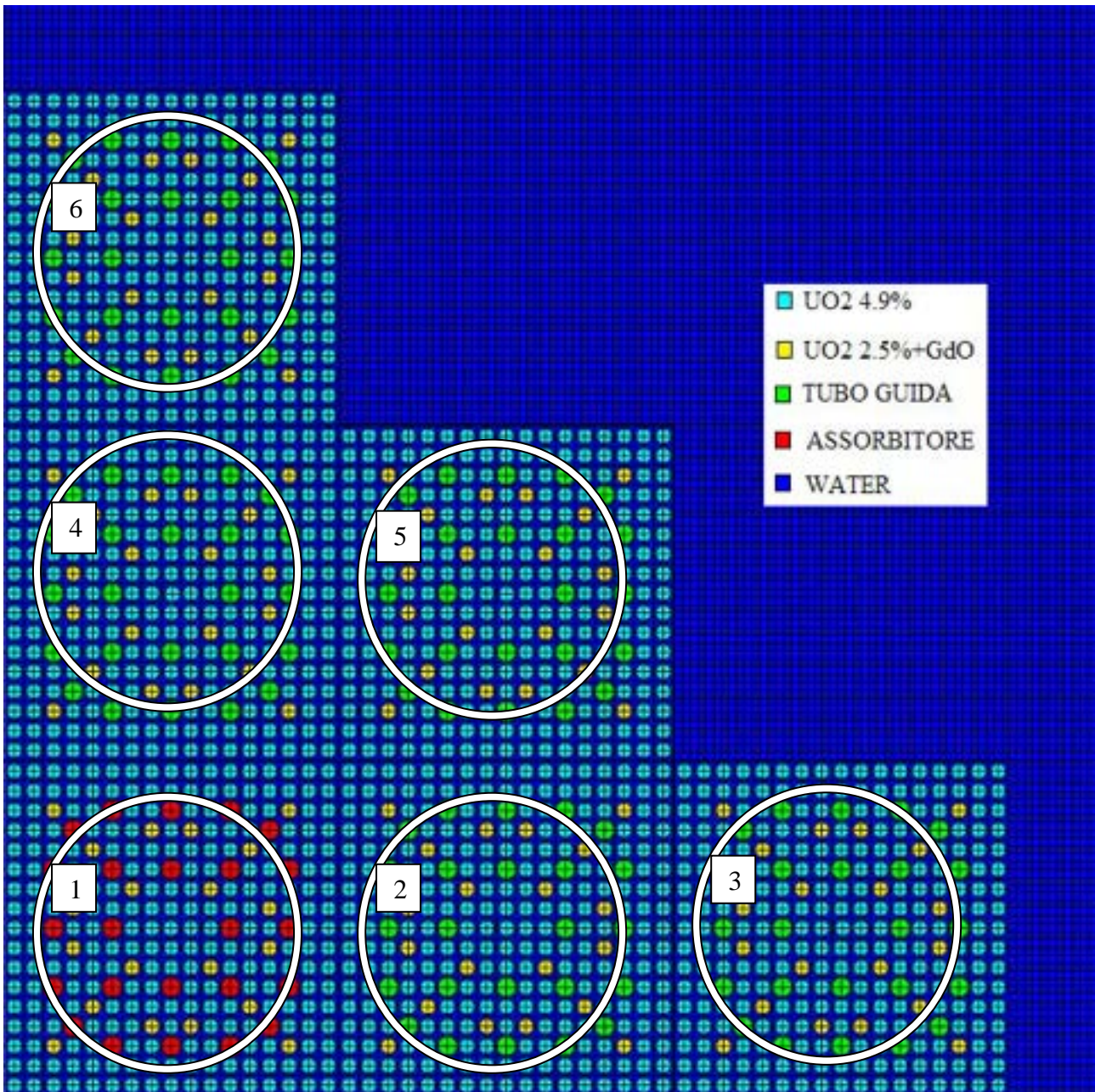
Figura 2.5 – Core “A-1”, numerazione cluster di barre di controllo (gruppo 1 estratto)
