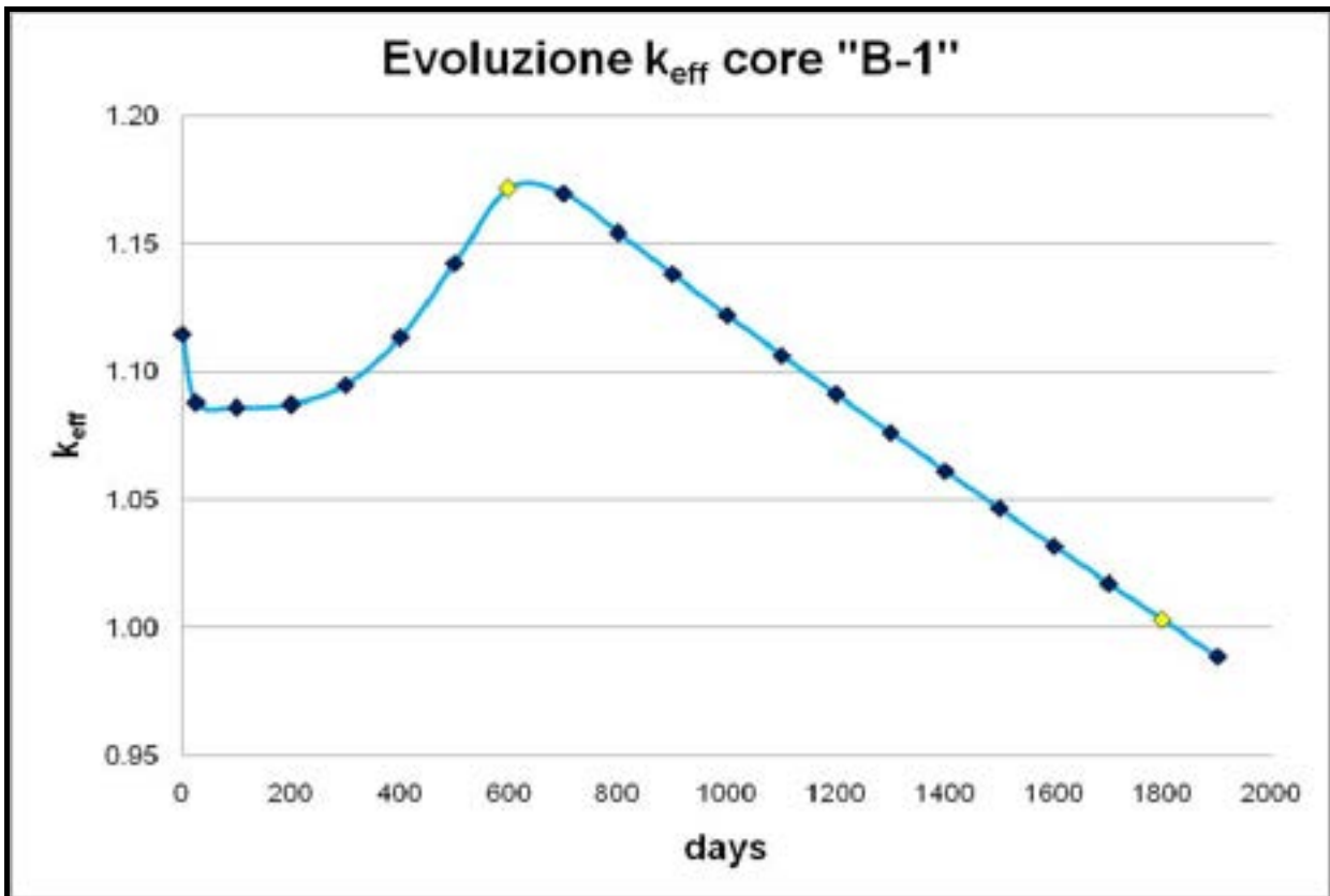
Figura 3.4 – Core “B-1”, evoluzione k_{eff} barre estratte
