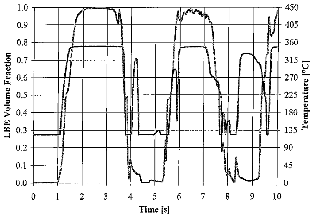
Figura 25. Andamenti della temperatura (linea blu) e della frazione volumetrica di LBE (linea arancione) all'interno della cella (1,35) per una rottura del tubo posta a 3.6 m di profondità
