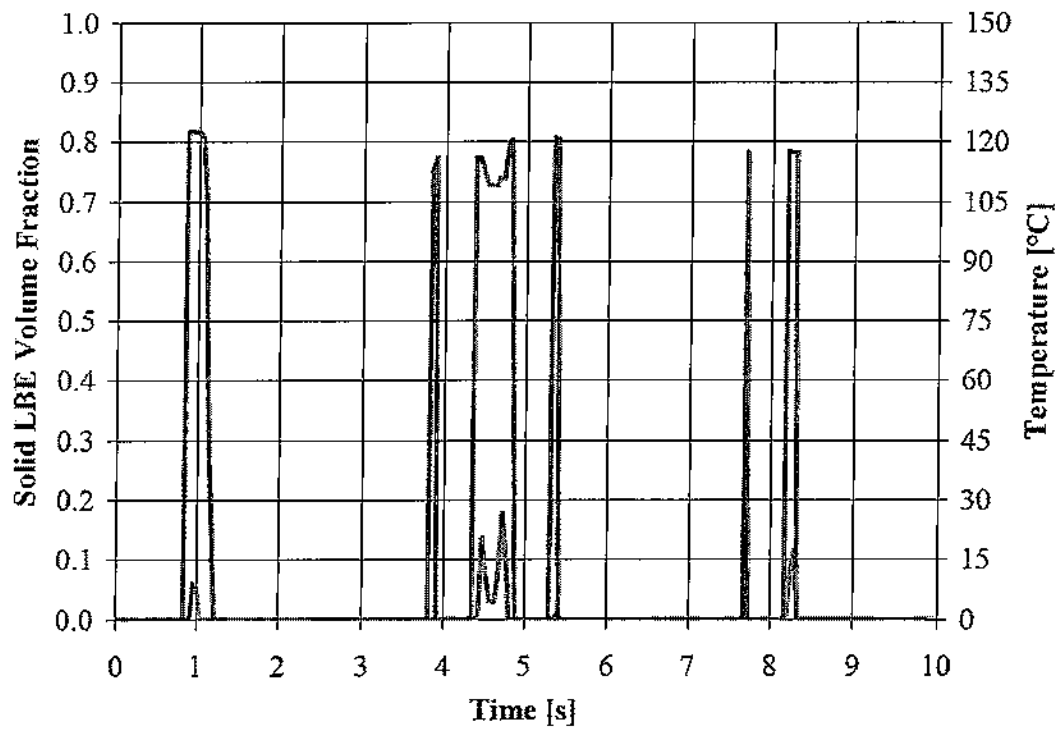
Figura 26. Andamenti della temperatura (linea blu) e della frazione volumetrica di LBE (linea arancione) all'interno della cella (1,35) per una rottura del tubo posta a 3.6 m di profondità
