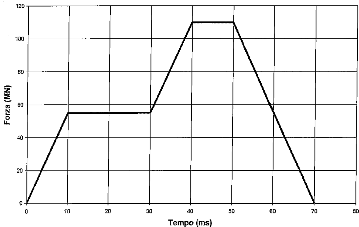
Figura 1.3 Diagramma di carico associato ad impatto aereo
