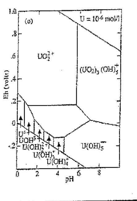
Fig. 5 : Diagramme Eh-pH illustrant l'importance relative des valances +4, +5 ( UO_2^{2+} ) et +6 de l'uranium à 25°C. ( \Sigma U = 10^{-6} M ) (d'après Langmuir, 1978)
