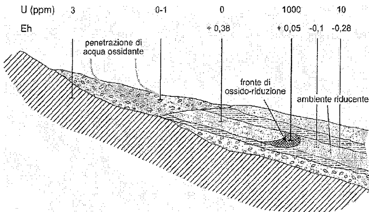
Figura 2.1 – La formazione dei giacimenti uraniferi come dimostrazione dell'efficacia della barriera geochemica esercitata dal carattere riducente di massa delle argille (Brondi A., Brondi F., 1999).
