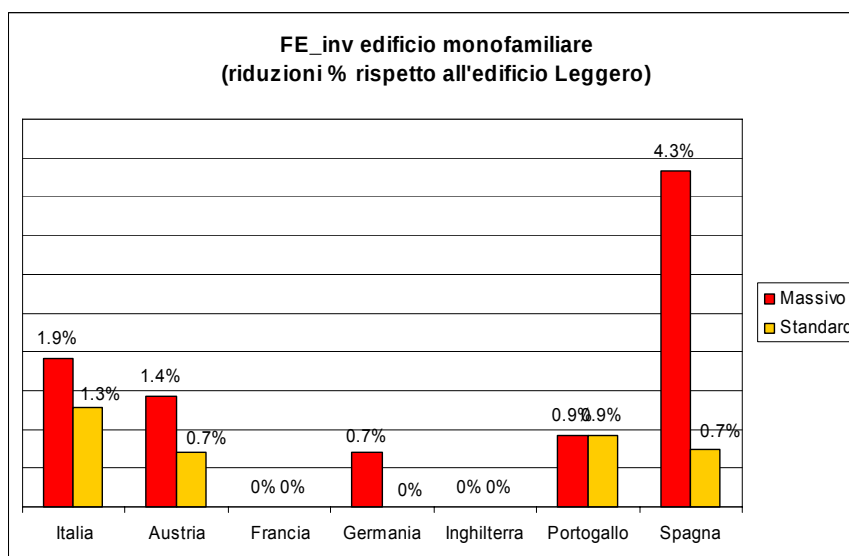
Grafico2: Confronto tra i risultati relativi al fabbisogno energetico per riscaldamento invernale (edificio monofamiliare)
