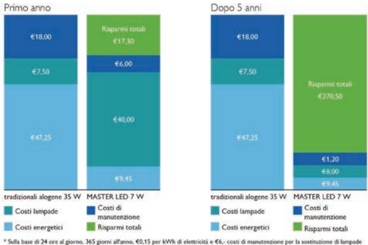
Fig. 14 - Risparmio ottenibile dalla sostituzione di una lampada ad alogeni 35W con una Philips MasterLED 7W.
