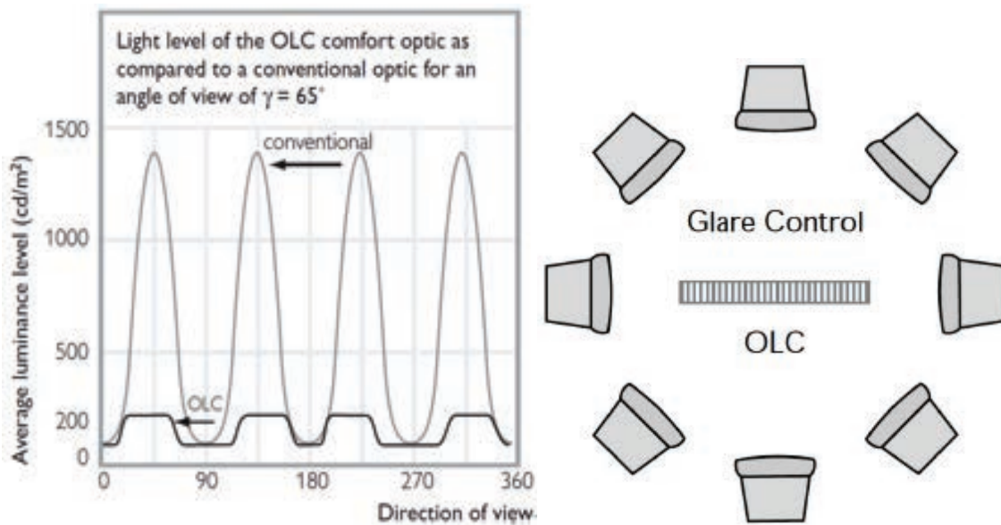
Fig. 21- Confronto tra la luminanza a 65^\circ di un apparecchio convenzionale e quella di un'ottica OLC in relazione alla direzione di osservazione
