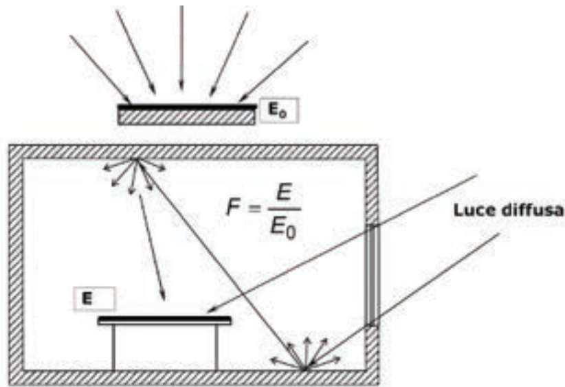
Fig. 6 - Schema del fattore di luce diurna
