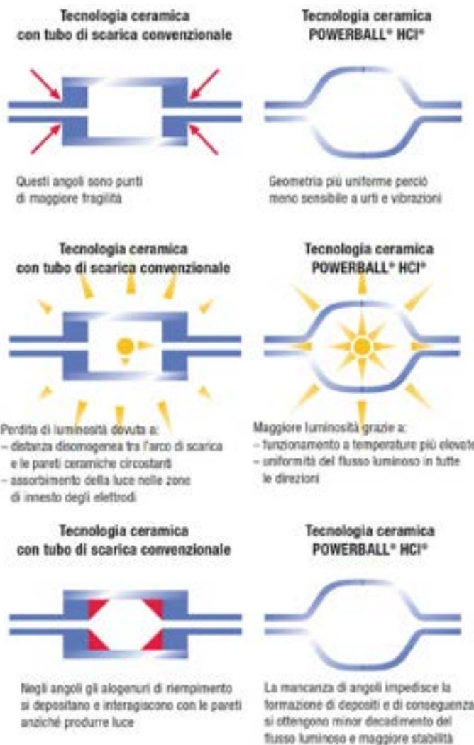
Fig. 49 - Confronto tra le prestazioni di un bruciatore cilindrico e quello della sorgente Powerball di Osram, di forma sferica.
