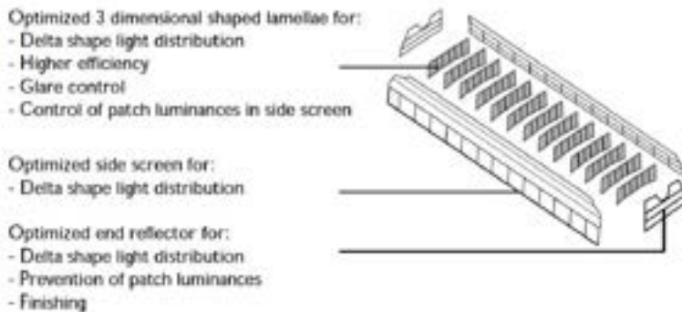
Fig. 75 - Parti che compongono un riflettore OLC
