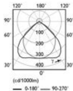
Fig. 76 - Curva fotometrica tipo BAP di un'ottica OLC
