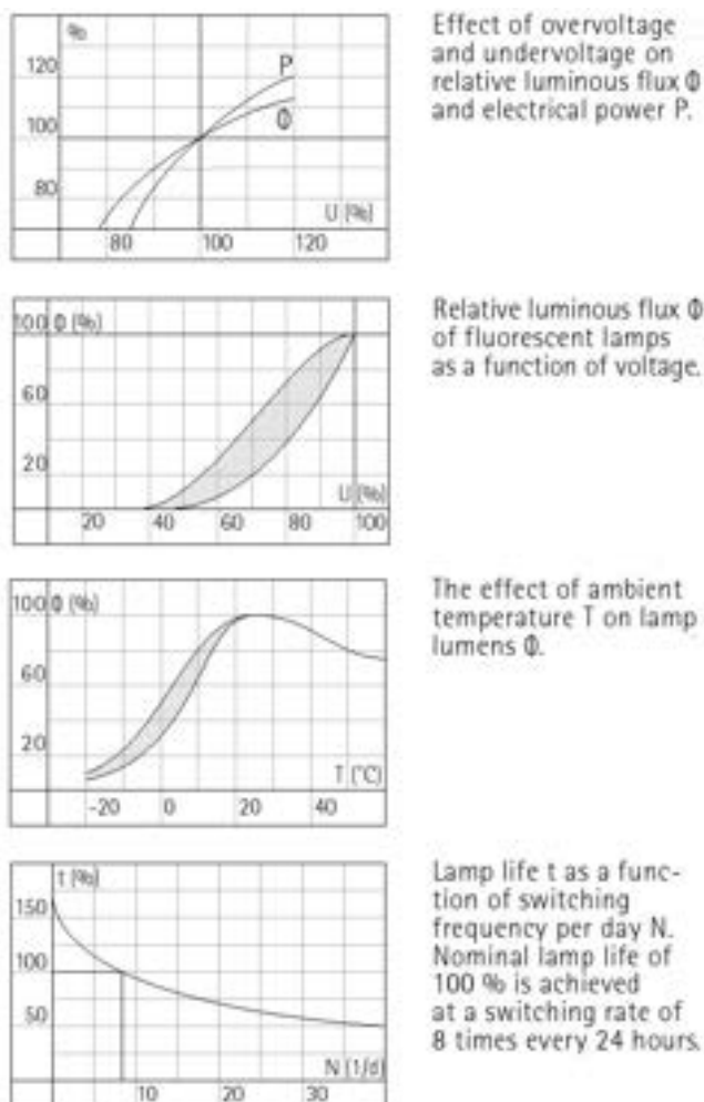
Fig. 44 - Variazioni del flusso luminoso e della durata di una lampada fluorescente al variare di alcuni parametri.
