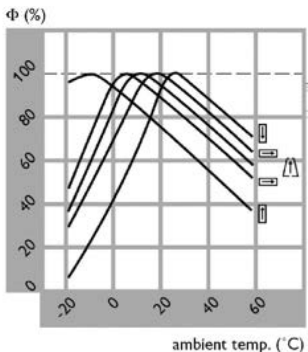
Fig. 46 - Relazione tra flusso luminoso di una sorgente fluorescente, temperatura ambiente e posizione di funzionamento.
