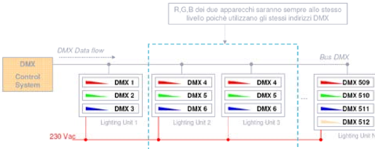
Figura 31 - Modalità di funzionamento del protocollo DMX (fonte: PHILIPS)
