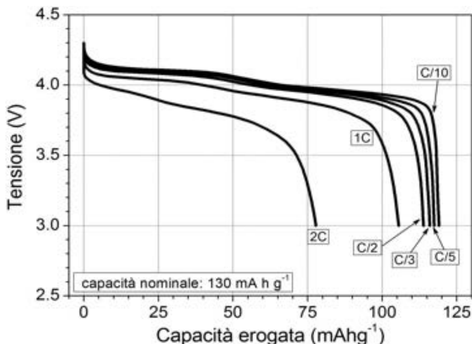
Figura 17. Profilo tensione-capacità, relativo a semi-cicli di scarica eseguiti a differenti valori di corrente, per i nastri catodici LiMn 2 O 4 . T = 20°C
