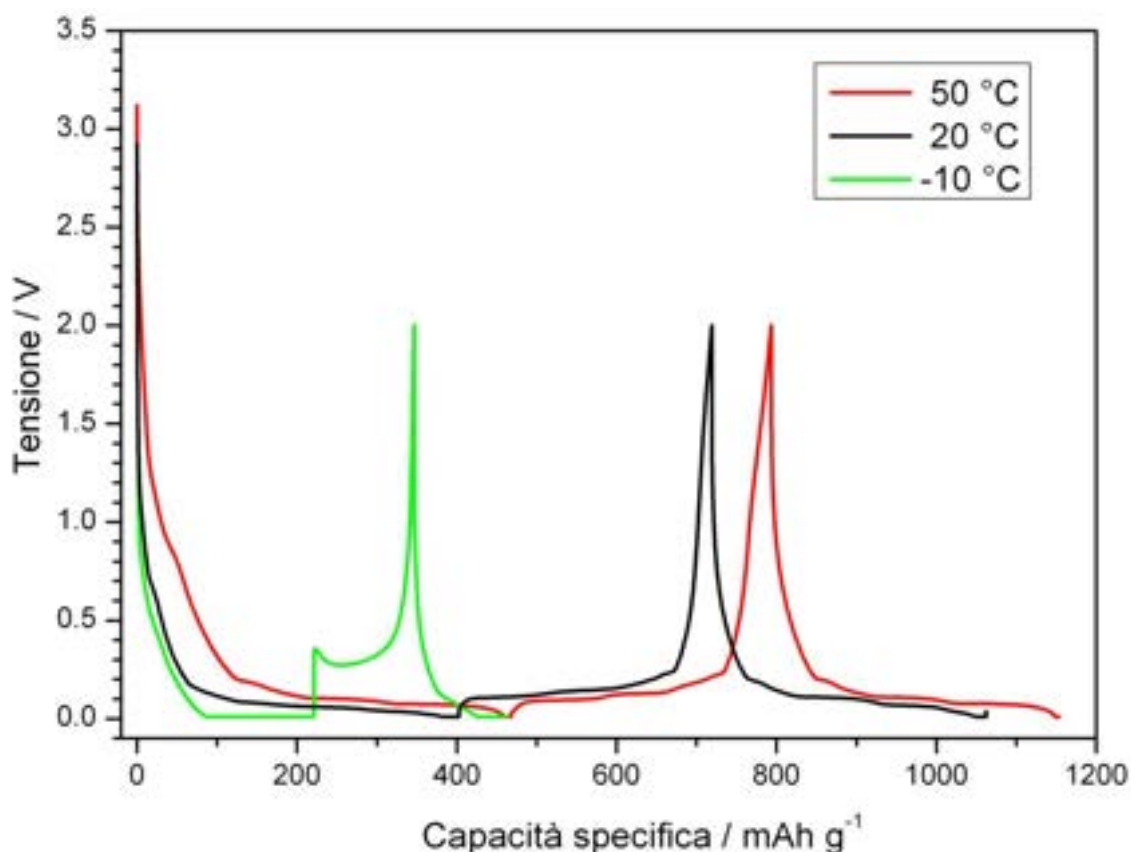
Figura 21. Profilo tensione-capacità specifica, relativo al 1° ciclo di scarica/carica ed il successivo semiciclo di scarica, per semicelle anodiche Li/LiPF 6 -EC-DMC/Anodo C-17-3 a differenti temperature di esercizio ( -10^{\circ}\text{C} , 20^{\circ}\text{C} , 50^{\circ}\text{C} ). j = 0.3\text{ mA cm}^{-2} (C/10).
