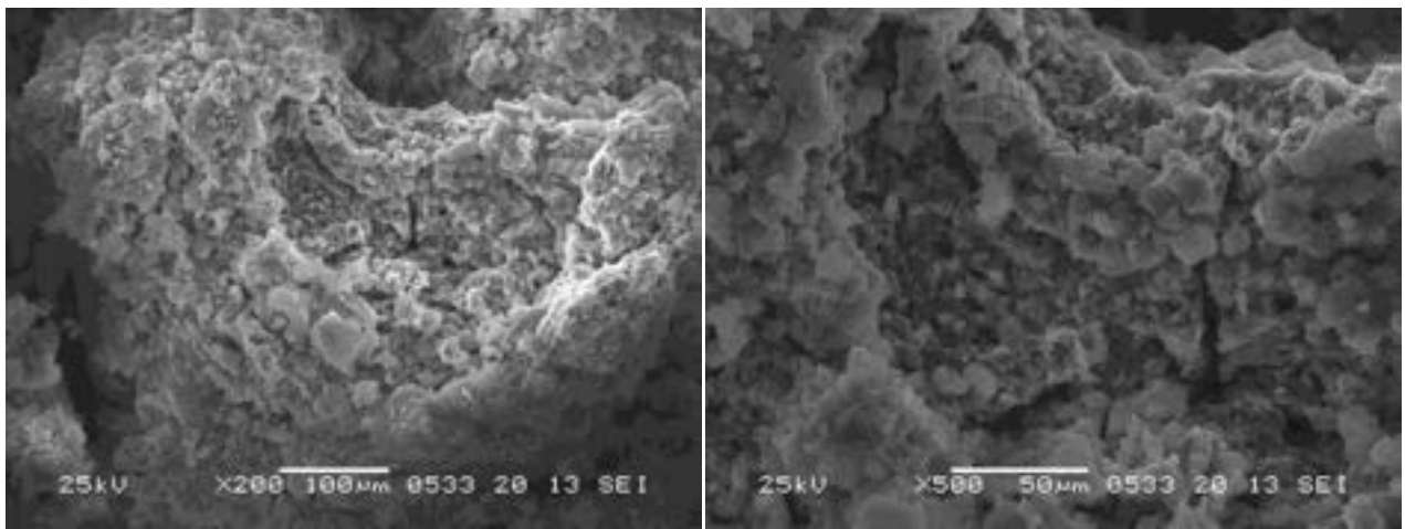
Figura 10. Microfotografie a due maggiori ingrandimenti effettuate sul campione preparato per precipitazione in fase eterogenea da fosfato ammonico stechiometrico sull'aggregato di secondo tipo.
