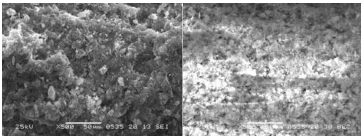
Figura 2. Microfotografie a 500 ingrandimenti effettuate sul campione preparato per precipitazione in fase omogenea in esposizione normale (sinistra) ed in back scattering (destra).
