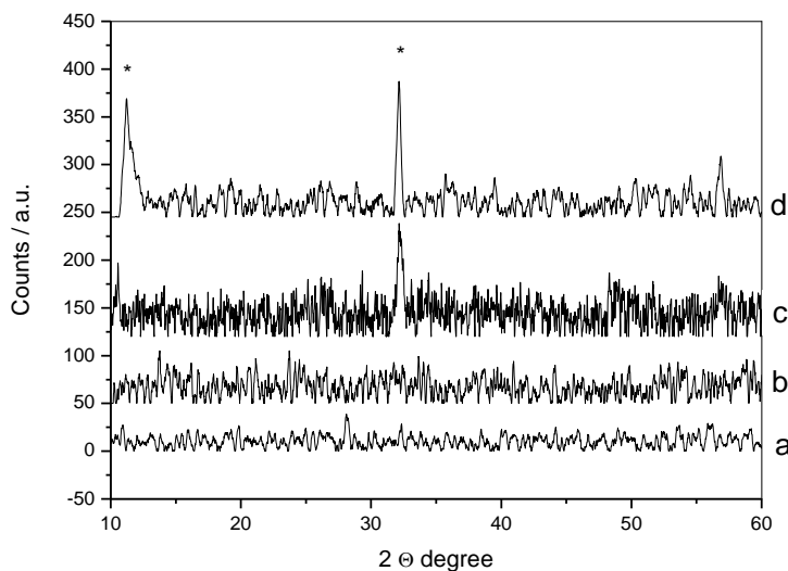
Figura 24. Spettri di diffrazione dei materiali sintetizzati: a) precipitazione in fase omogenea, b) precipitazione in fase eterogenea da fosfato ammonico stechiometrico, c) precipitazione in fase eterogenea da fosfato sodico stechiometrico, d) precipitazione in fase eterogenea da fosfato ammonico sopra stechiometrico.
