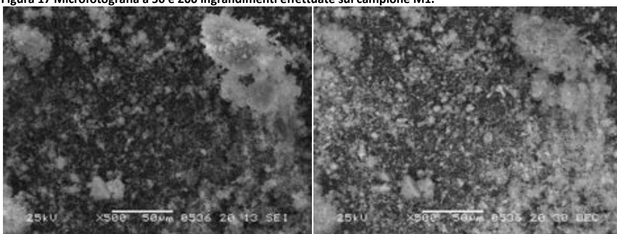
Figura 18. Microfotografie a 500 ingrandimenti effettuate sul campione M1. La foto in basso a destra è l'immagine in back scattering di quella in basso a sinistra.
