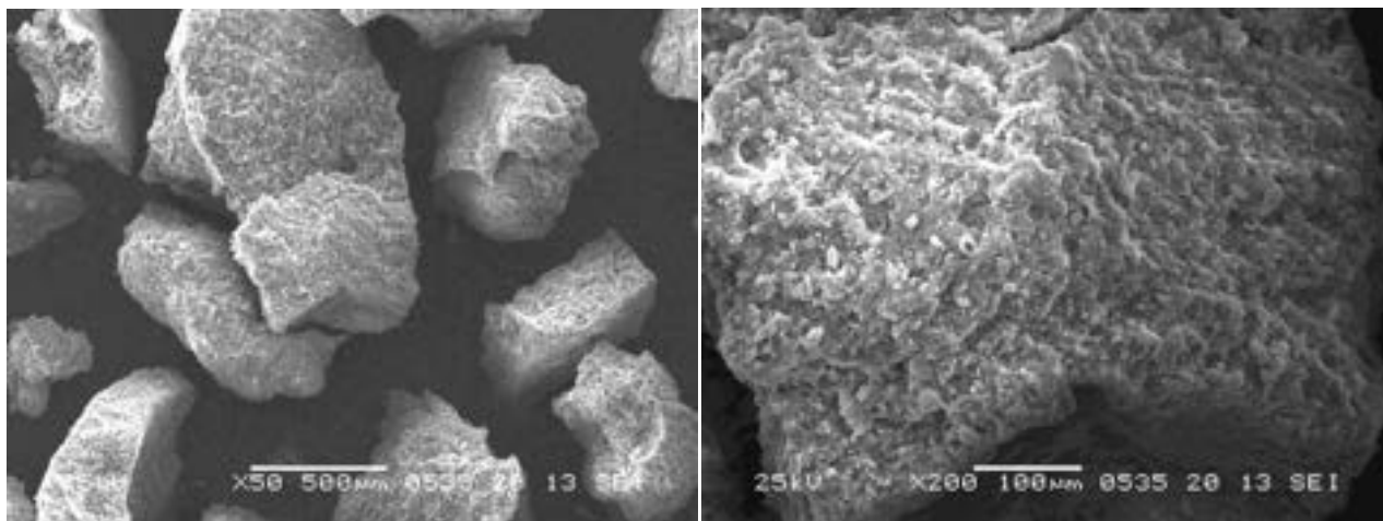
Figura 1. Microfotografie a due differenti ingrandimenti effettuate sul campione preparato per precipitazione in fase omogenea.
