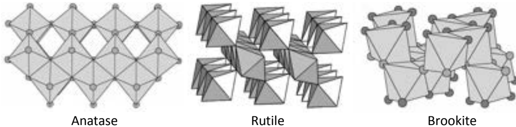
Figura 2. Struttura cristallina delle forme principali di TiO_2 .
