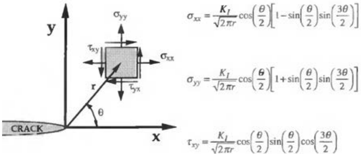
Fig. 1 – apice di un difetto in un materiale elastico-lineare
