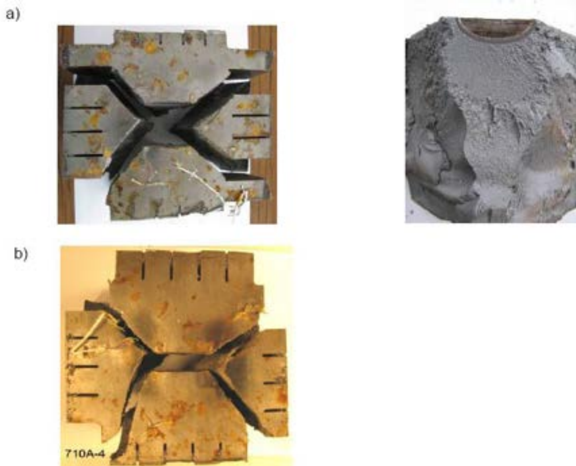
Fig. 18 – Superfici di frattura dei provini
