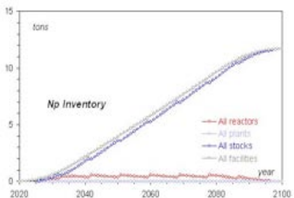
Figura 17: Np accumulato.
