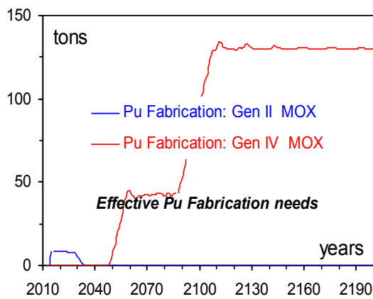
Figura 25: Fabbricazione Pu/Tipo-Reattore; Caso 1.
