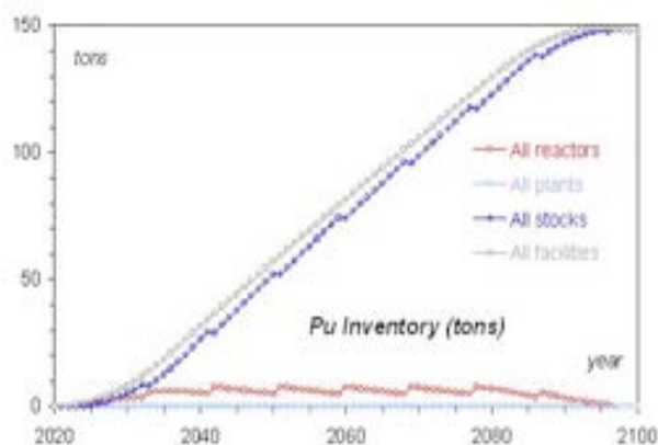
Figura 16: Pu accumulato.
