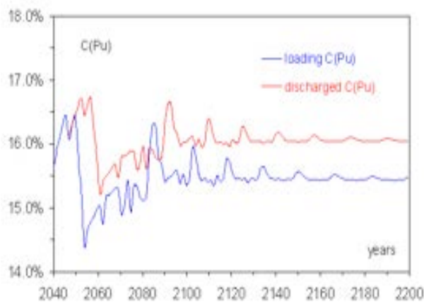
Figura 21: Contenuto in Pu: Pu/(Pu + U); Caso 1.
