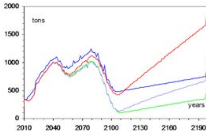
Figura 20: Margine di Pu per lo spegamento dei reattori veloci (FR) e sostenibilità dello scenario energetico. Caso 1 Break-even core, no MA recycling, 5y cooling time; Caso 2 Break-even core, MA recycling, 5y cooling time; Caso 3 Break-even core, no MA recycling, 2y cooling time; Caso 4 Breeder core, no MA recycling, 5y cooling time.
