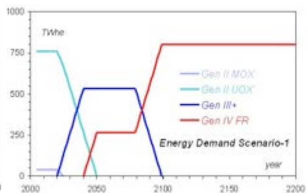
Figura 19 Energia prodotta.
