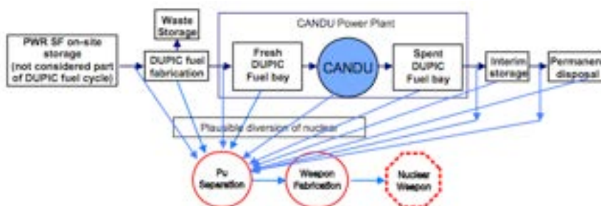
Figura 7: Flusso di materiale nel ciclo DUPIC e possibili punti di accesso al materiale
