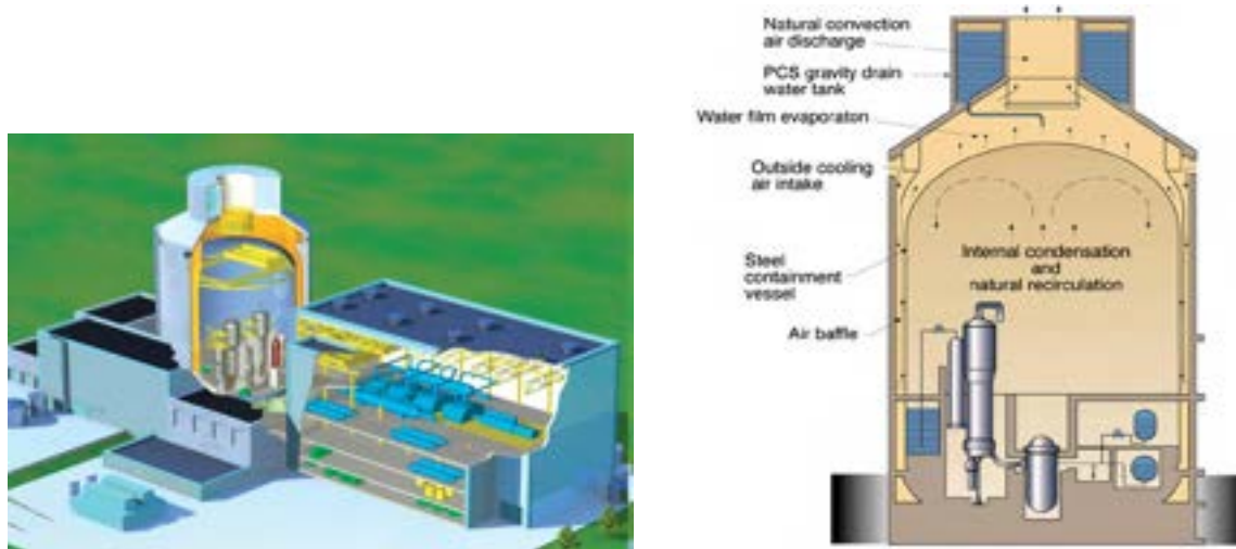
Fig. 4.5 - Reattore AP-1000
