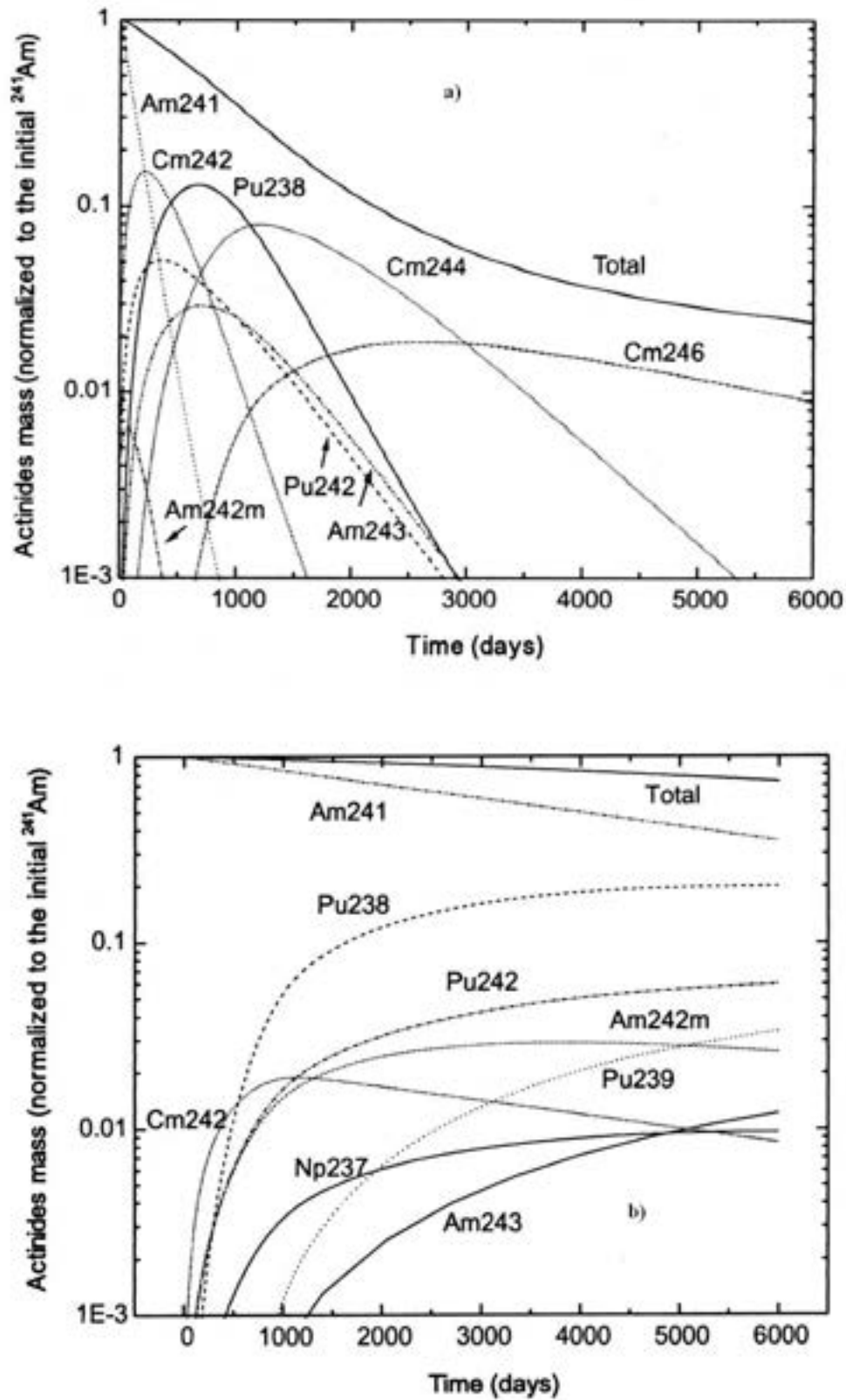
Figura 1: Evoluzione isotopica in un campione di ^{241}\text{Am} irraggiato in uno spettro termico (a) ed in uno spettro veloce (b) con flusso costante di 10^{15} \text{ n cm}^{-2} \text{ s}^{-1} [5].
