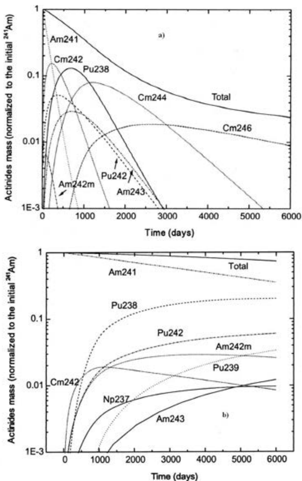
Figura 1: Evoluzione isotopica in un campione di 241 Am irraggiato in uno spettro termico (a) ed in uno spettro veloce (b) con flusso costante di 10^{15} \text{ n cm}^{-2} \text{ s}^{-1} [5].
