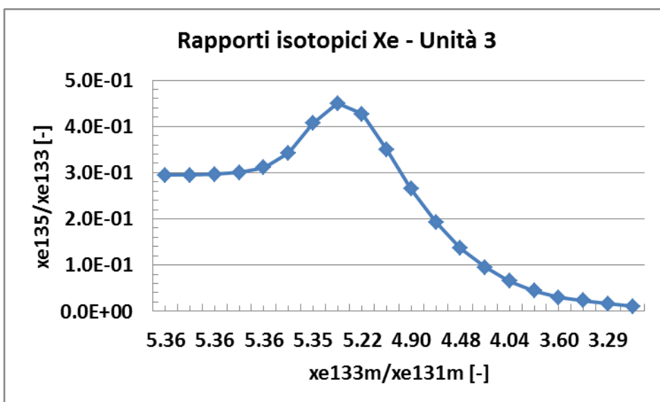
Figura 12: Rapporti isotopici per Unità 3.
