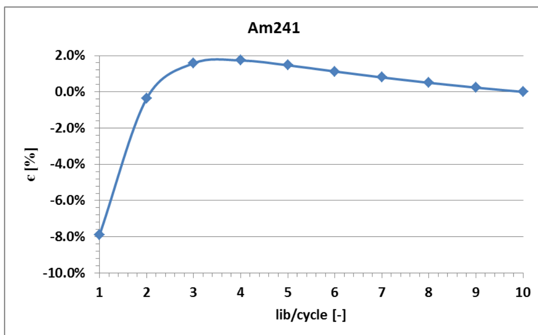
Figura 21: Errore relativo al variare del numero di librerie per ciclo per ^{241}\text{Am} .
