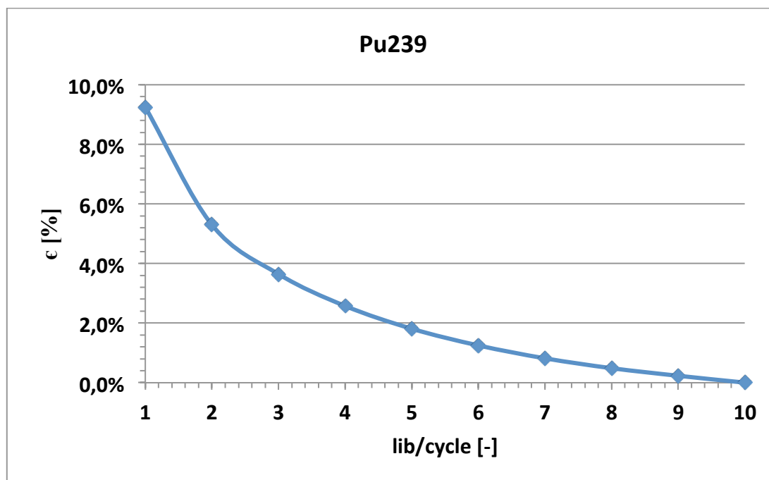
Figura 19: Errore relativo al variare del numero di librerie per ciclo per 239Pu.
