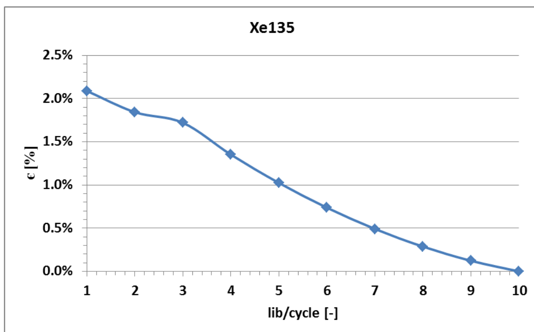
Figura 20: Errore relativo al variare del numero di librerie per ciclo per ^{135}\text{Xe} .
