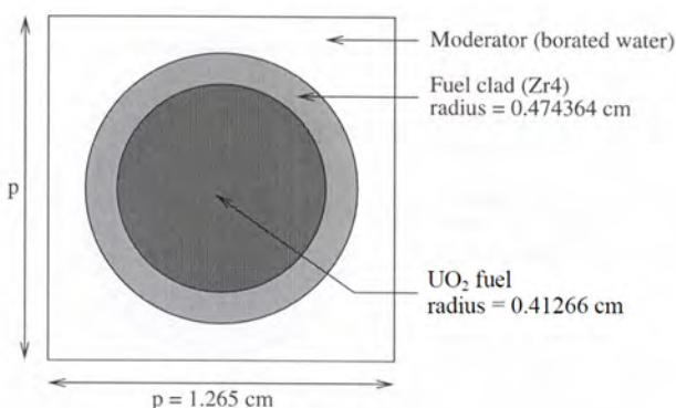
Figura 14: Cella elementare di fuel dell'assembly 17x17.
