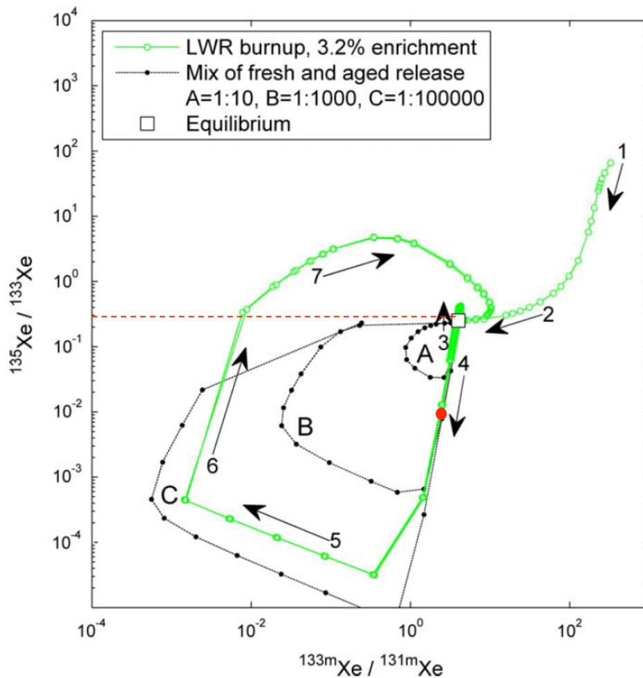
Figura 6: Rapporti isotopici dello Xeno per un LWR (curva verde) [11].
