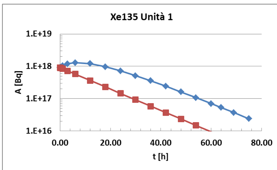
Figura 8: Andamento temporale Xe135 Unità 1 (linea blu).
